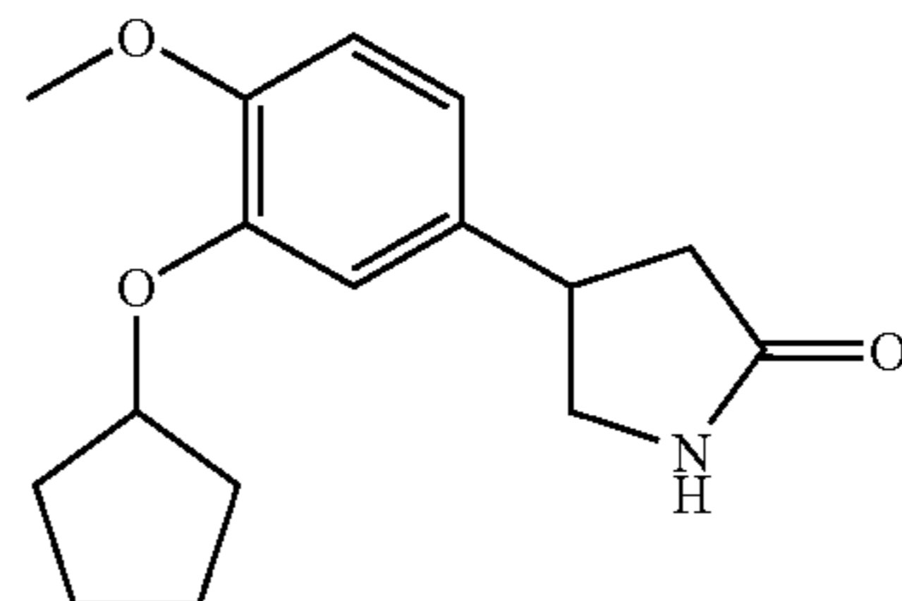
rolipram
