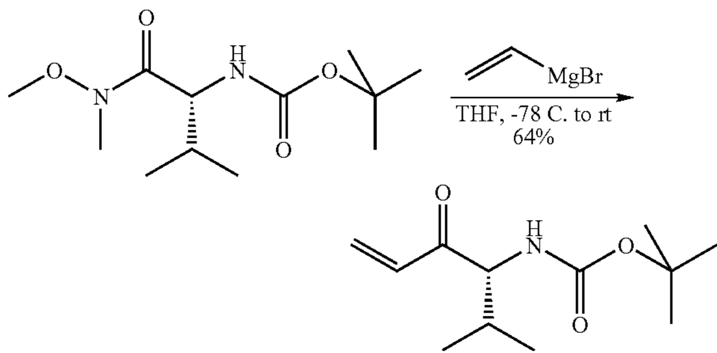
((R)-1-Isopropyl-2-oxo-but-3-enyl)-carbamic acid tert-butyl ester
