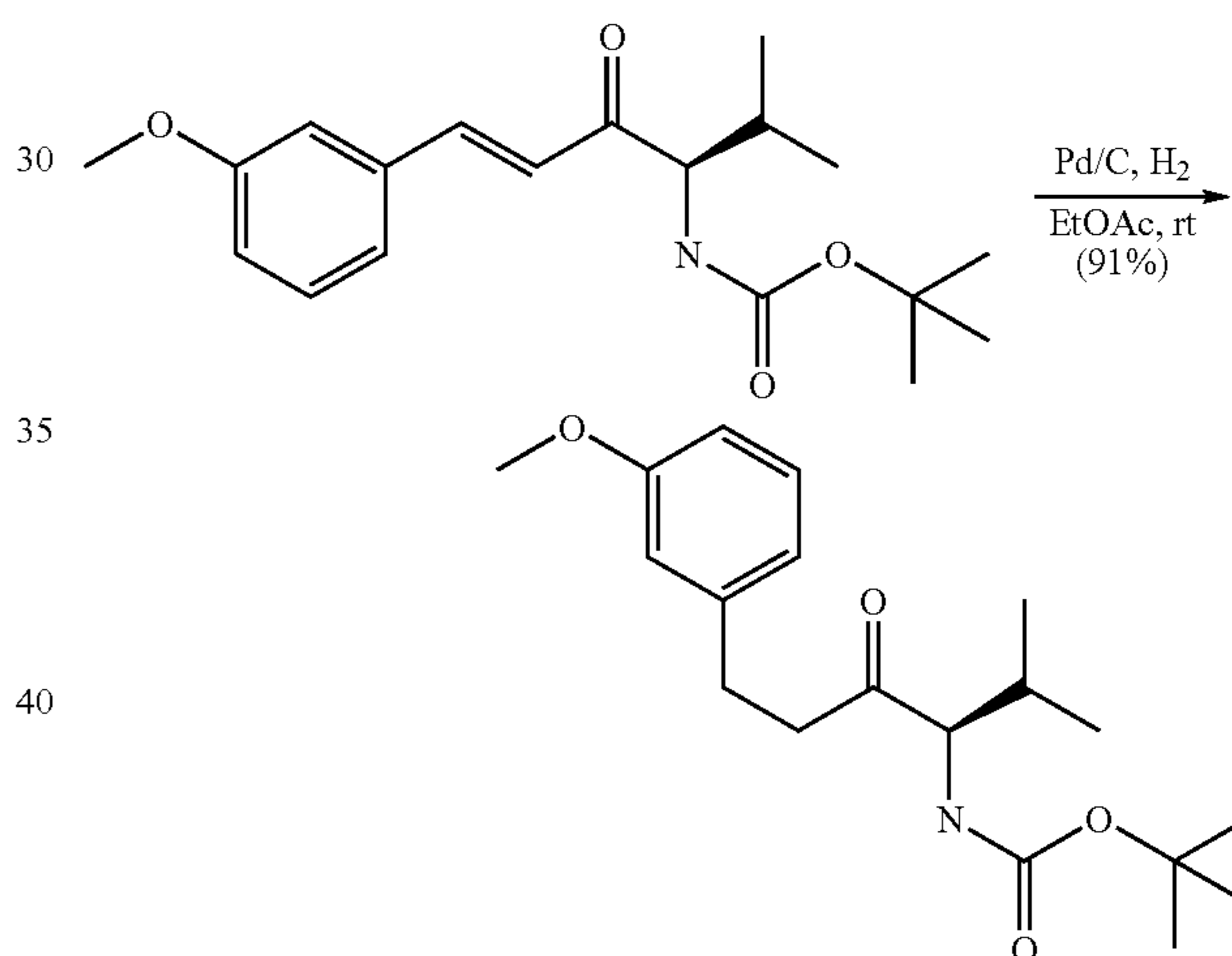
[(R)-E)-1-Isopropyl-4-(3-methoxy-phenyl)-2-oxo-butyl]-carbamic acid tert-butyl ester
