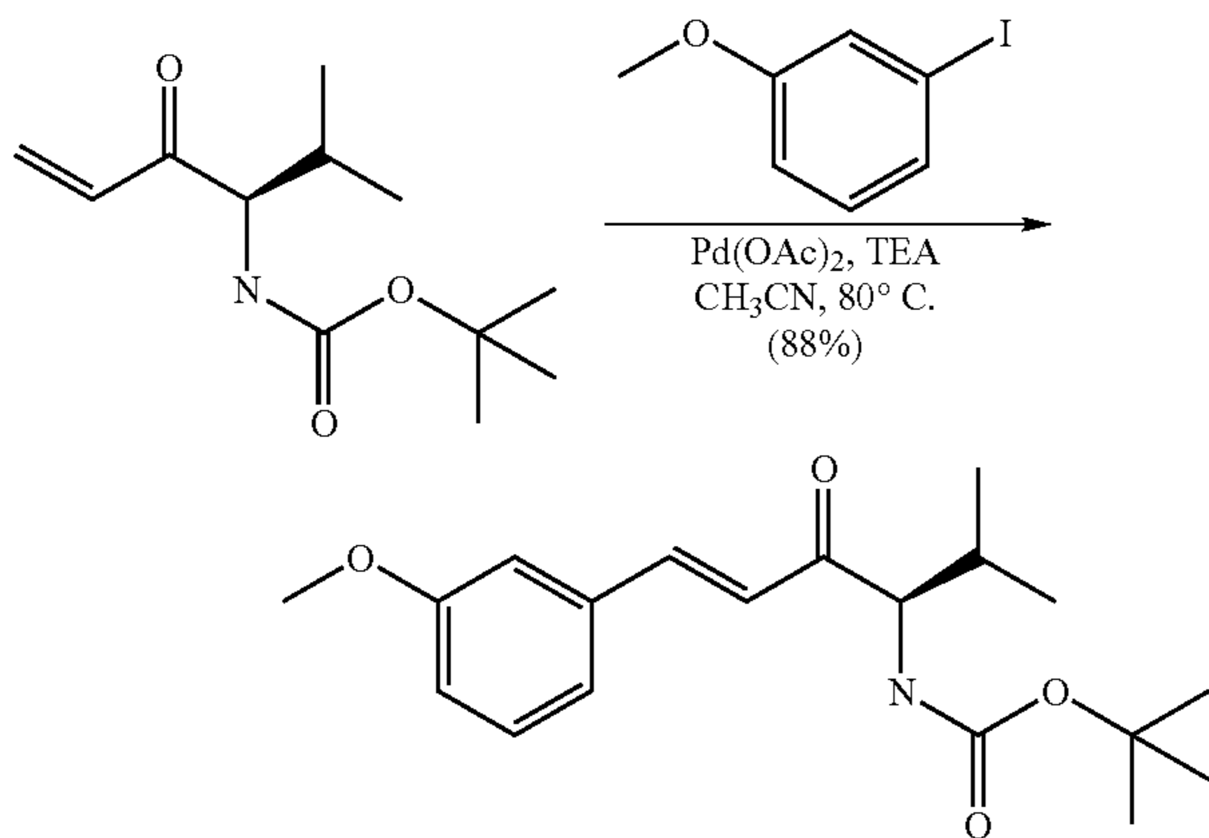
((R)-E)-1-Isopropyl-4-(3-methoxy-phenyl)-2-oxo-but-3-enyl]-carbamic acid tert-butyl ester
