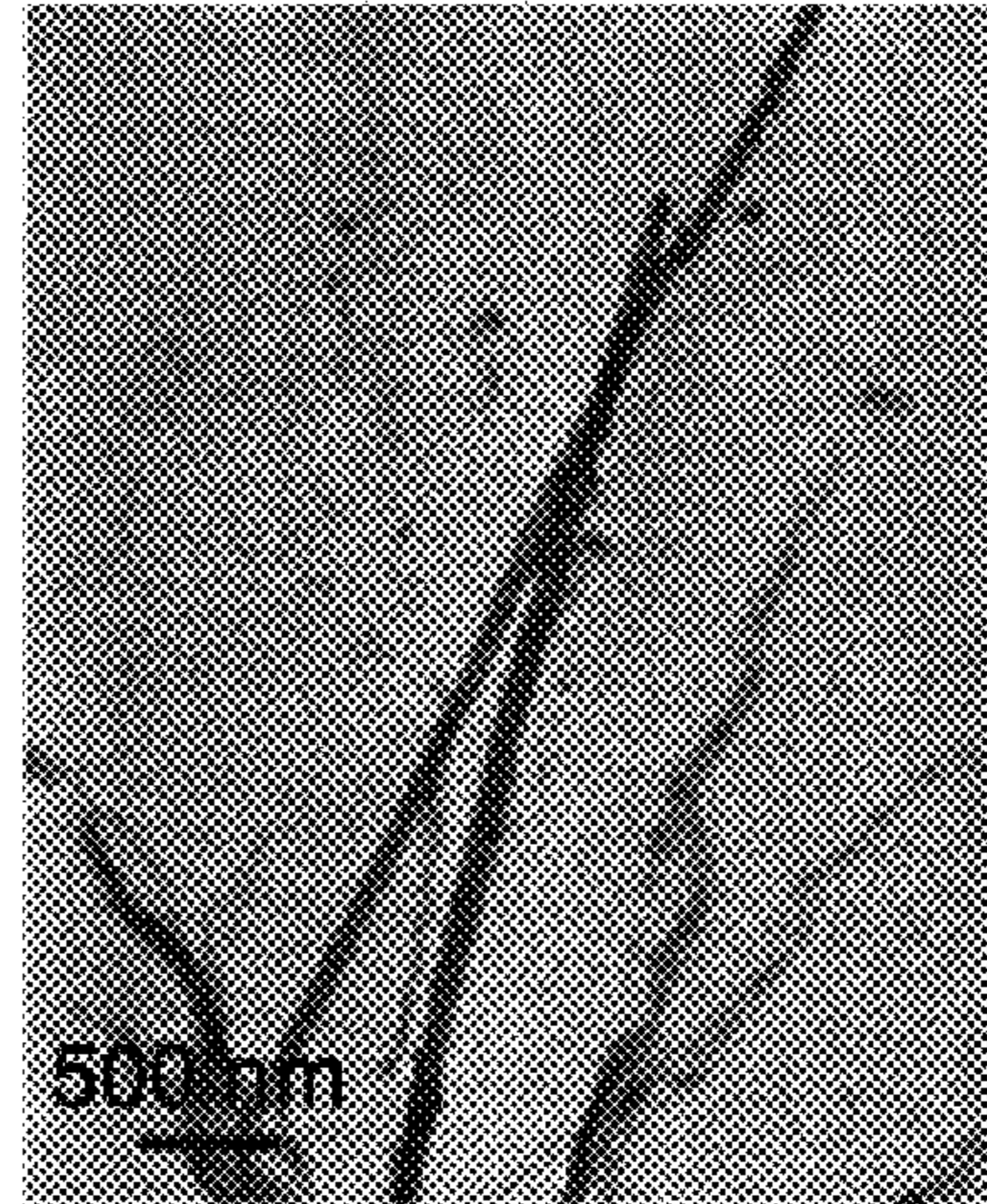
NH 2 -L-Phe-L-Trp-COOH
