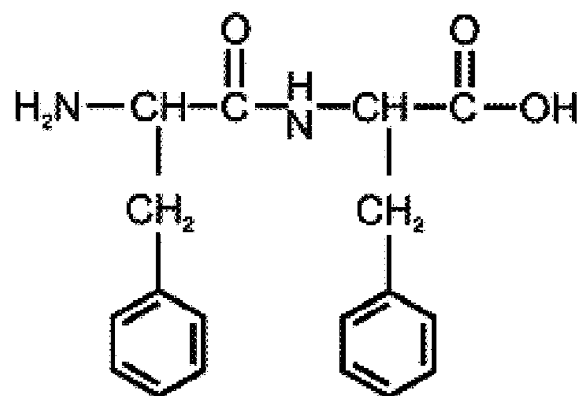
NH 2 -Phe-Phe-COOH
