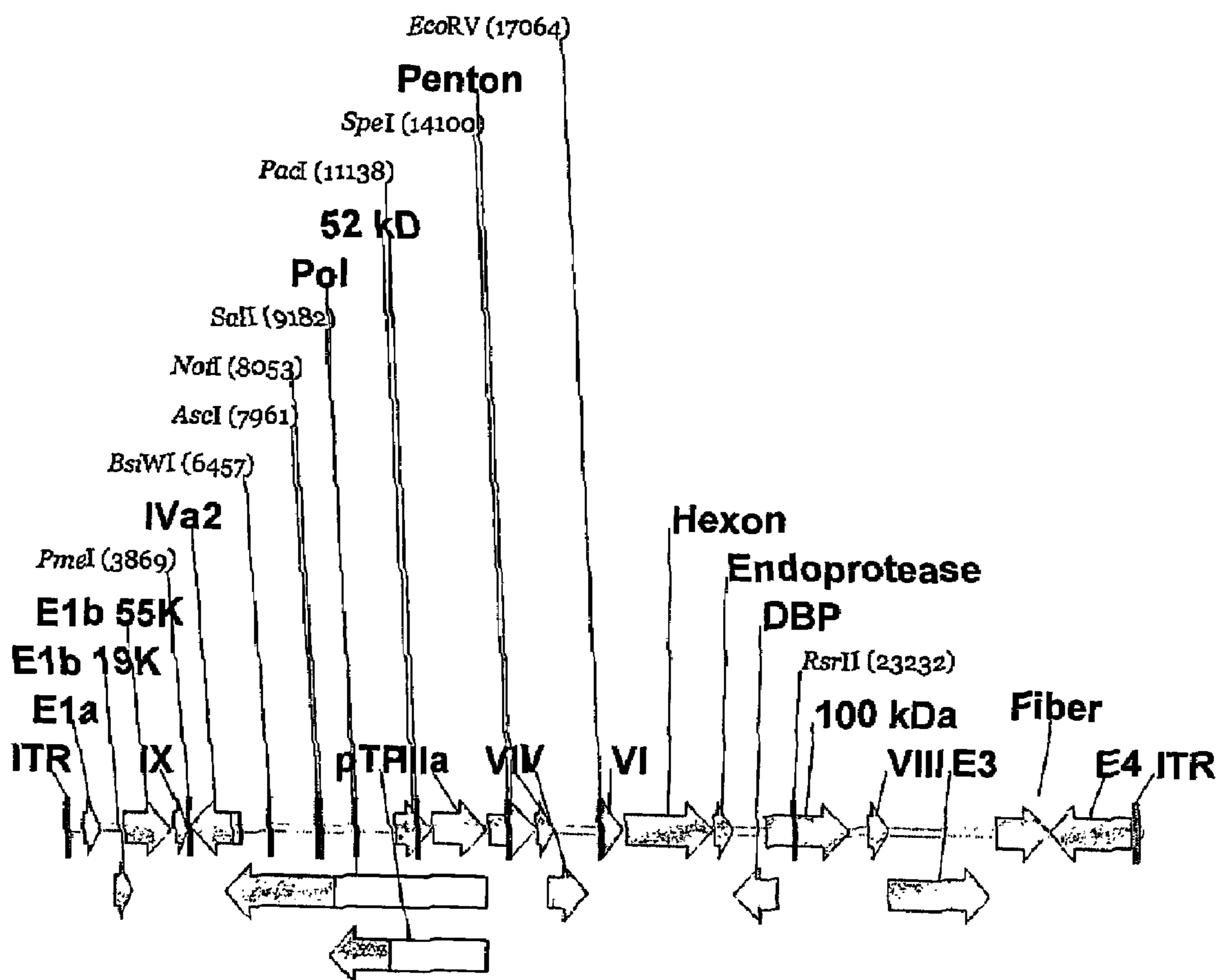
Simian Adenovirus 34302 bp
