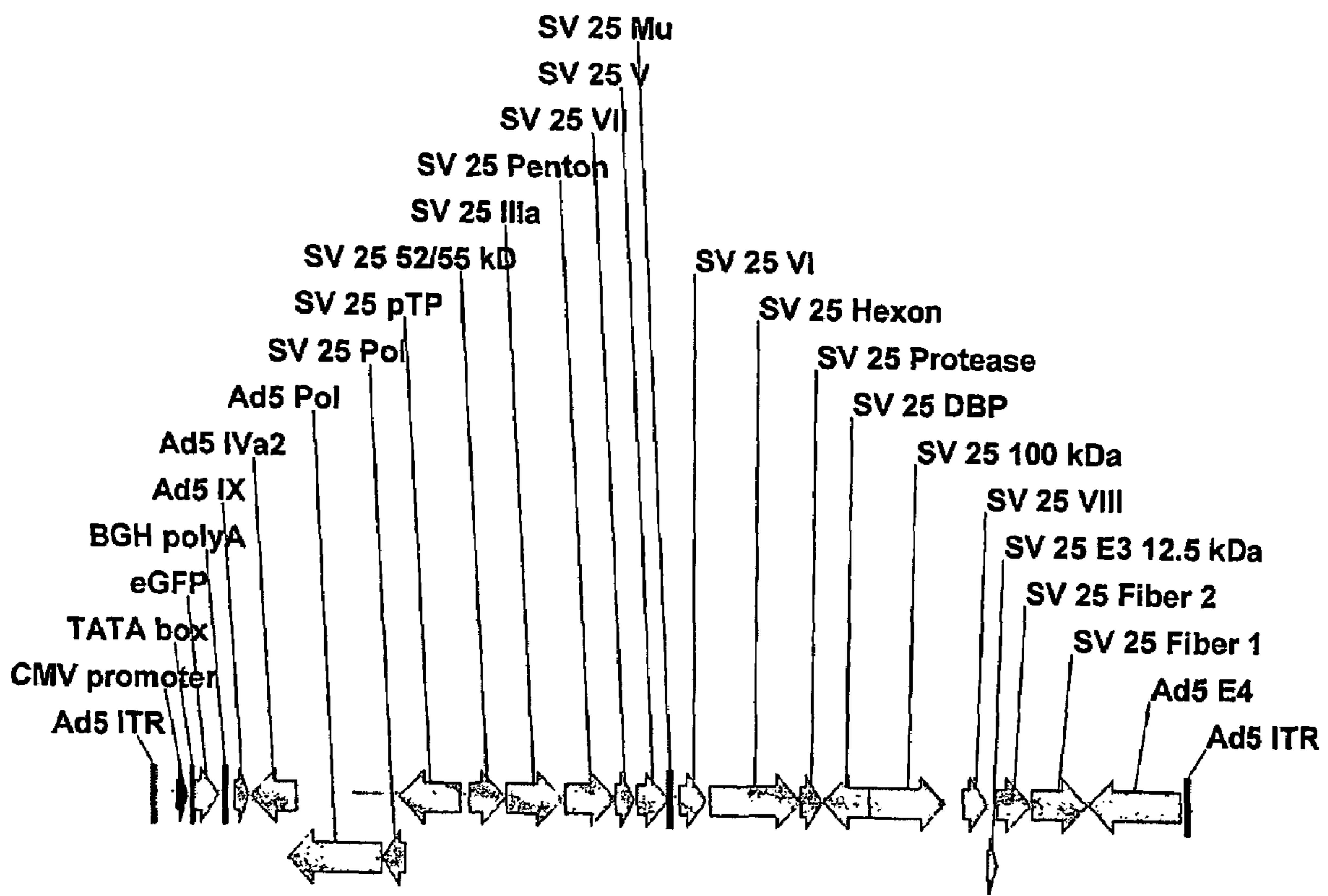
Ad H5S25H5eGFP 31518 bp
