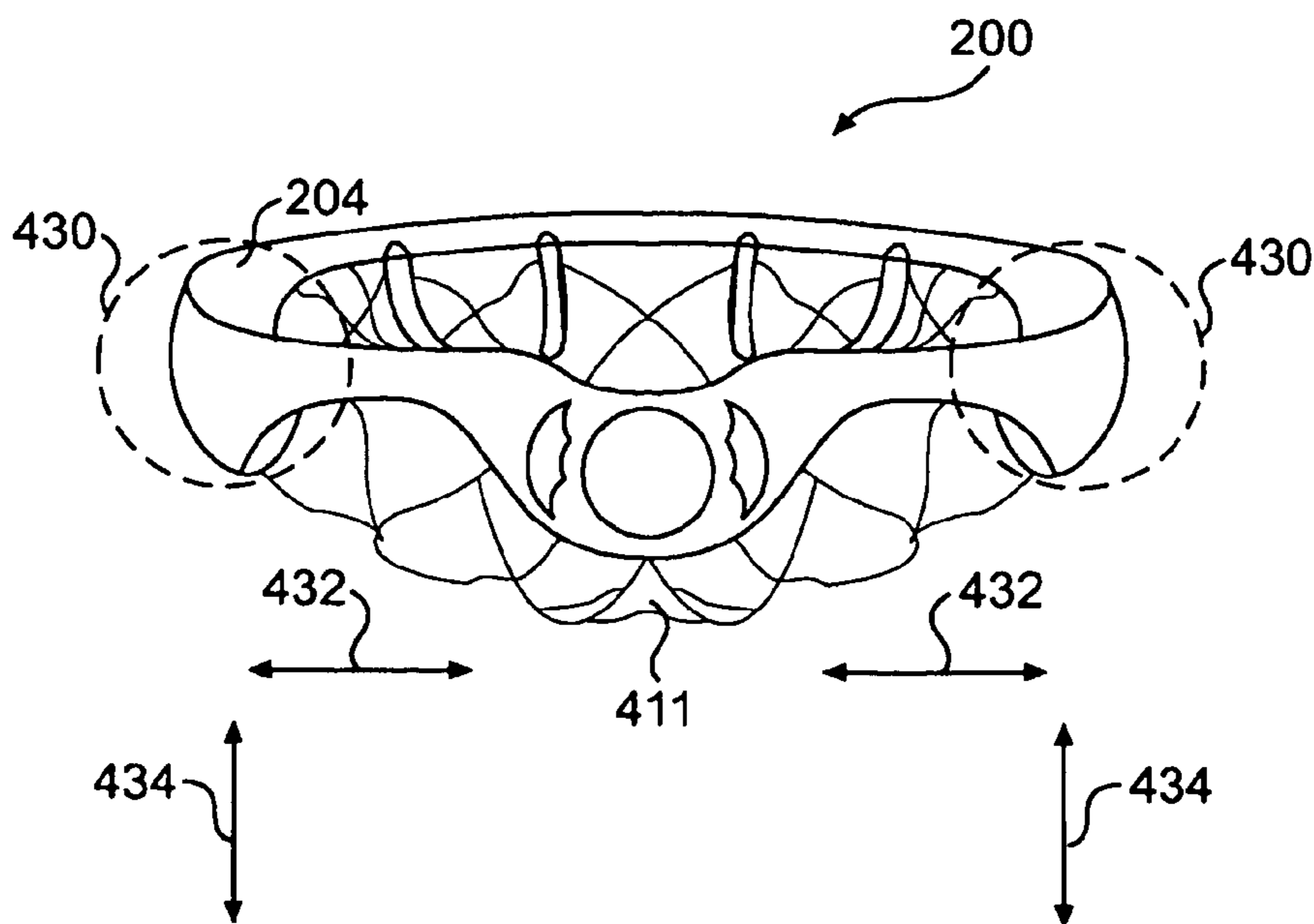
FIG. 4D
