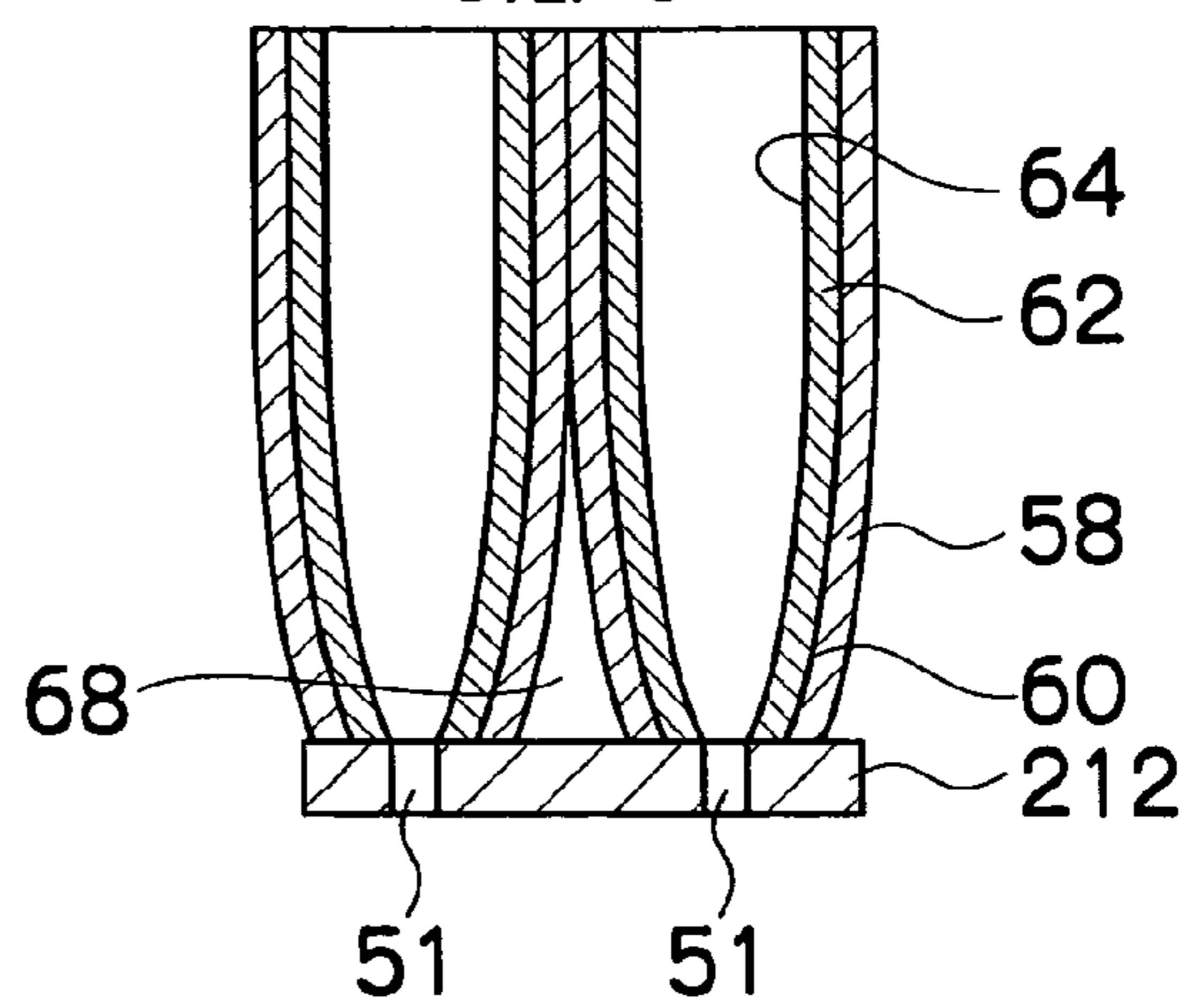
FIG.11E STEP 5
