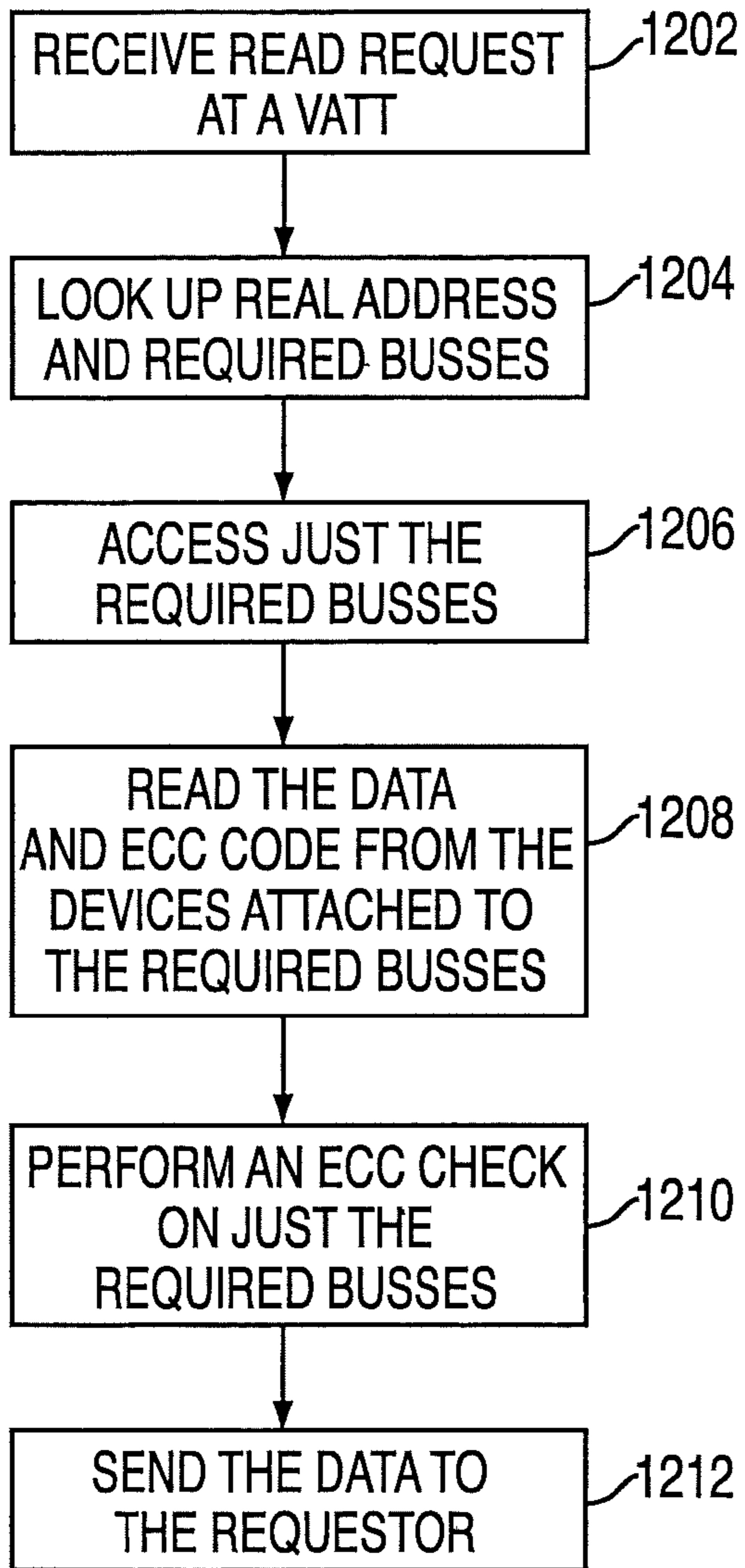
FIG. 12
