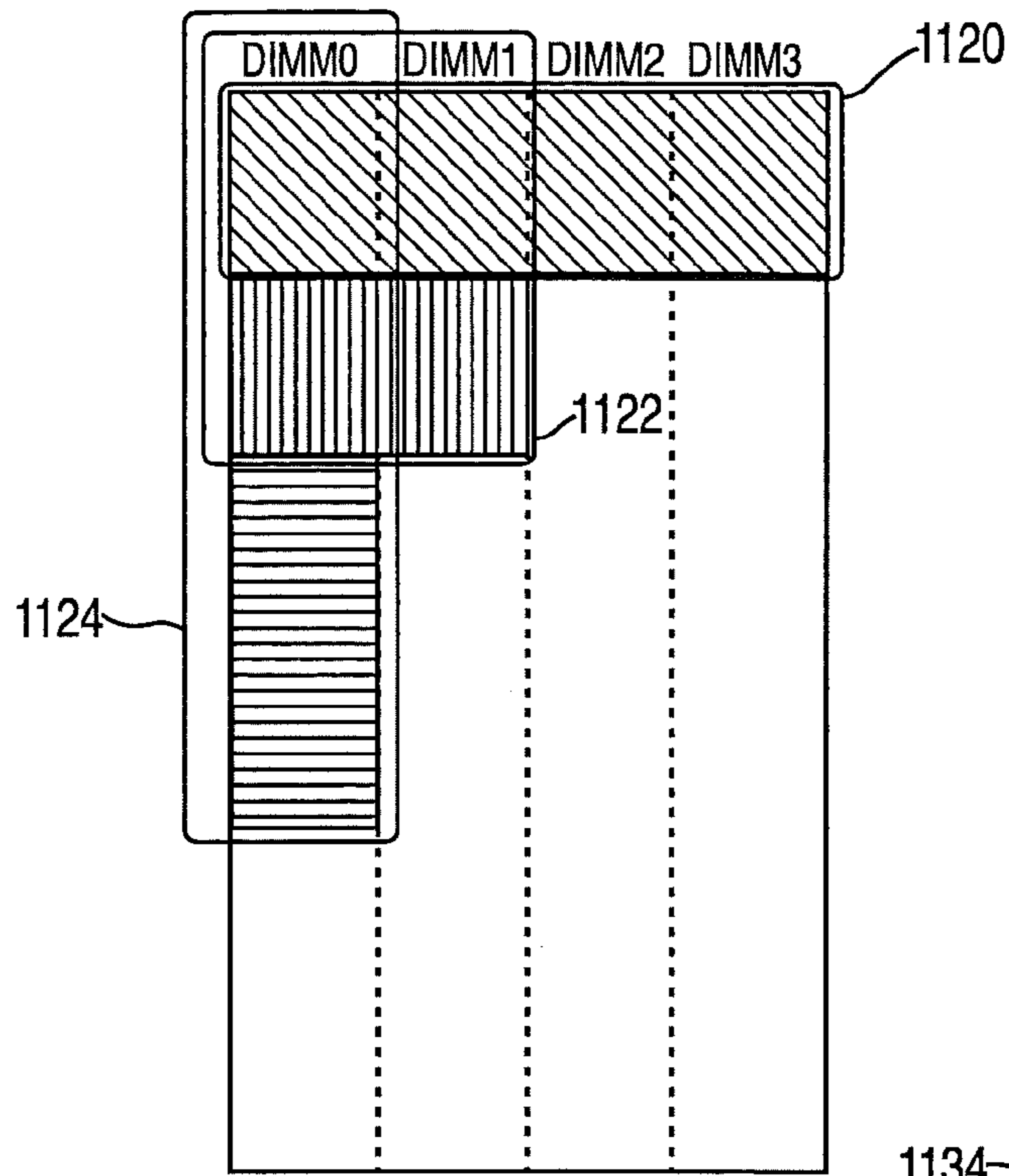
FIG. 11b
