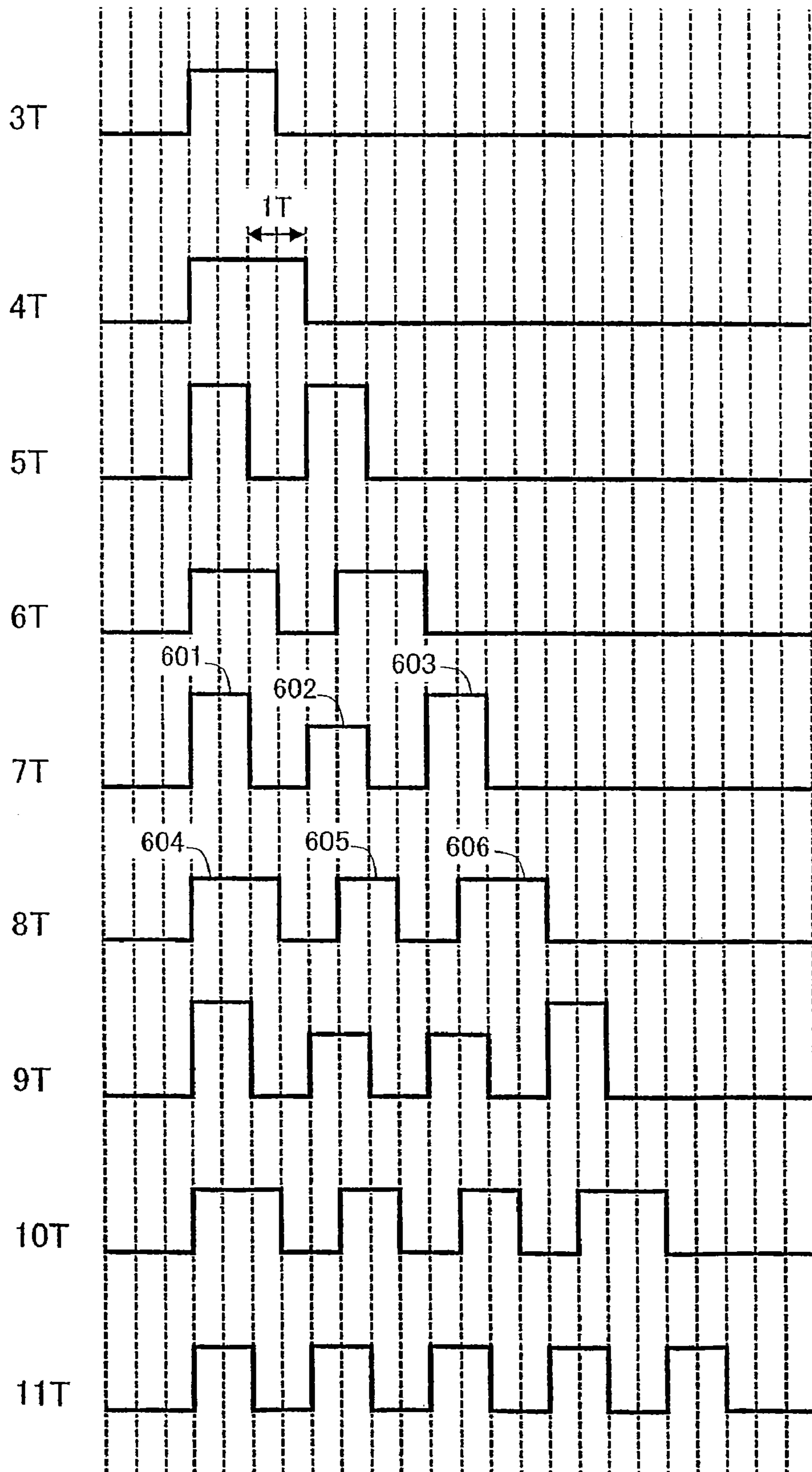
FIG. 16
