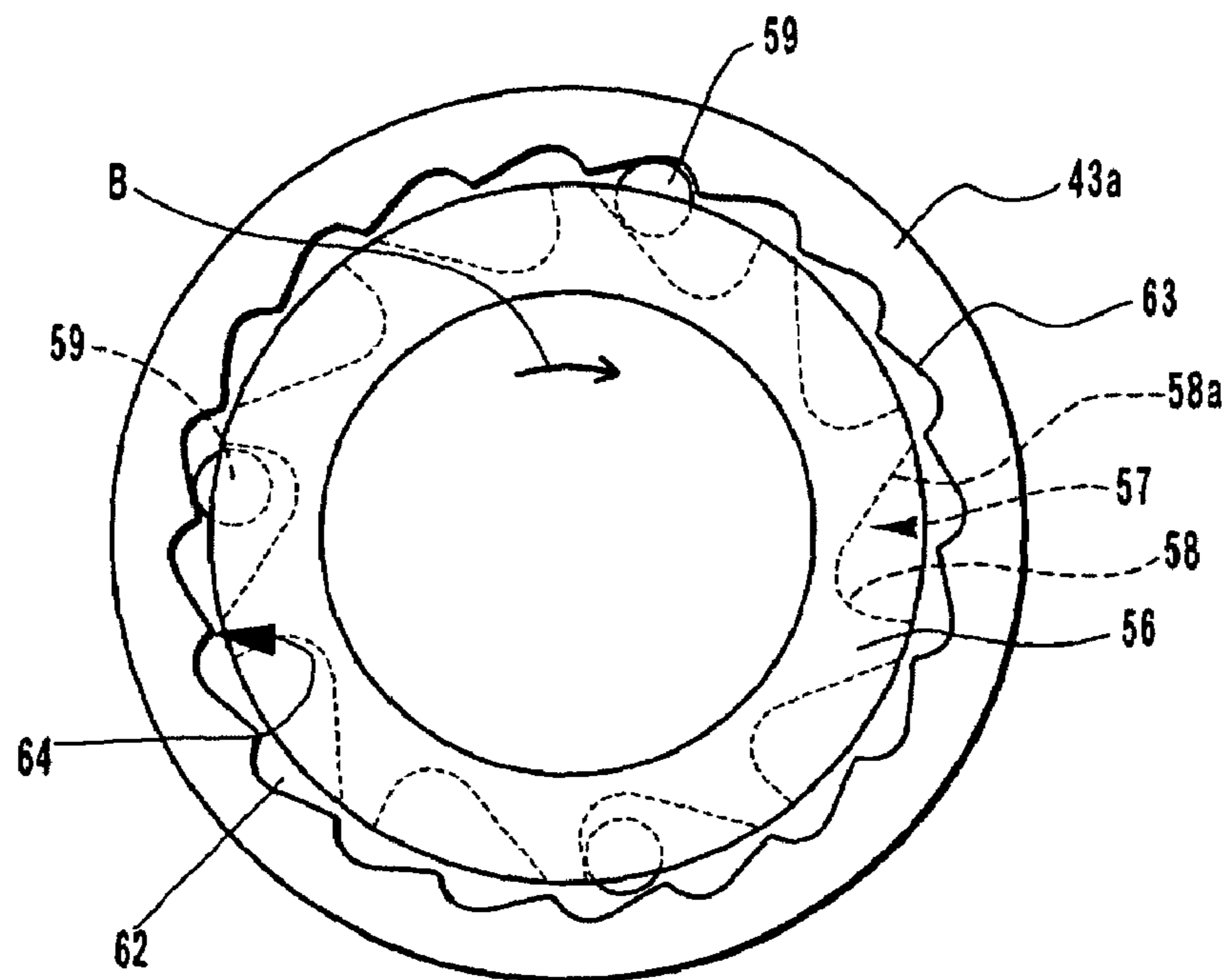
FIG. 6A
