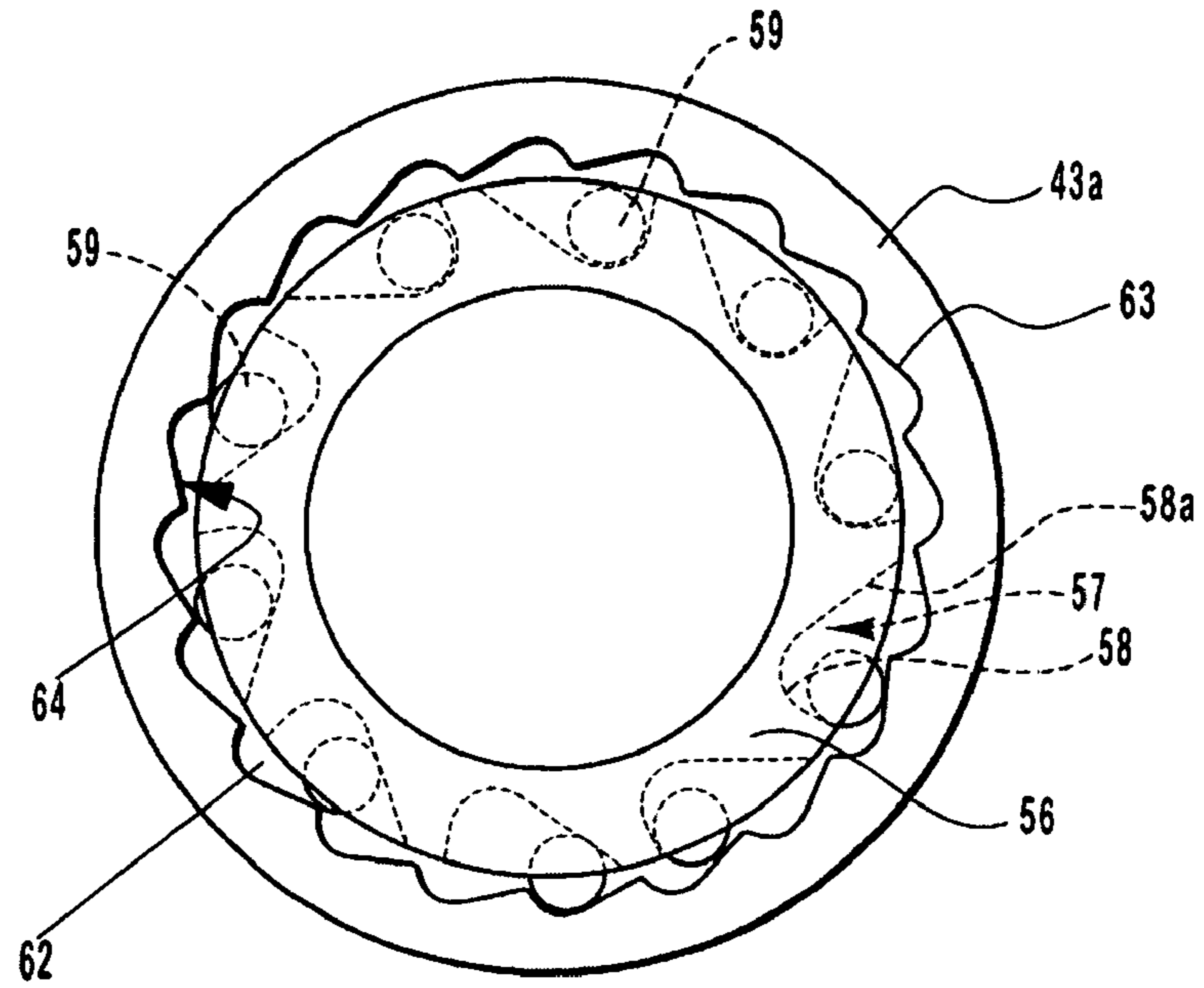
FIG. 6C
