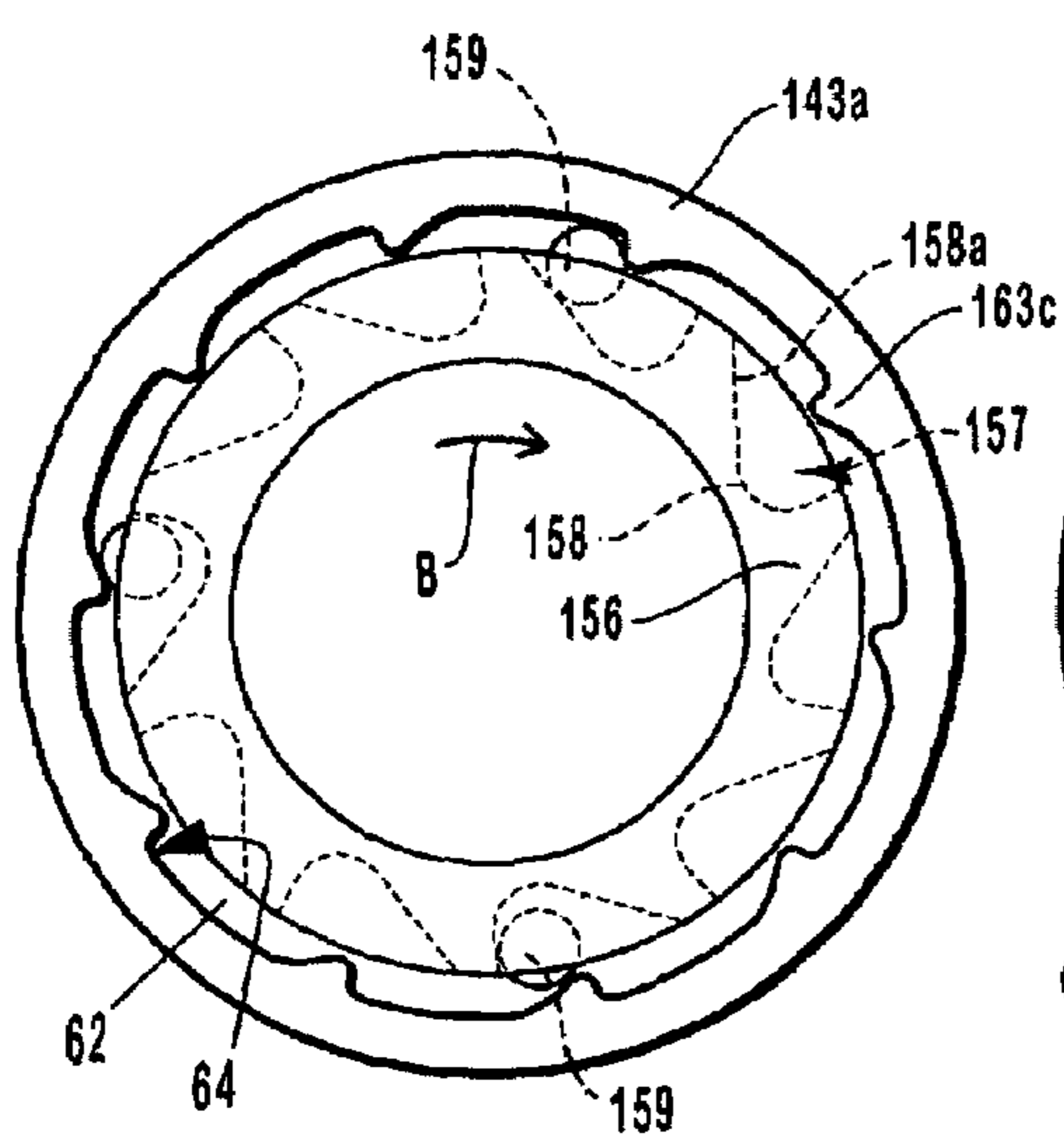
FIG. 8C
