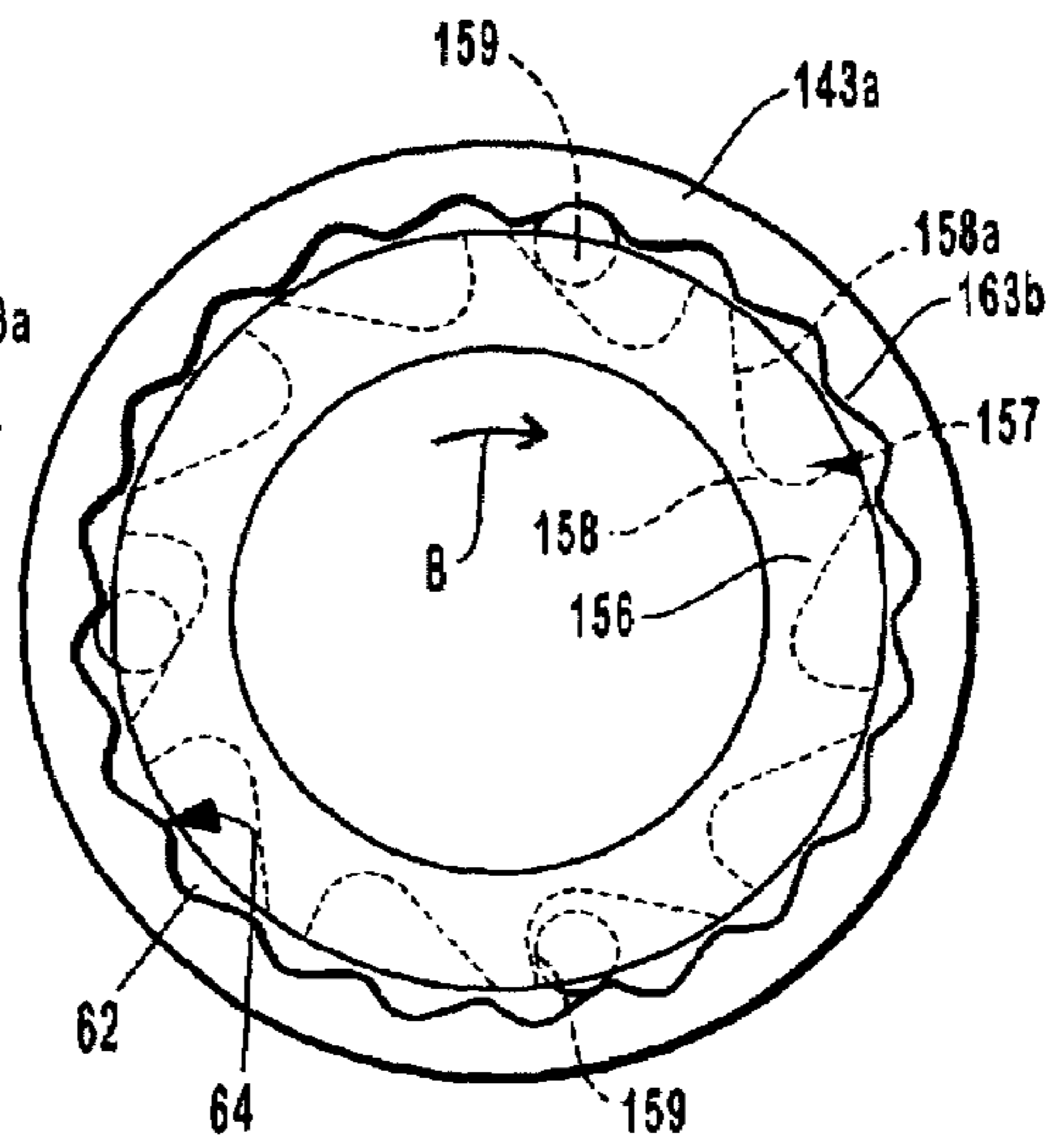
FIG. 8B
