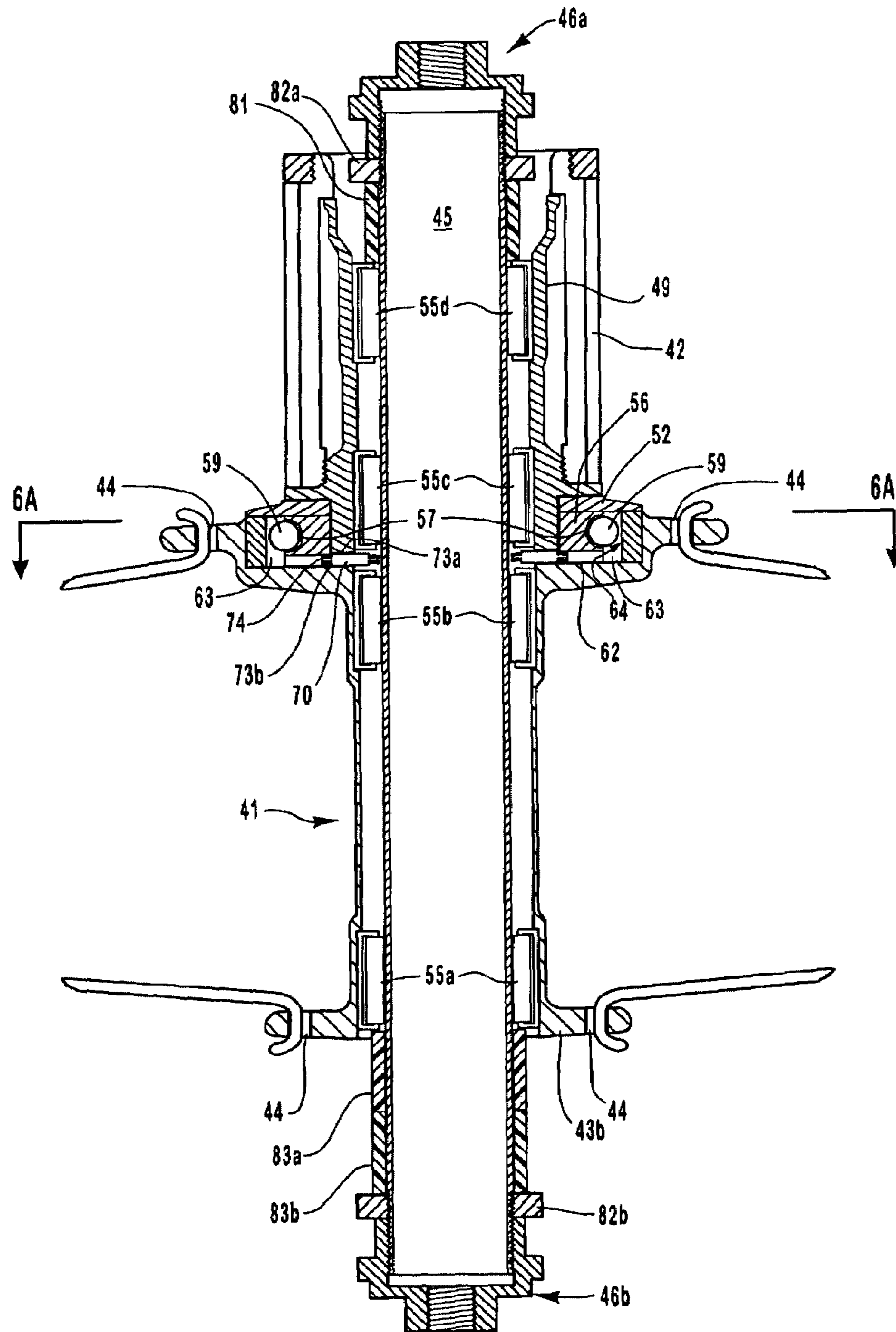
FIG. 5
