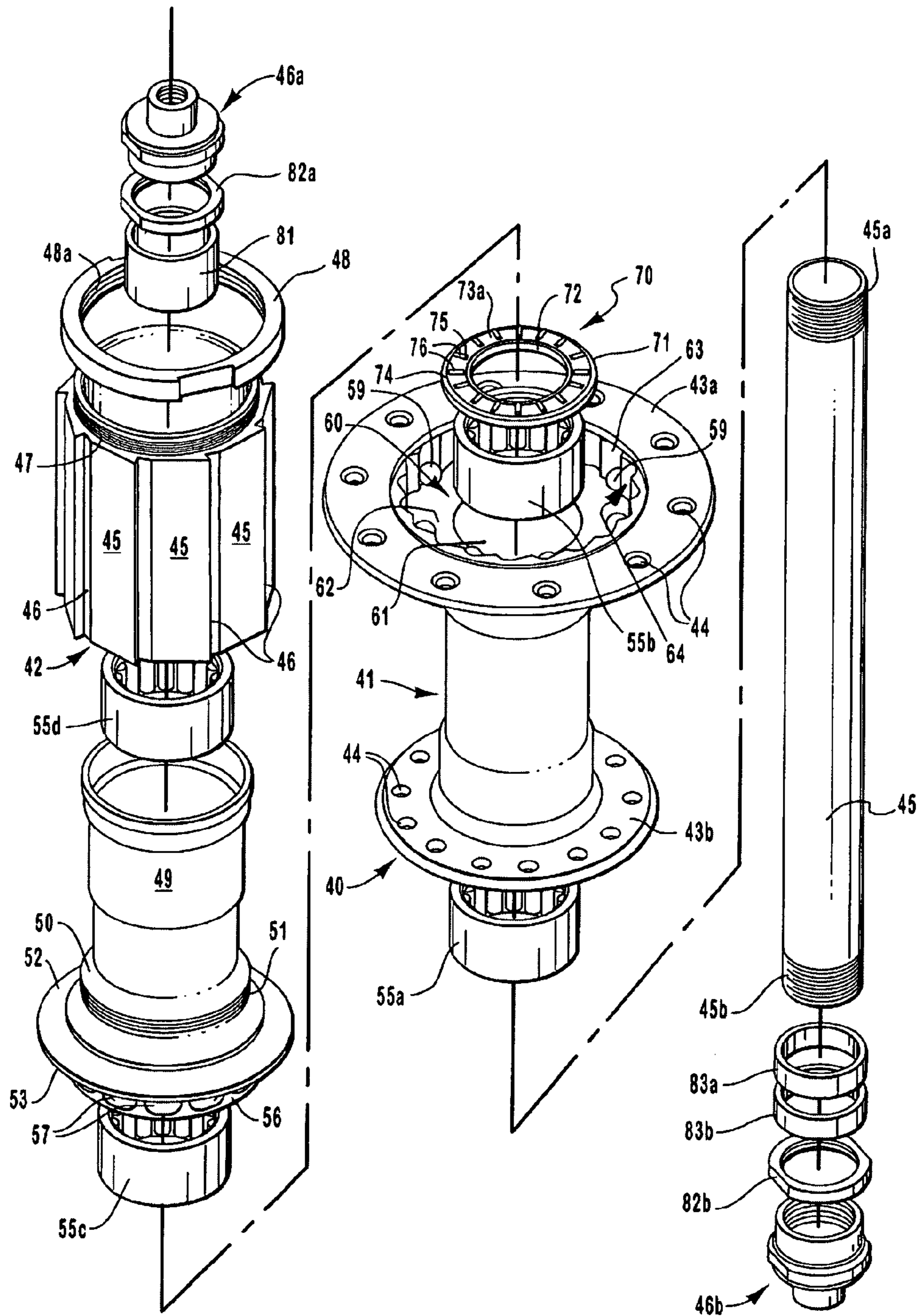
FIG. 4
