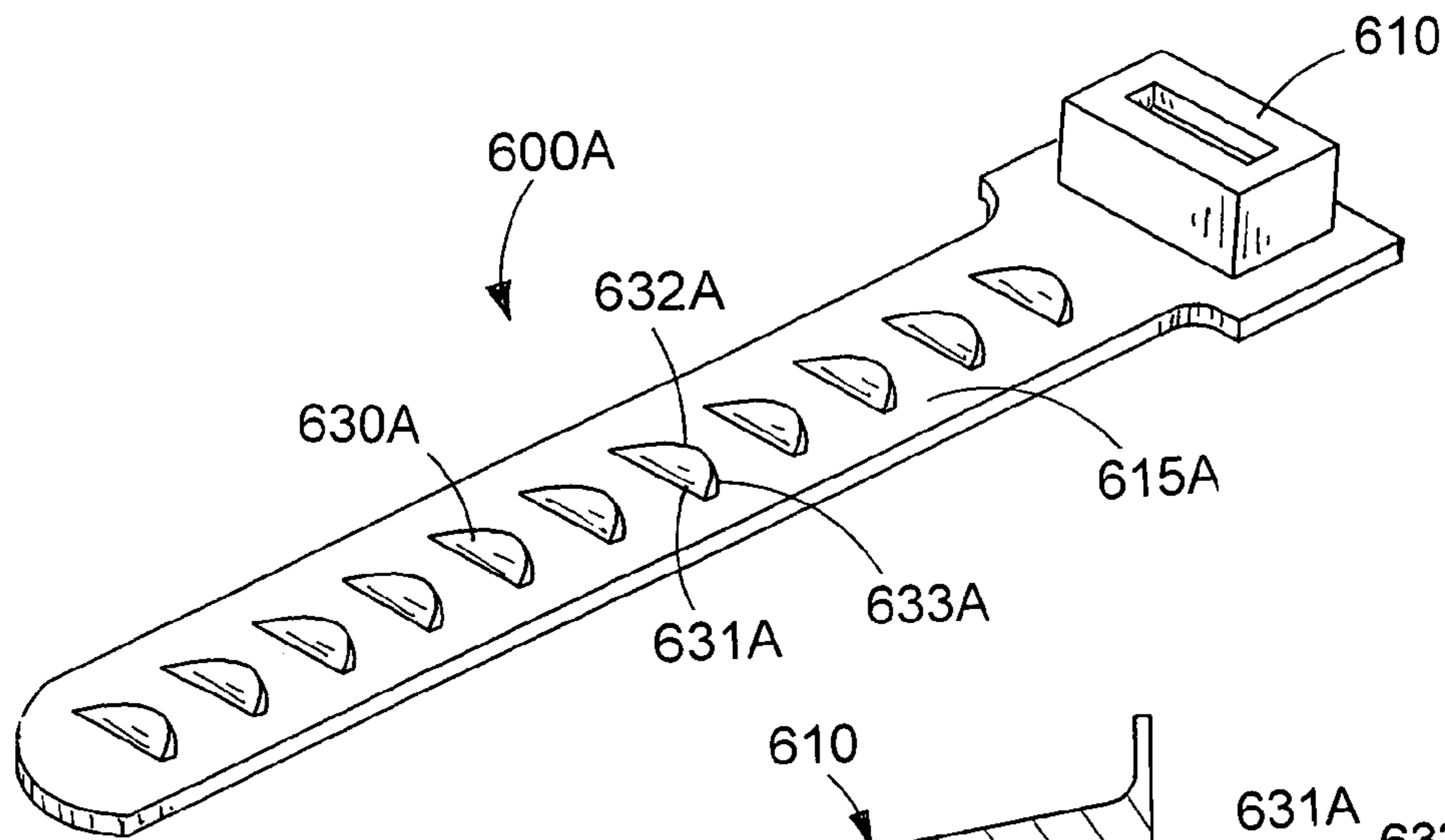
FIG. 22
