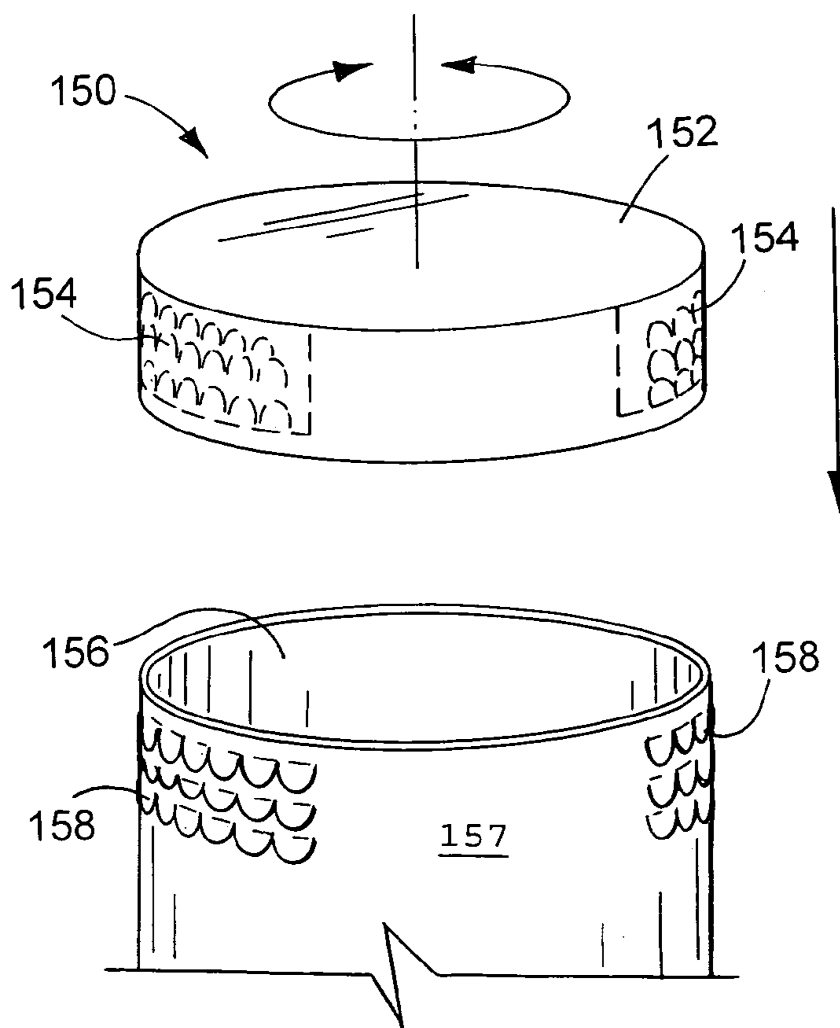
FIG. 19
