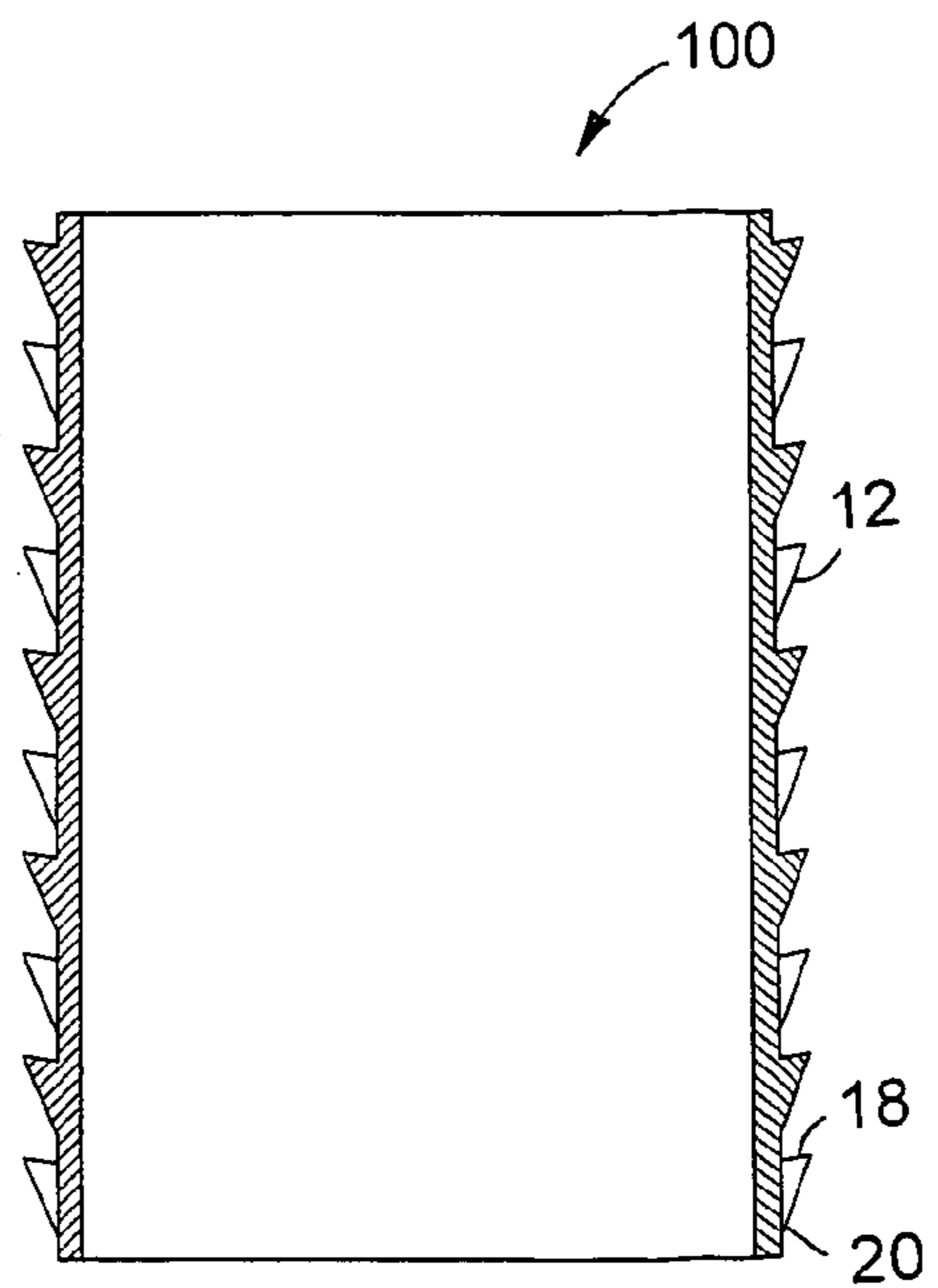
FIG. 11A
