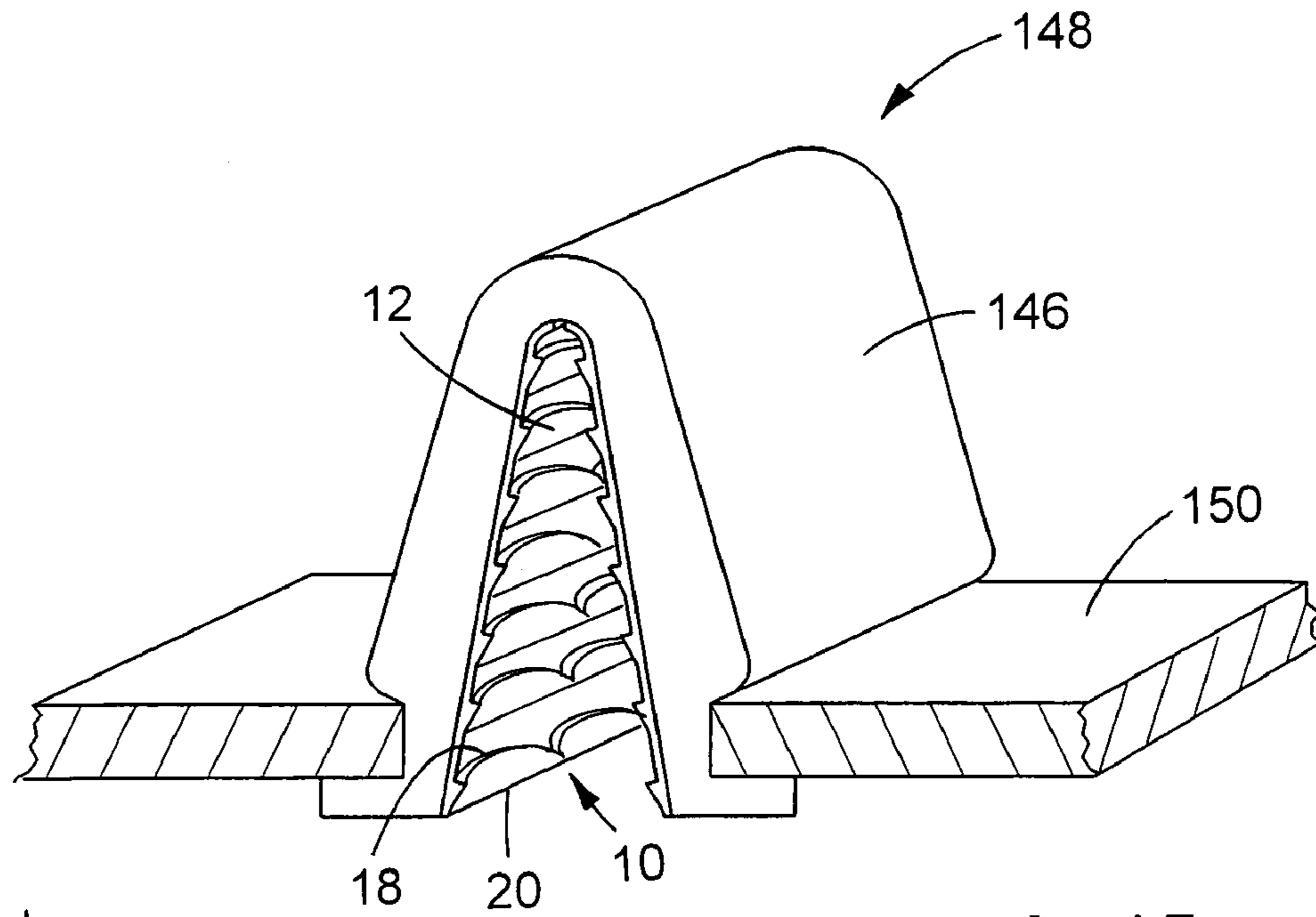
FIG. 15
