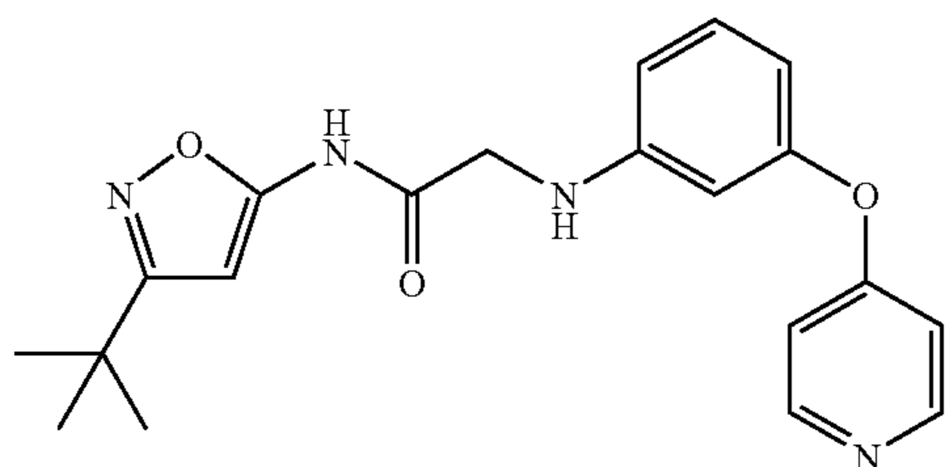
(5): N-(3-tert.-Butyl-isoxazol-5-yl)-2-[3-(pyridin-4-yloxy)-phenylamino]-acetamide
