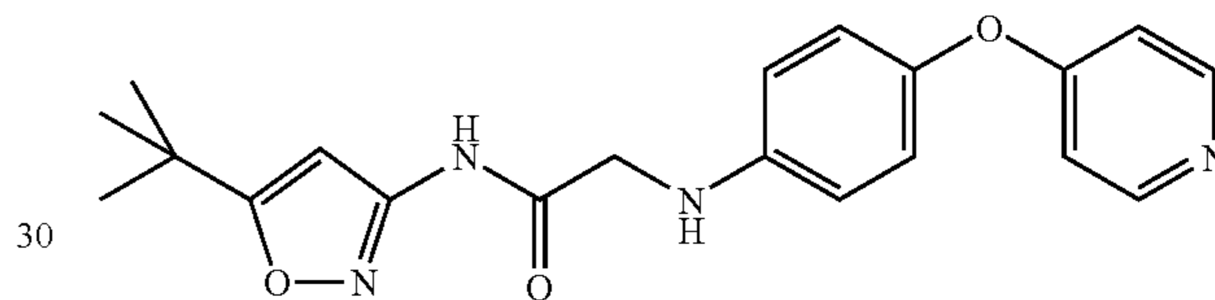
(5): N-(3-tert.-Butyl-isoxazol-5-yl)-2-[3-(pyridin-4-yloxy)-phenylamino]-acetamide
