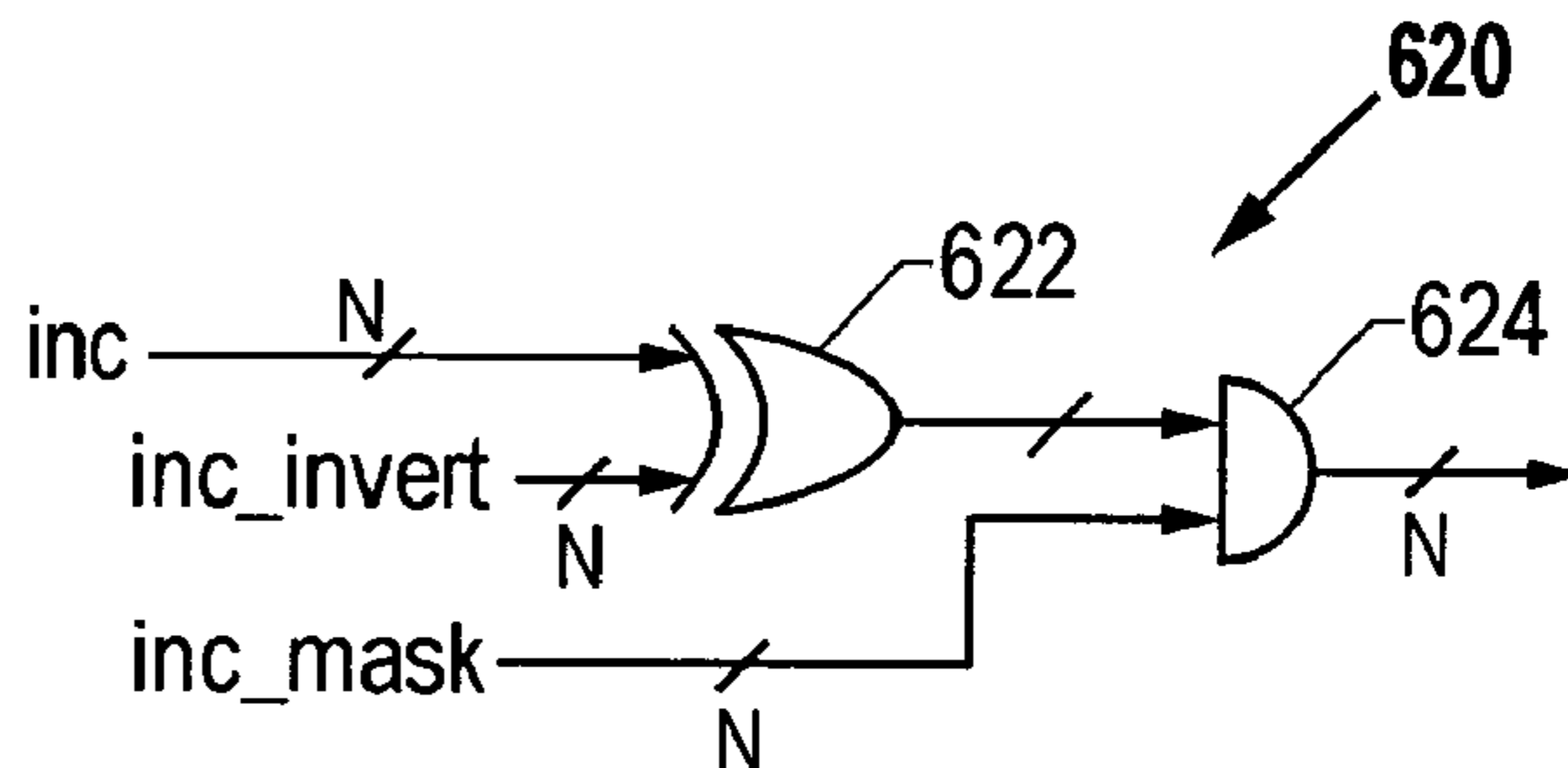
FIG. 6A
