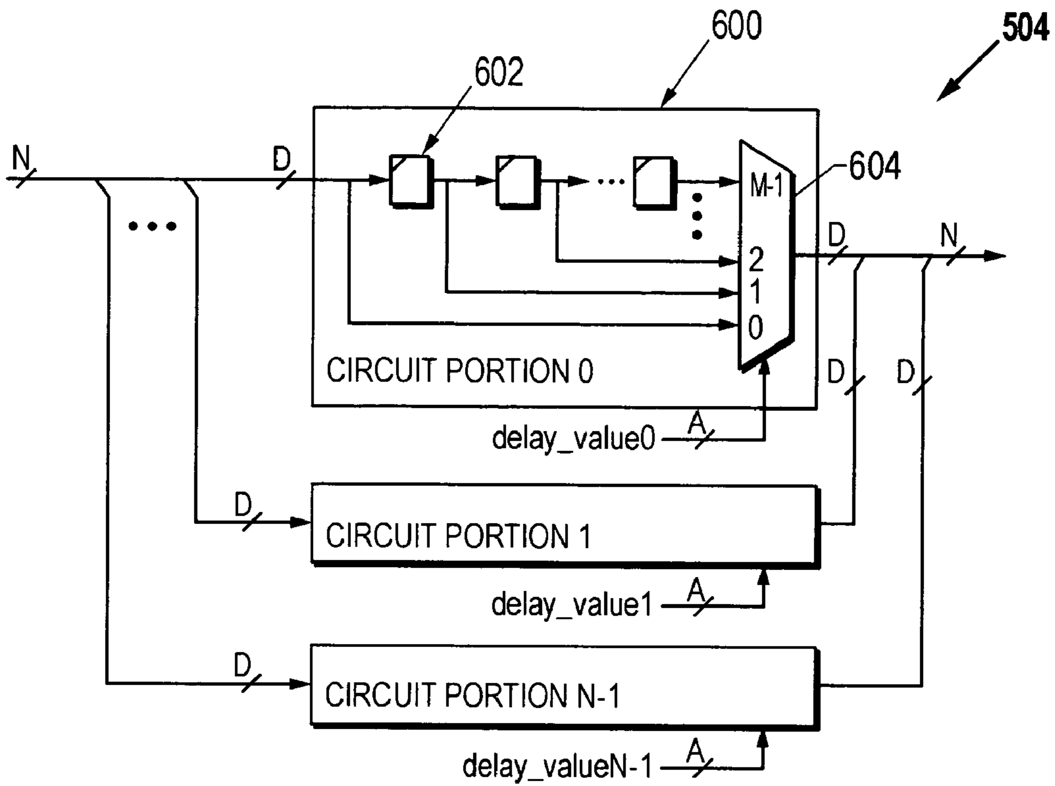
FIG. 6A
