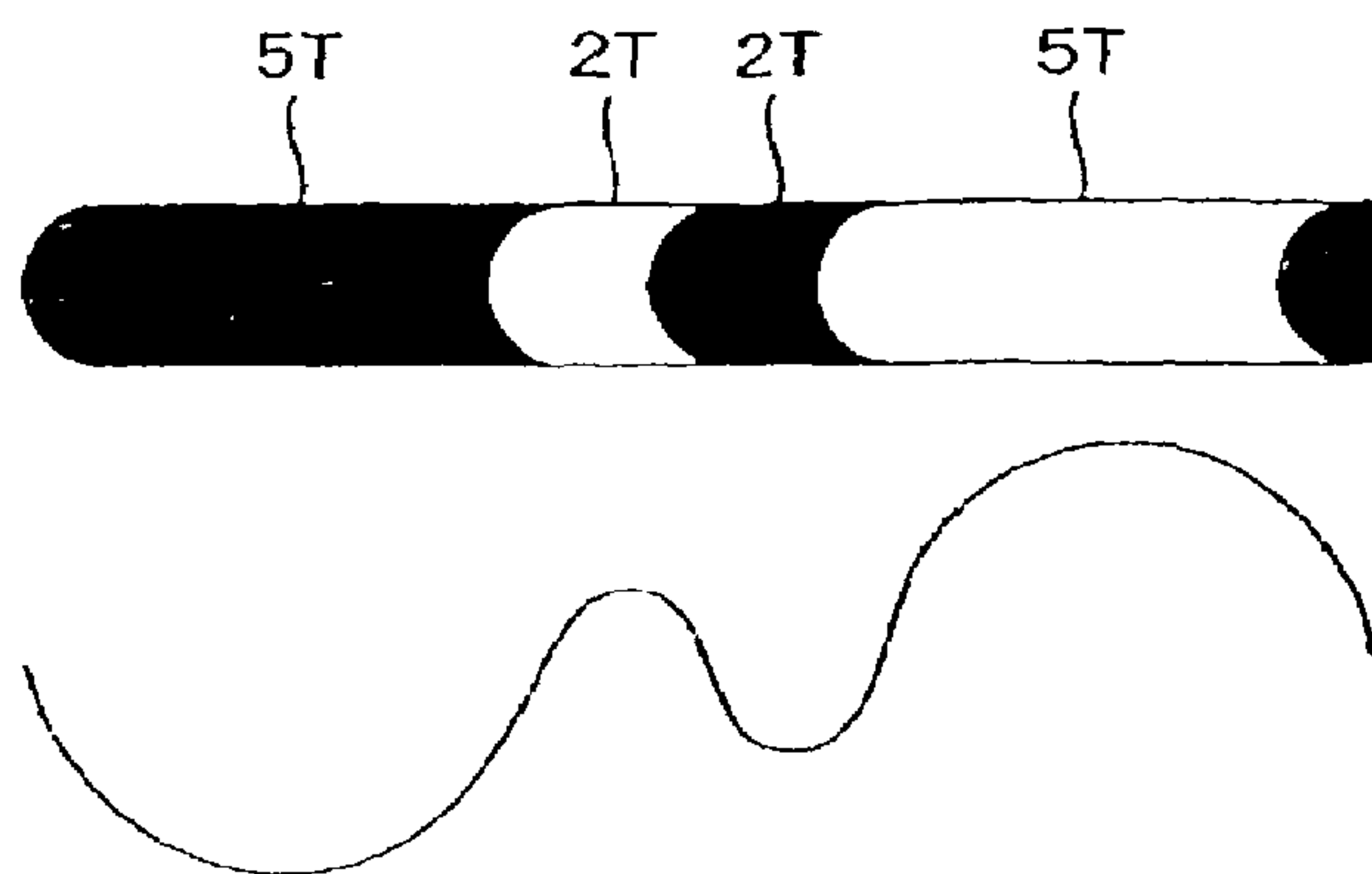
FIG. 8 (d) 5T2T2T5T (PRIOR ART)
