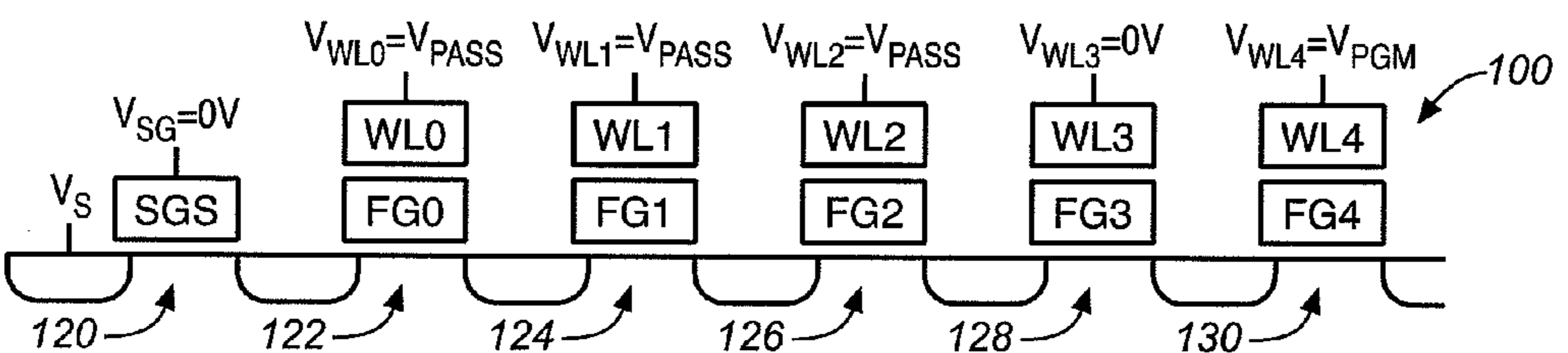
FIG. 6E (PRIOR ART)
