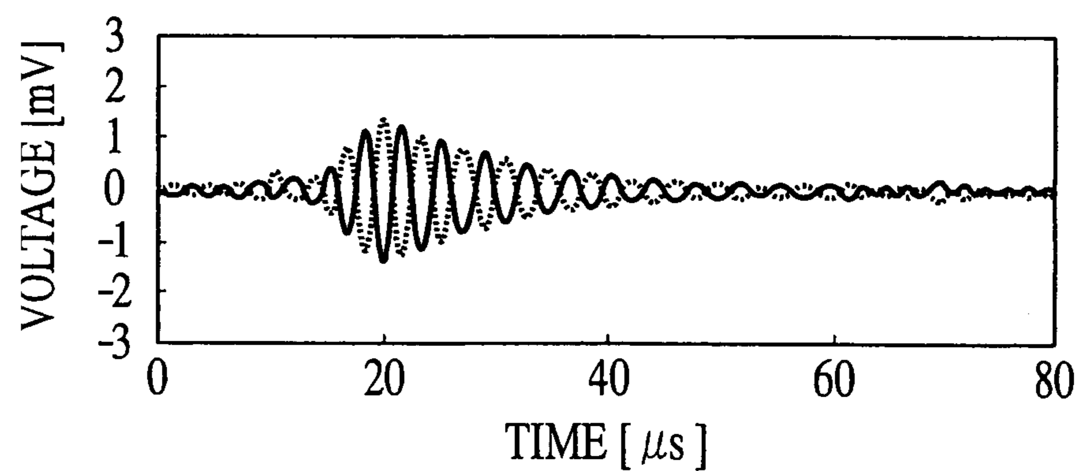
FIG.9B \theta = 45^\circ
