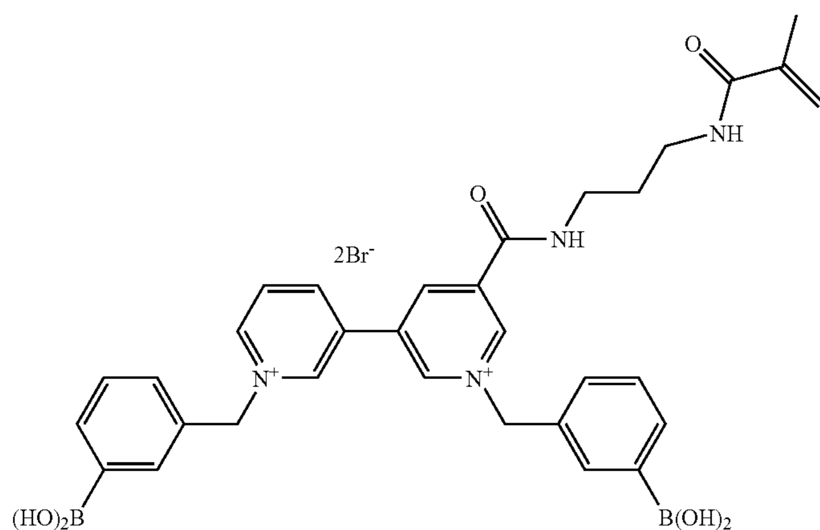
3,3'-mBBV
