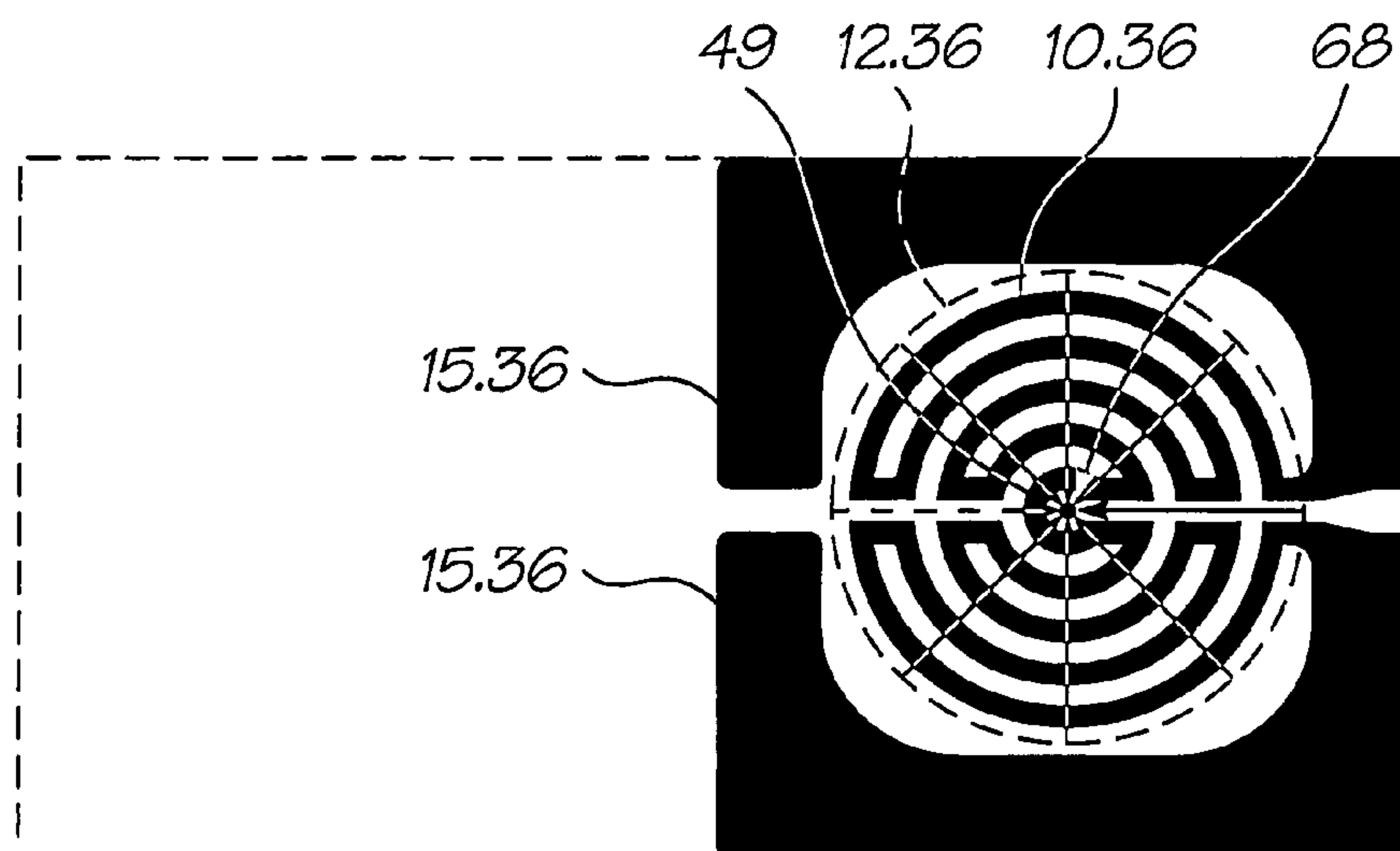
FIG. 36
