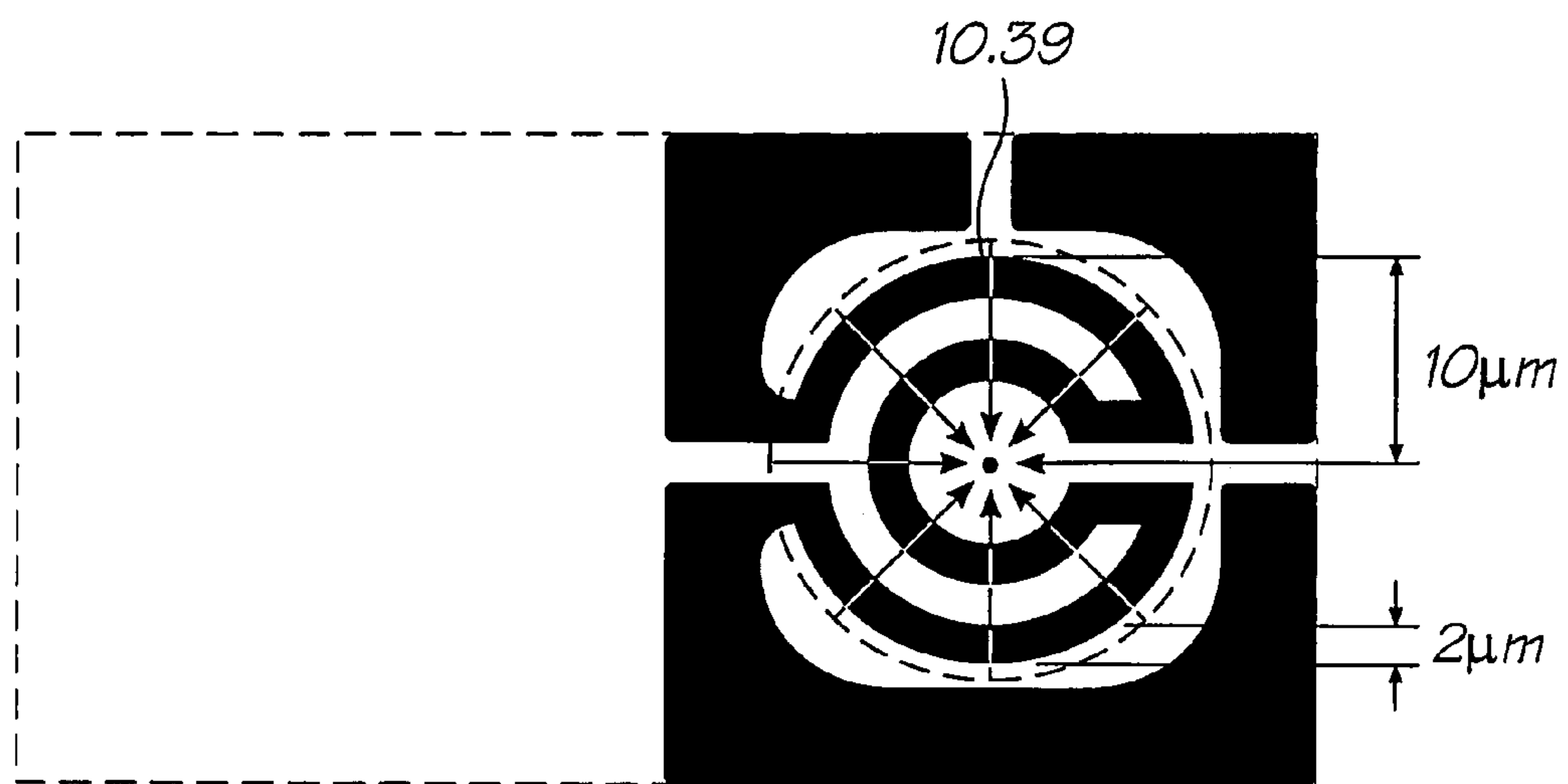
FIG. 39
