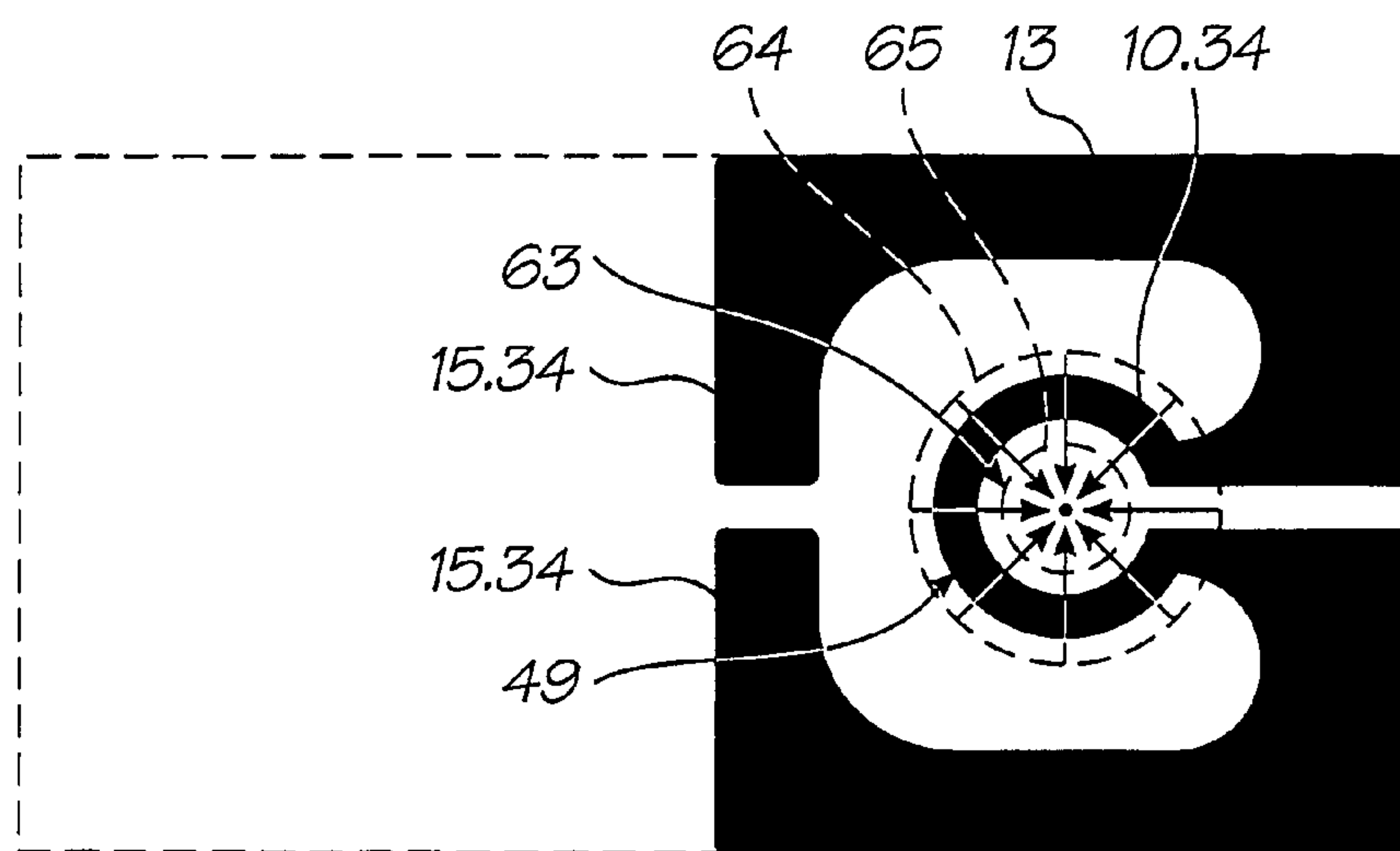
FIG. 34
