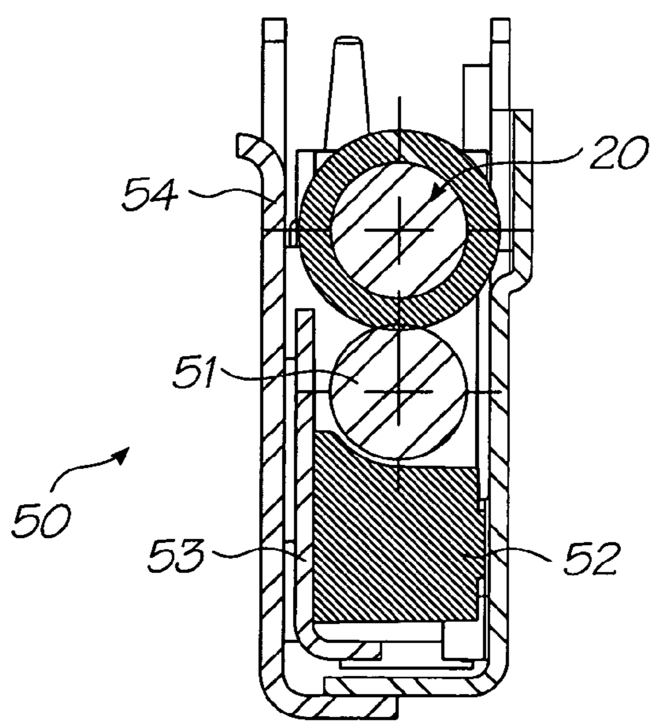
Section A-A
