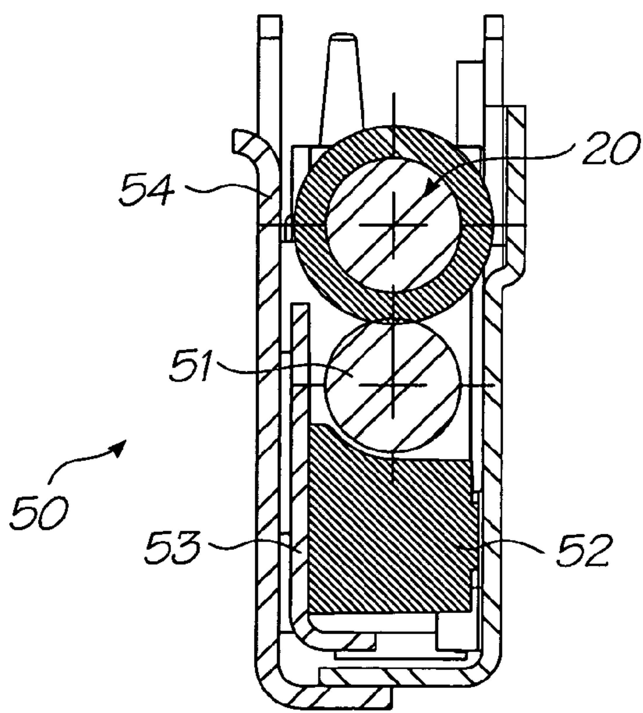
Section A-A
