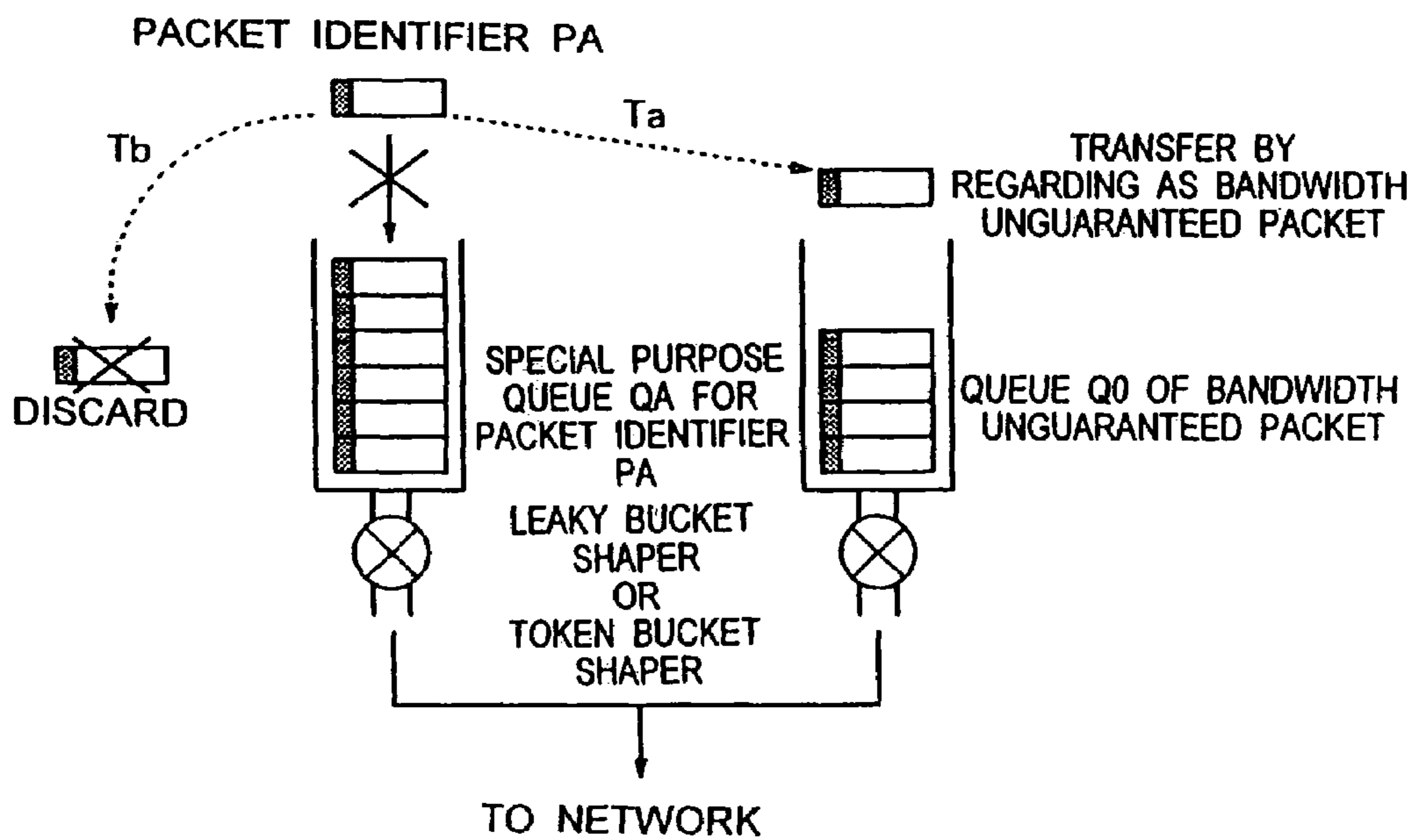
PRIOR ART FIG. 9A
