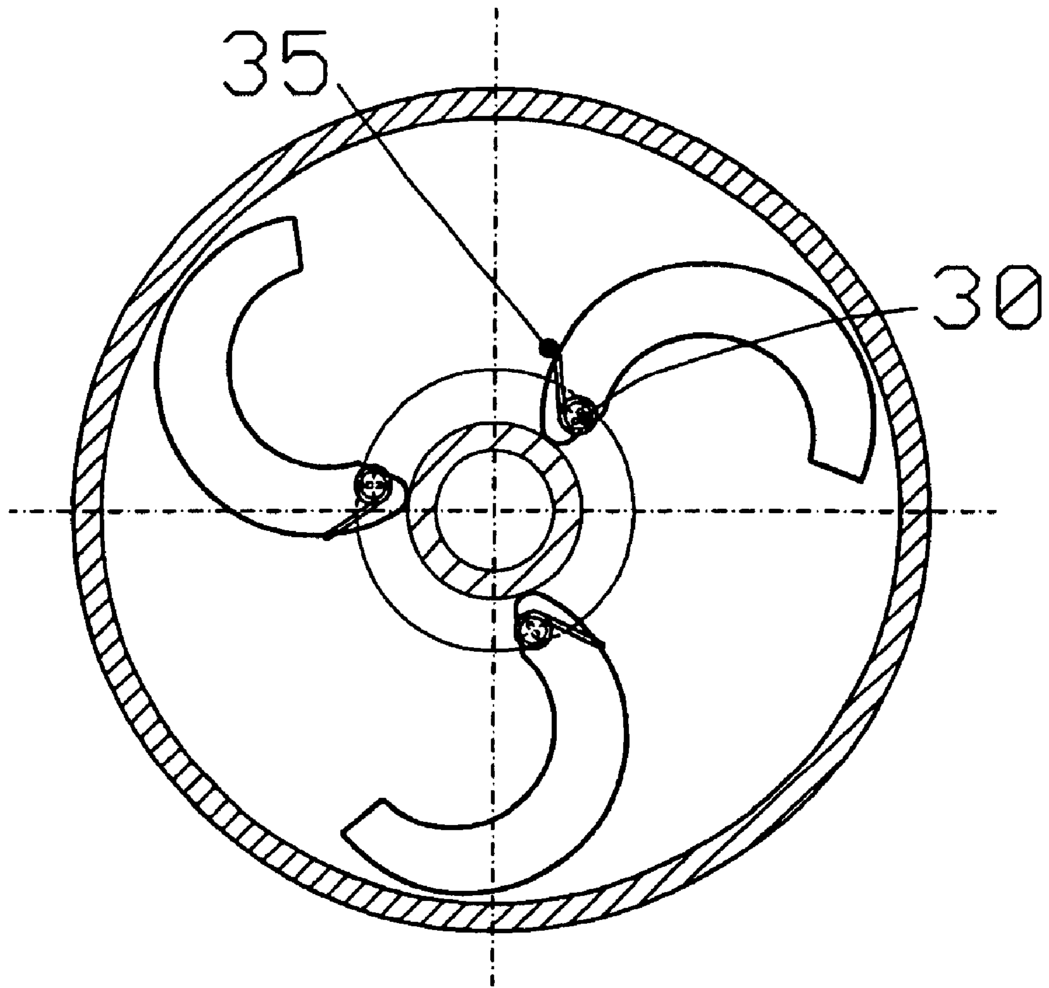
Fig.4F section A-A
