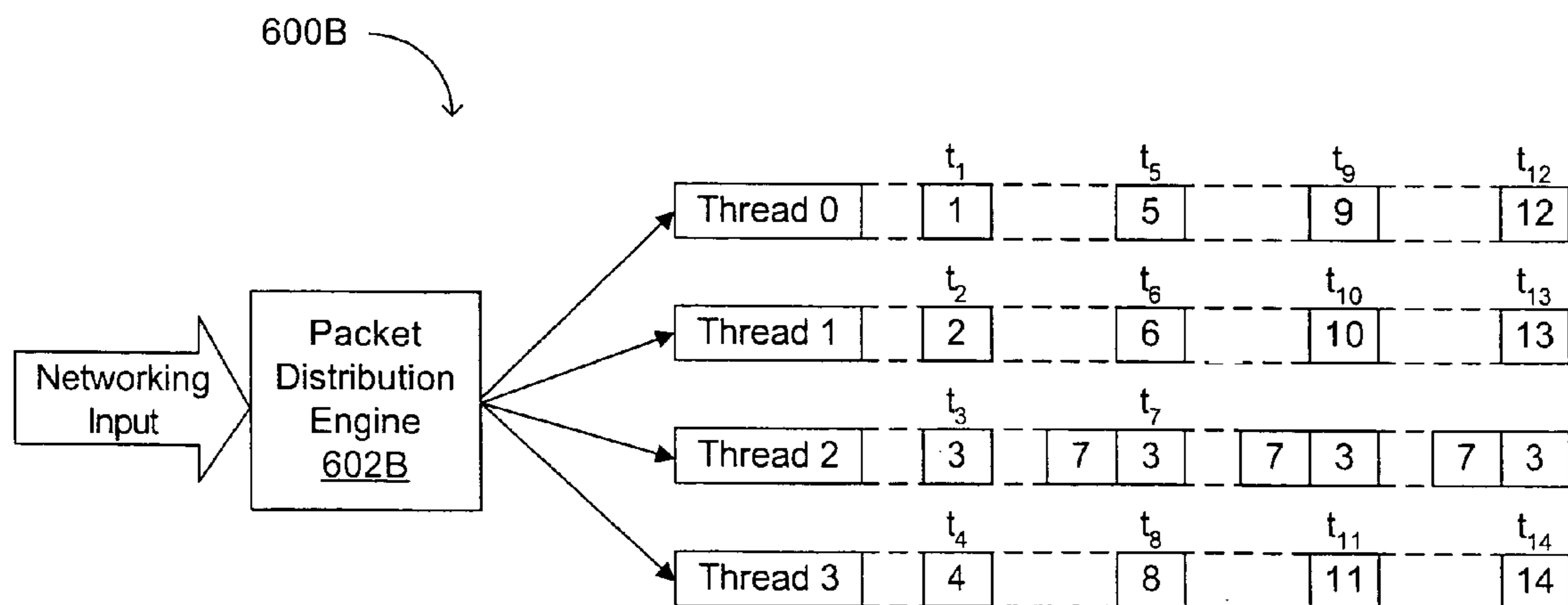
FIG. 6B
