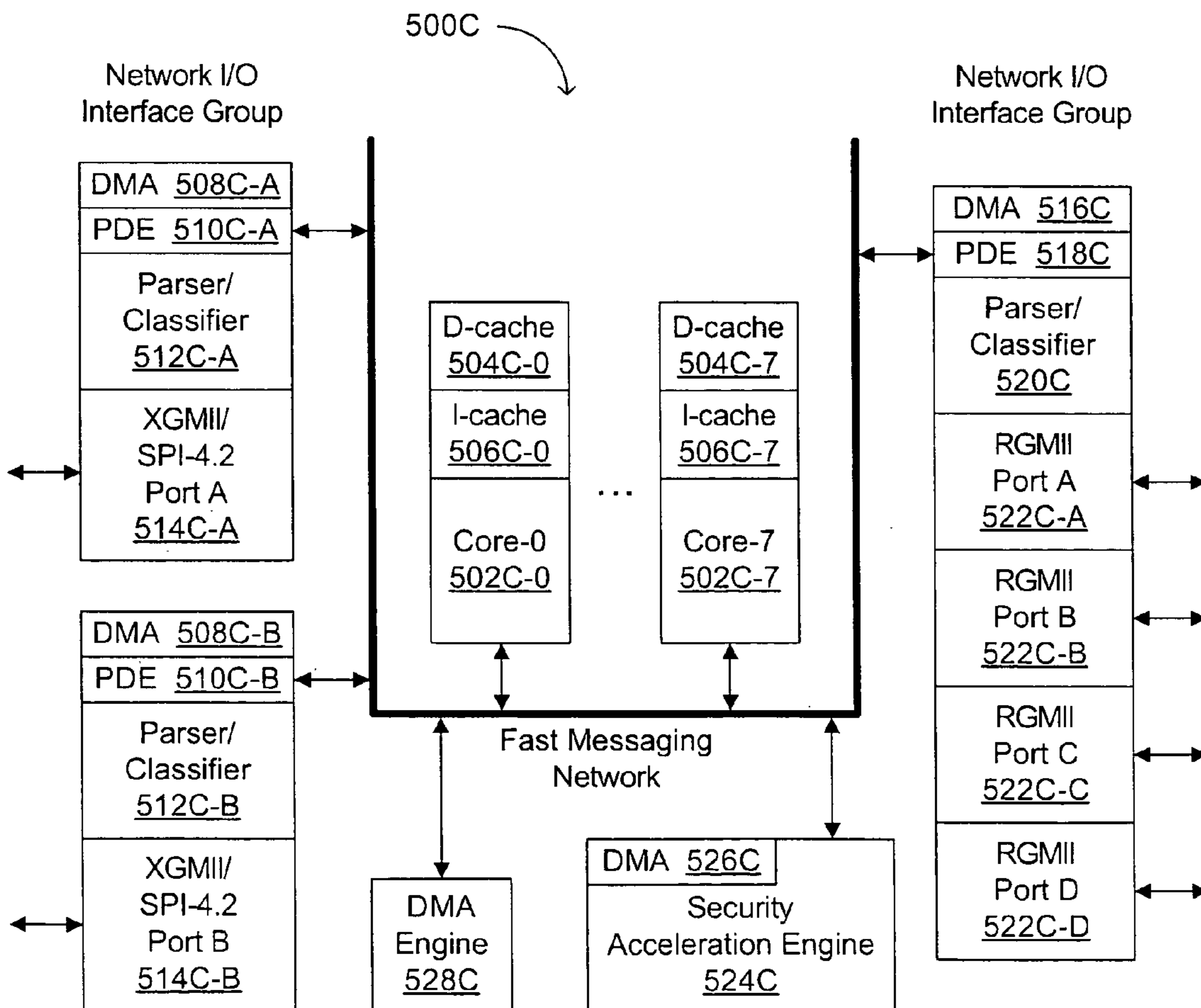
FIG. 5C
