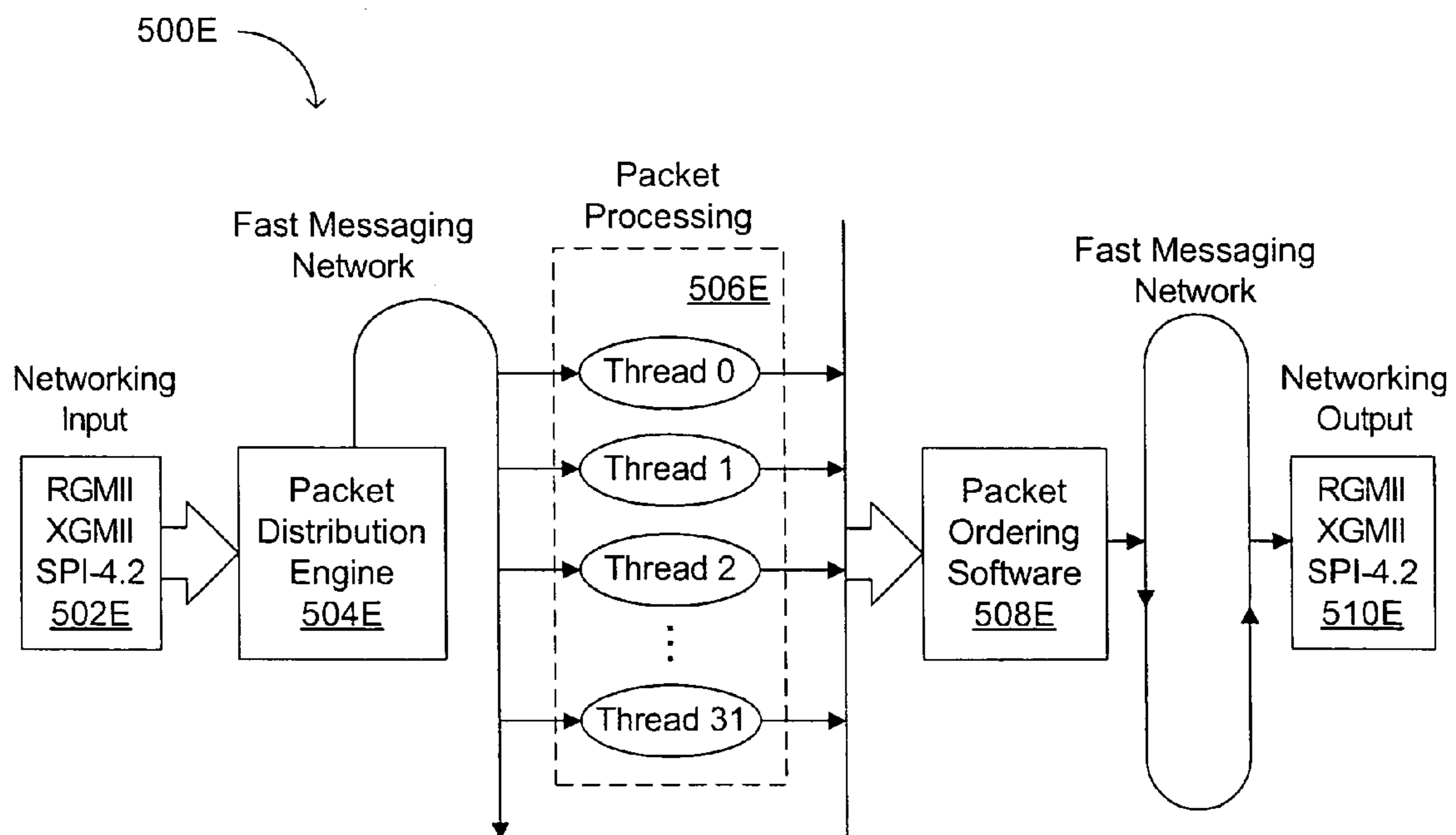
FIG. 5E
