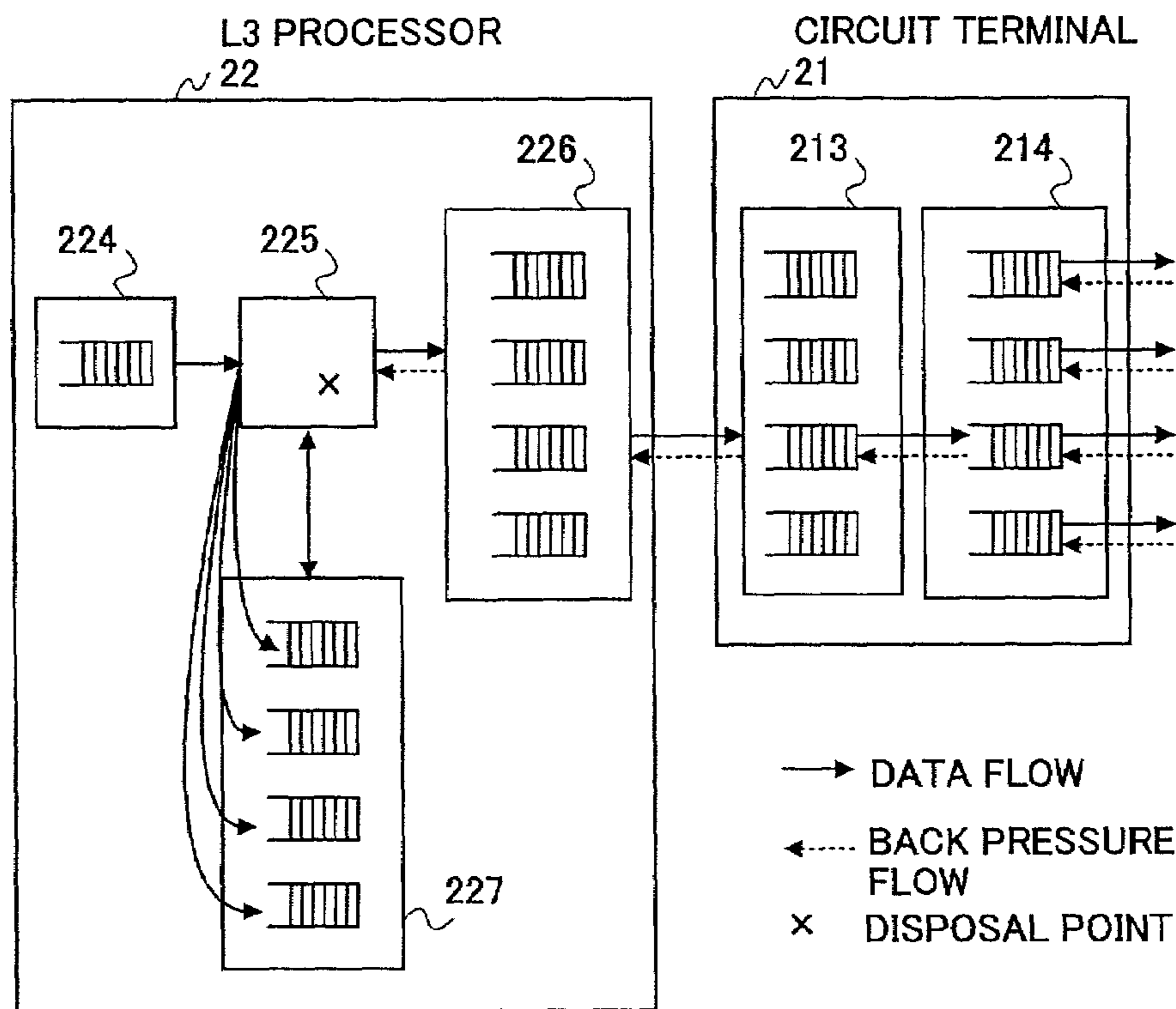
FIG.17A
