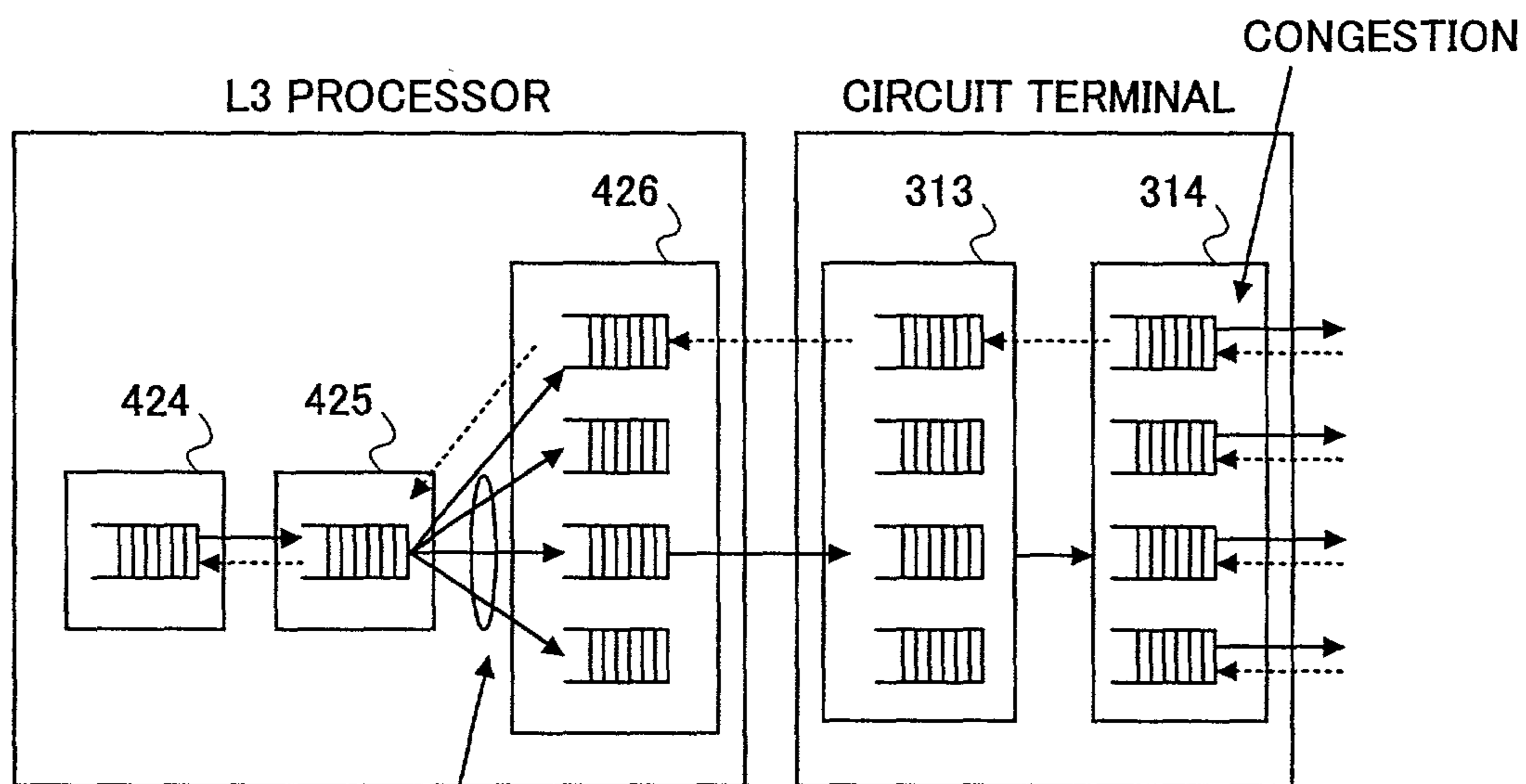
FIG. 16B
