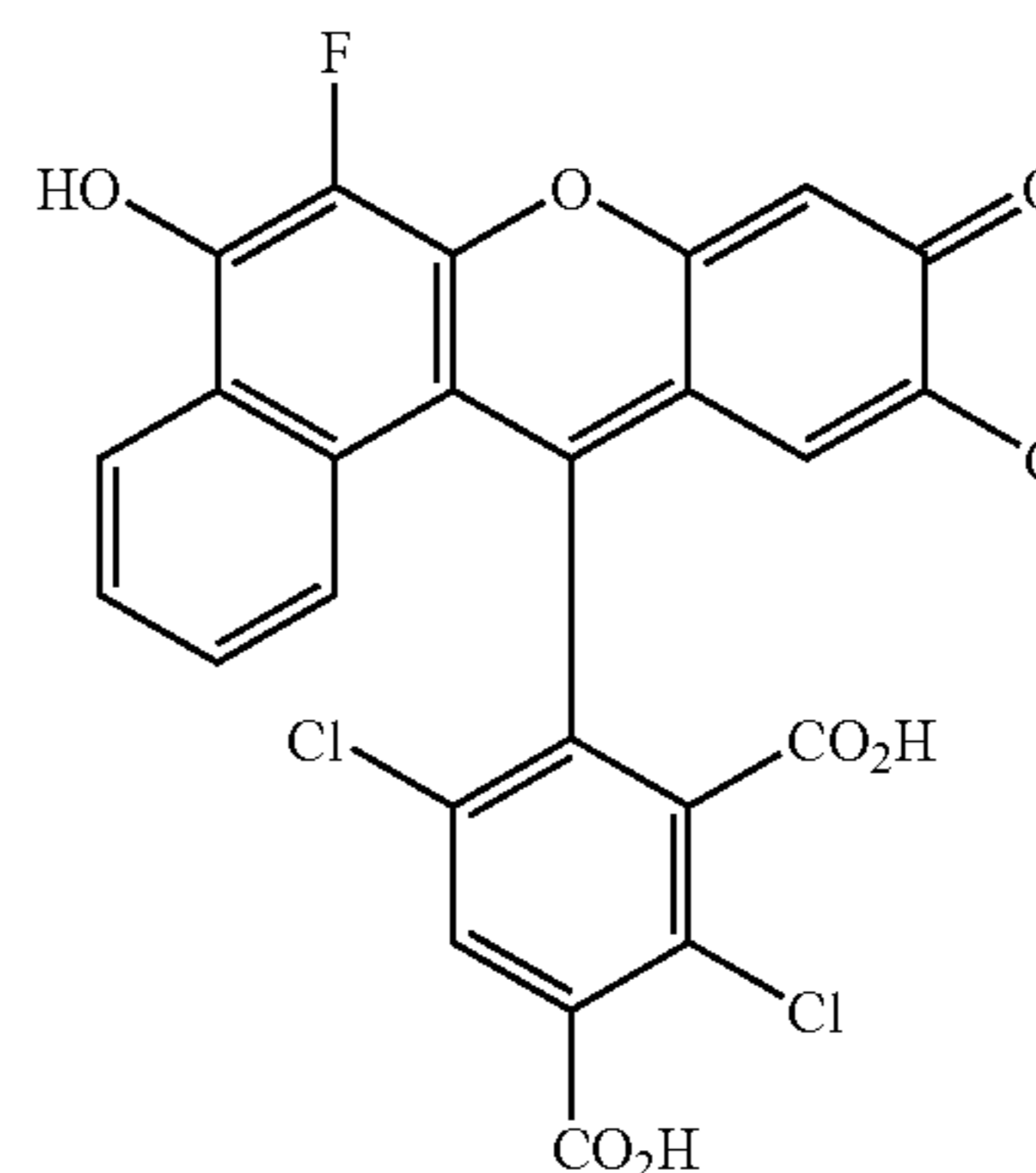
Cl-FLAN
