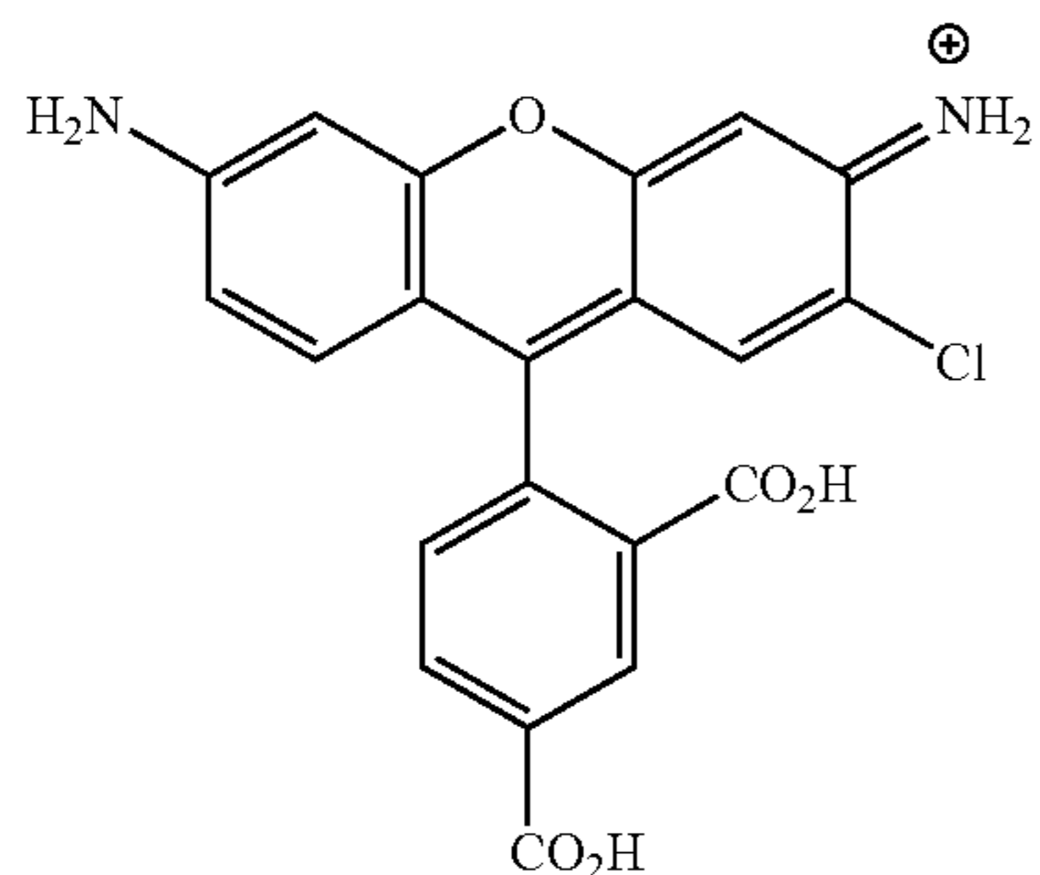
R110
