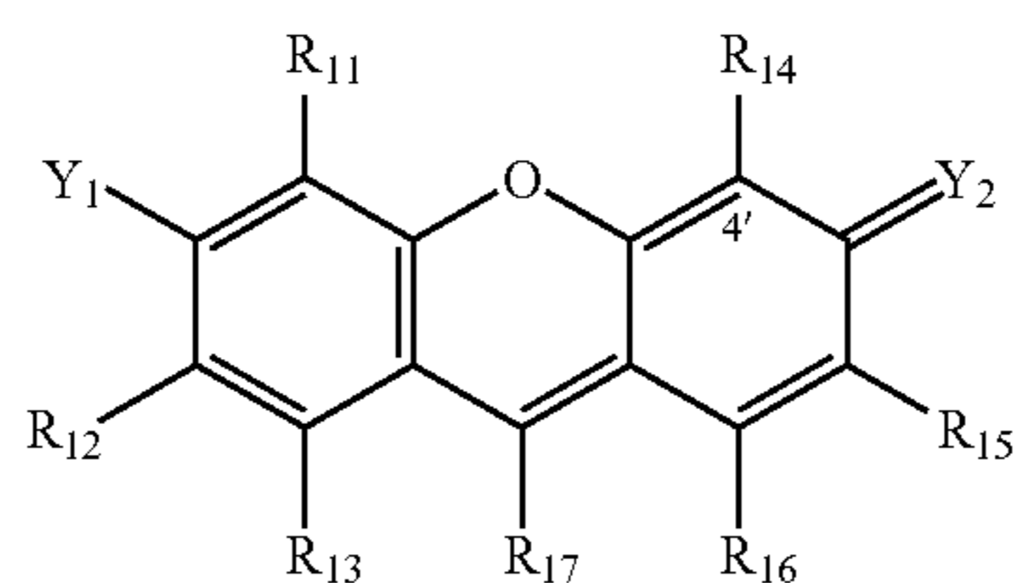
XANTHENE
