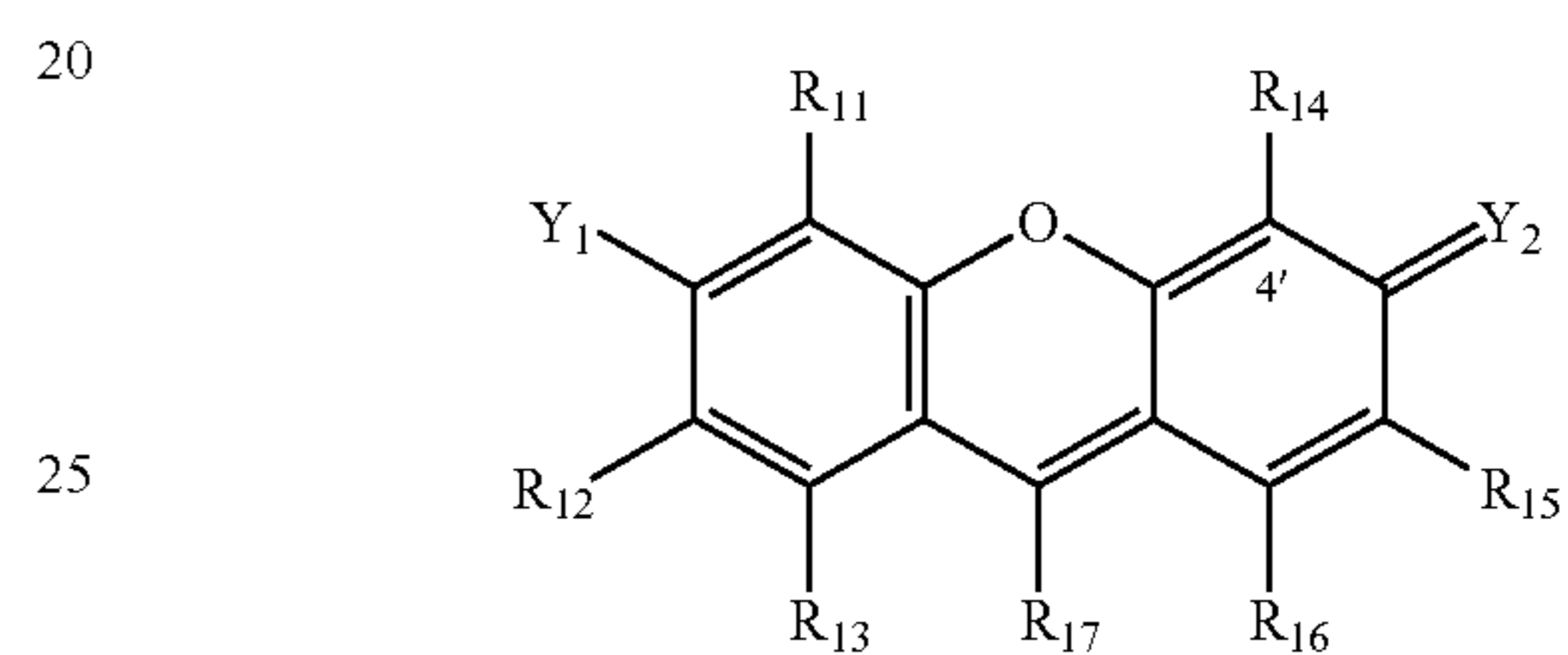
XANTHENE
