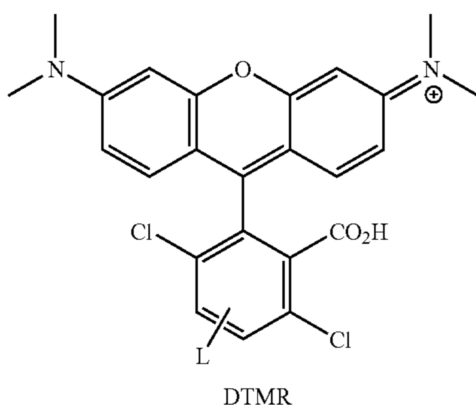
DTMR
