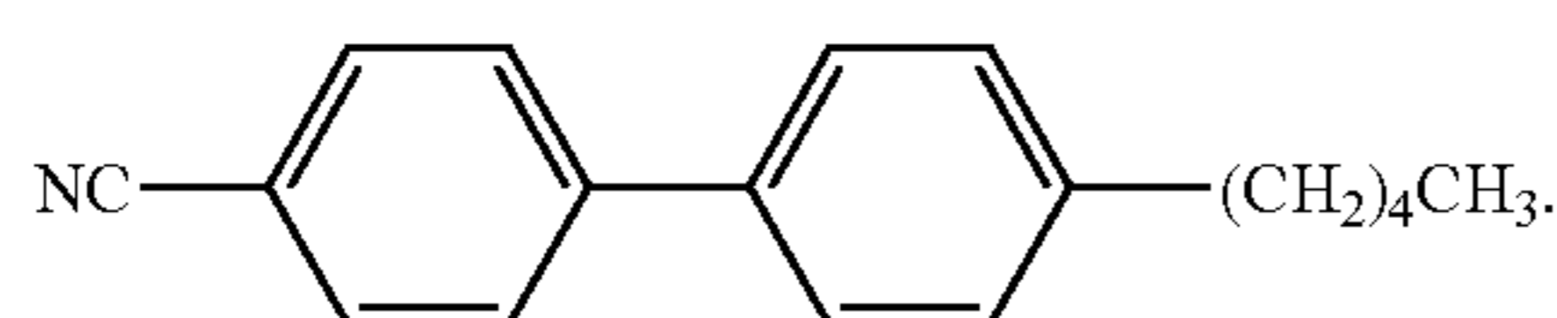
5CB, CAS 40817-08-1
