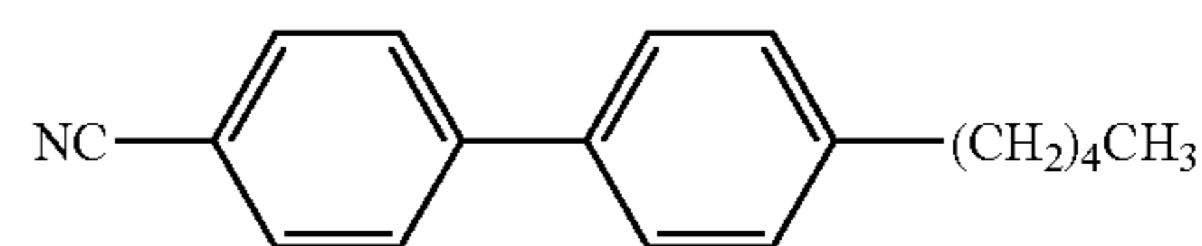
5CB, CAS 40817-08-1
