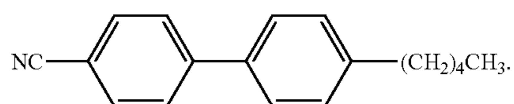
5CB, CAS 40817-08-1
