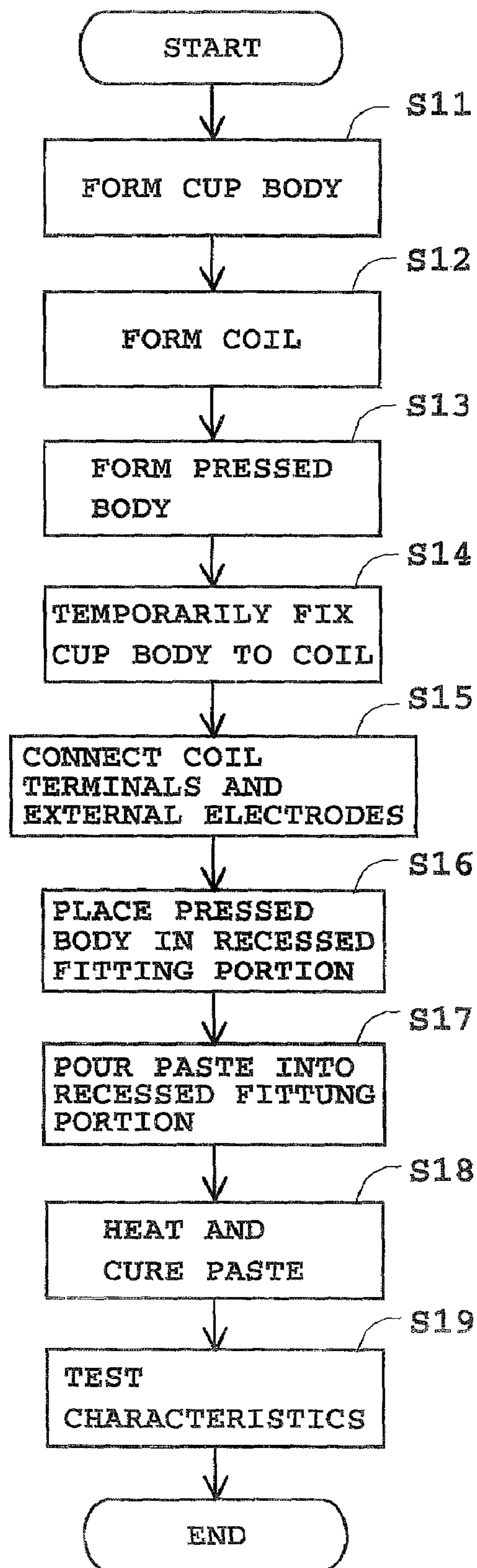
FIG. 19
