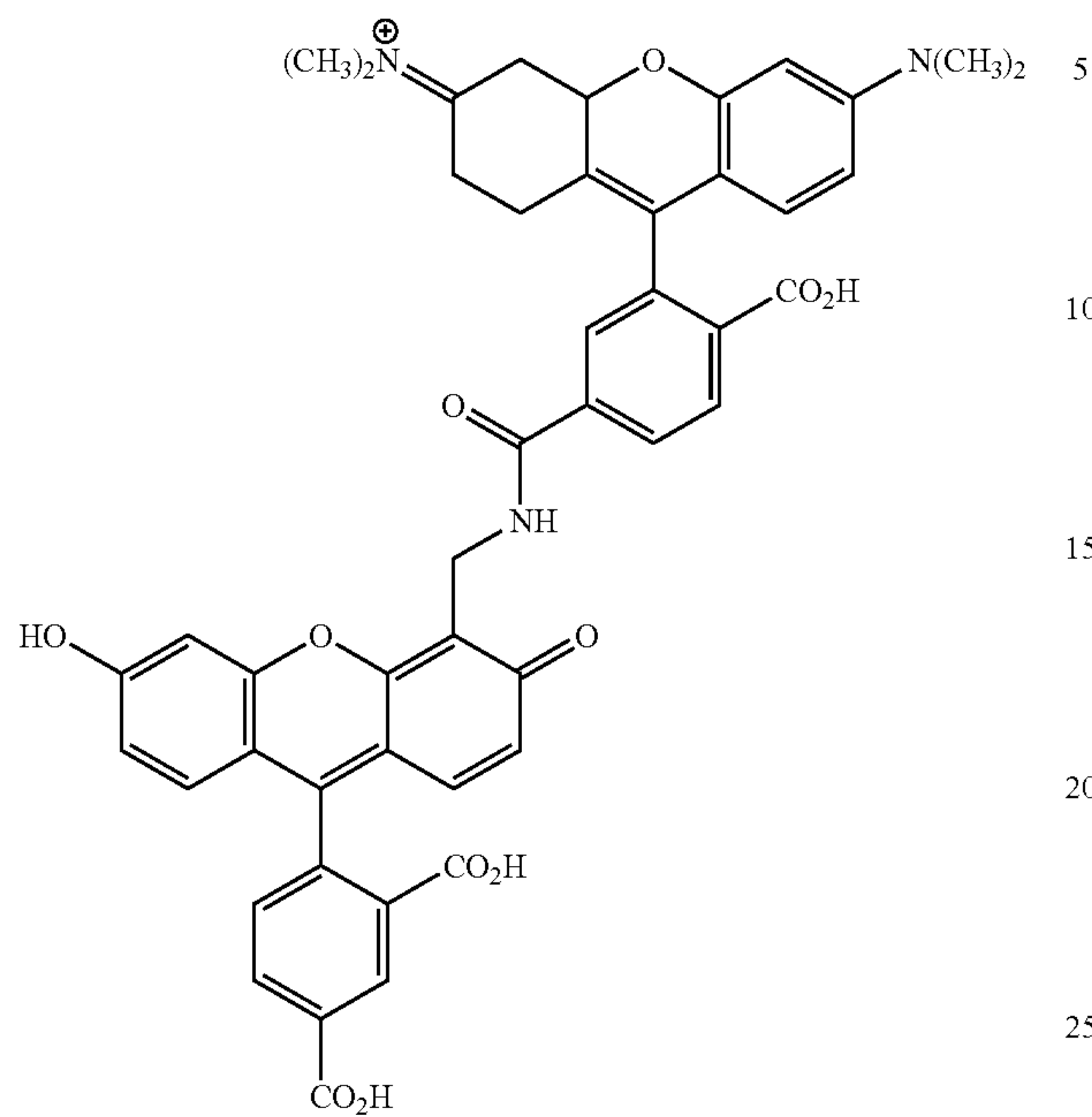
6TMR-CF
