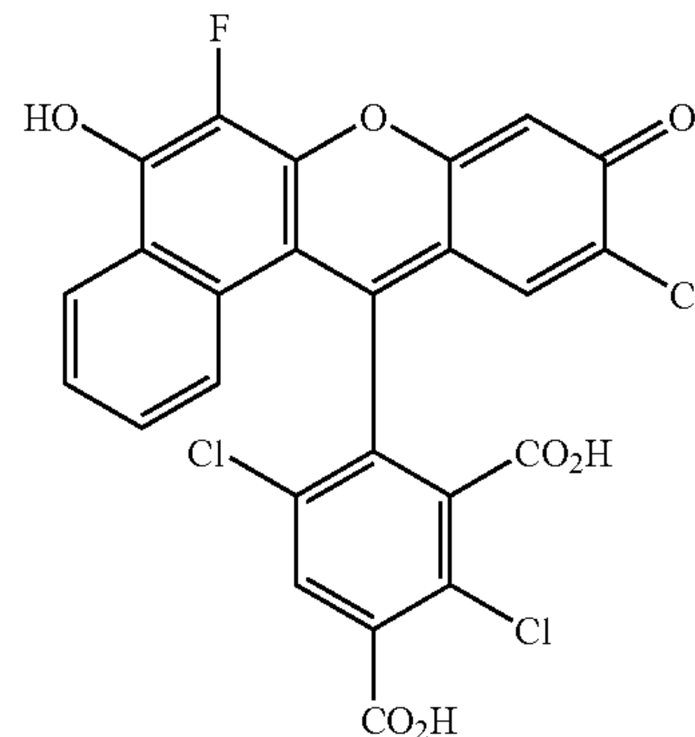
Cl-FLAN
