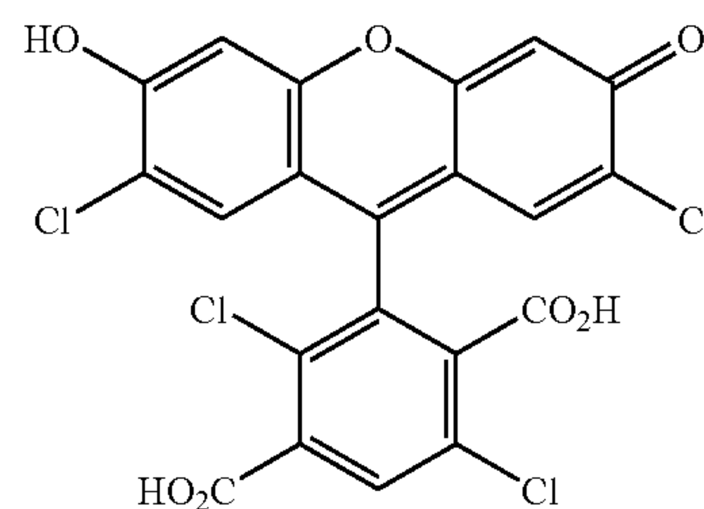
TET
