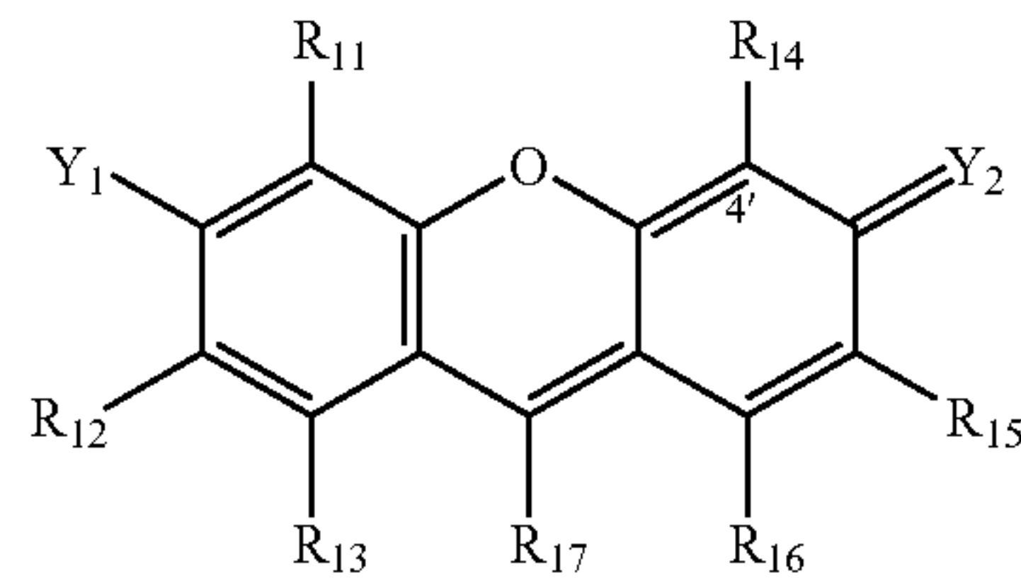
XANTHENE
