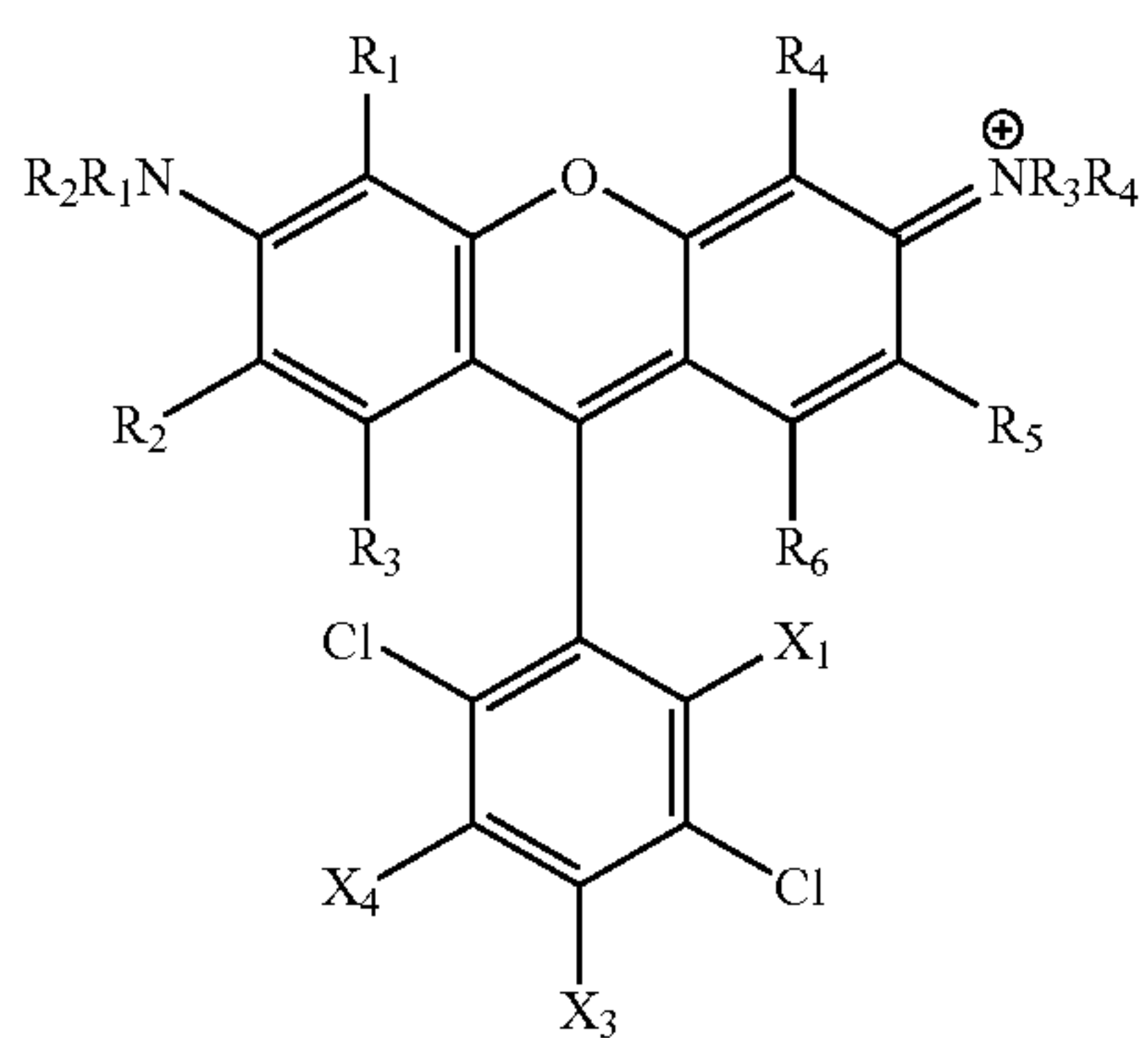
4,7-Dichlororhodamine
