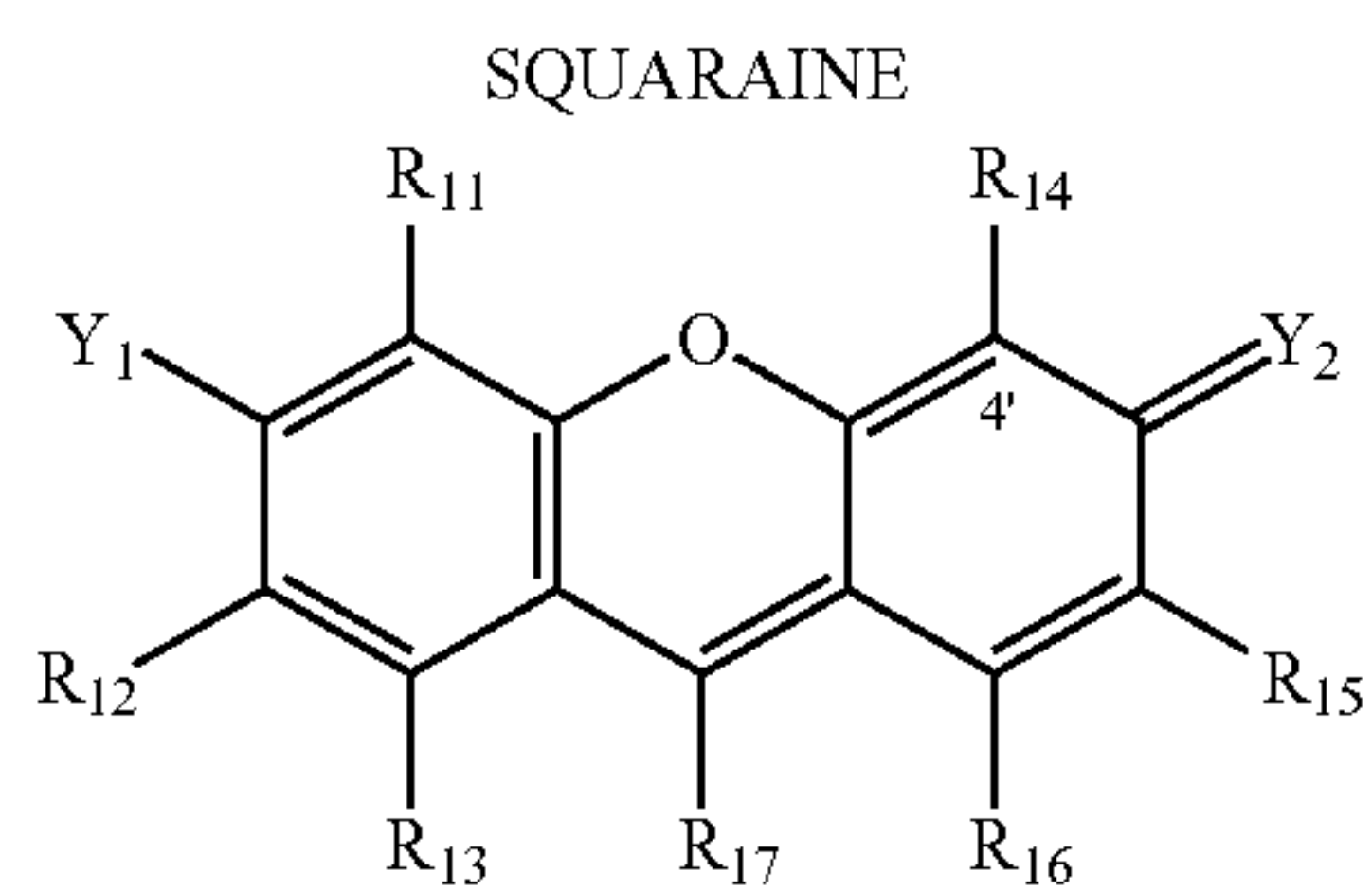
XANTHENE
