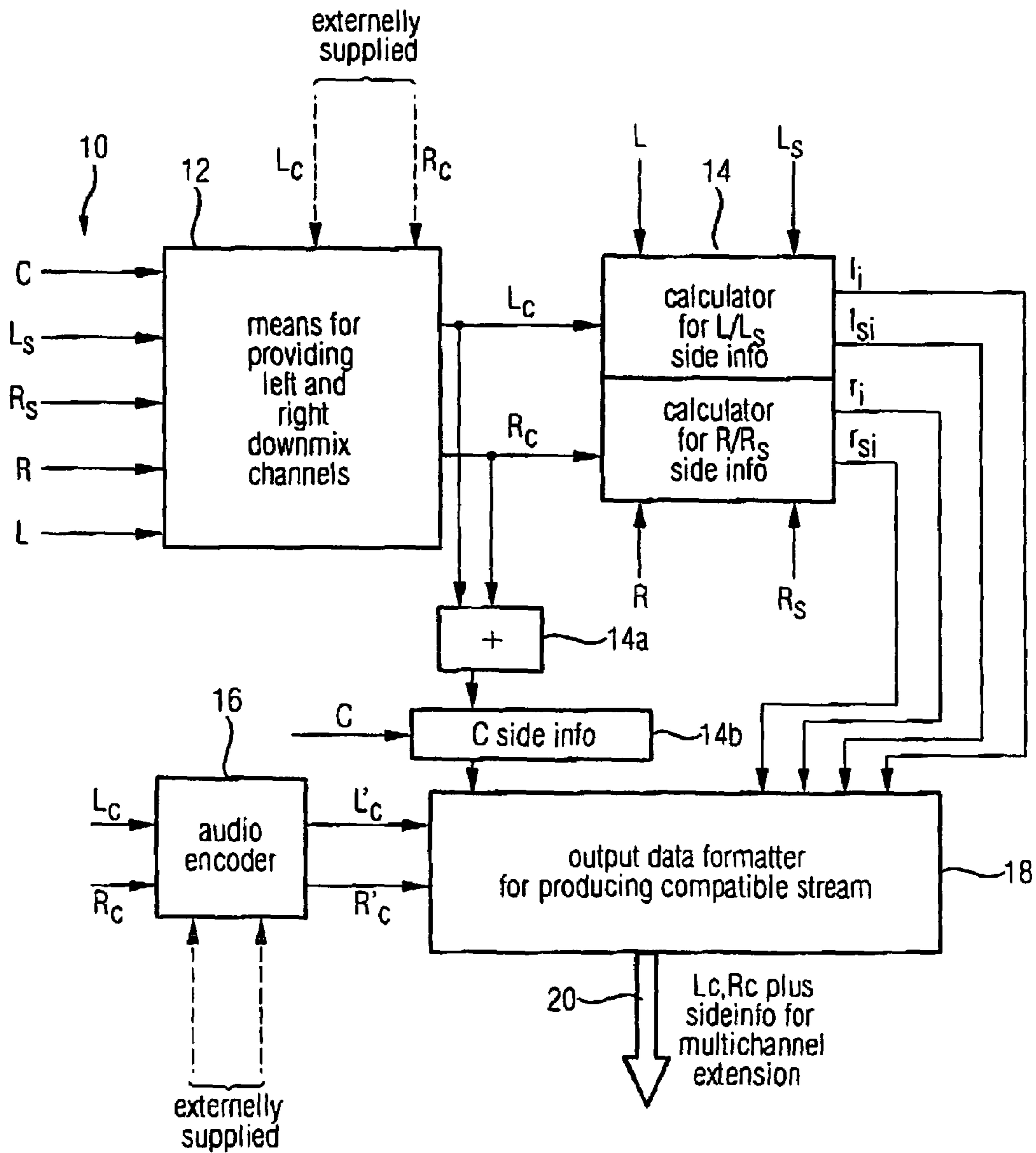
FIG 1 (Encoder)
