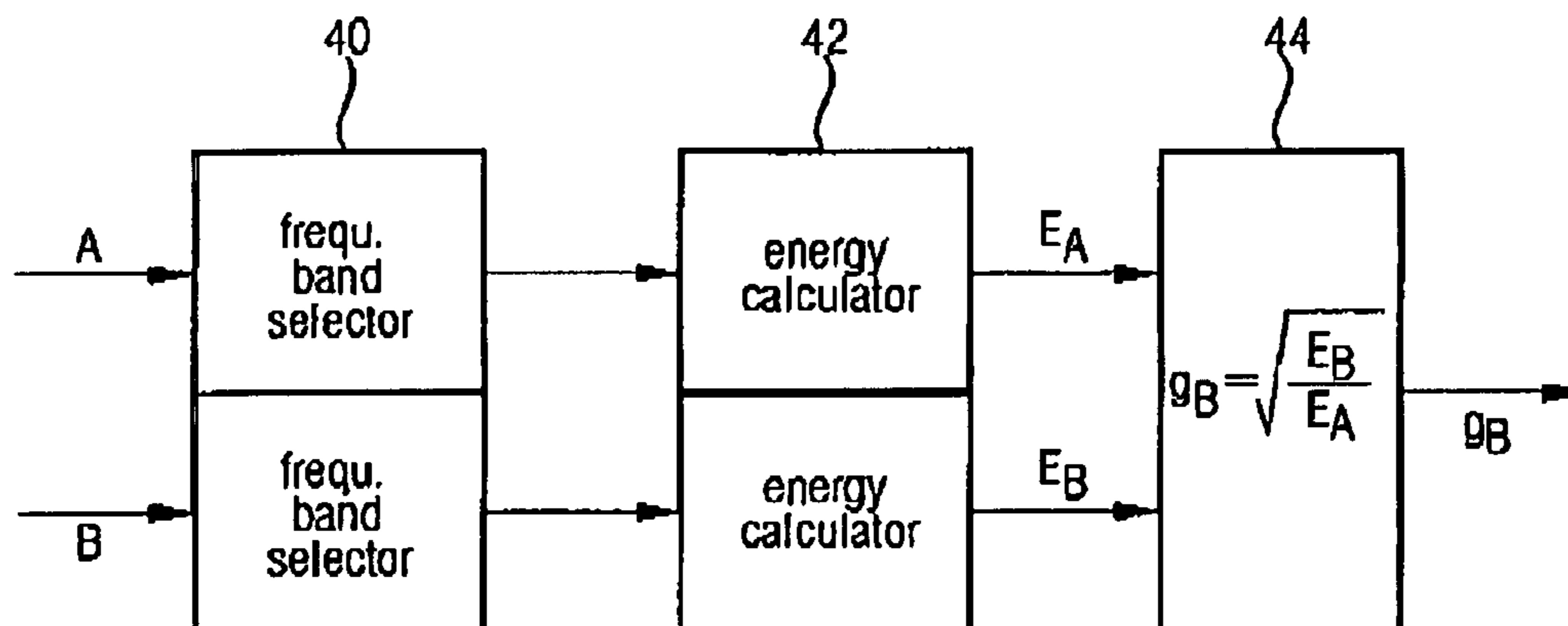
FIG 4 (encoder side)
