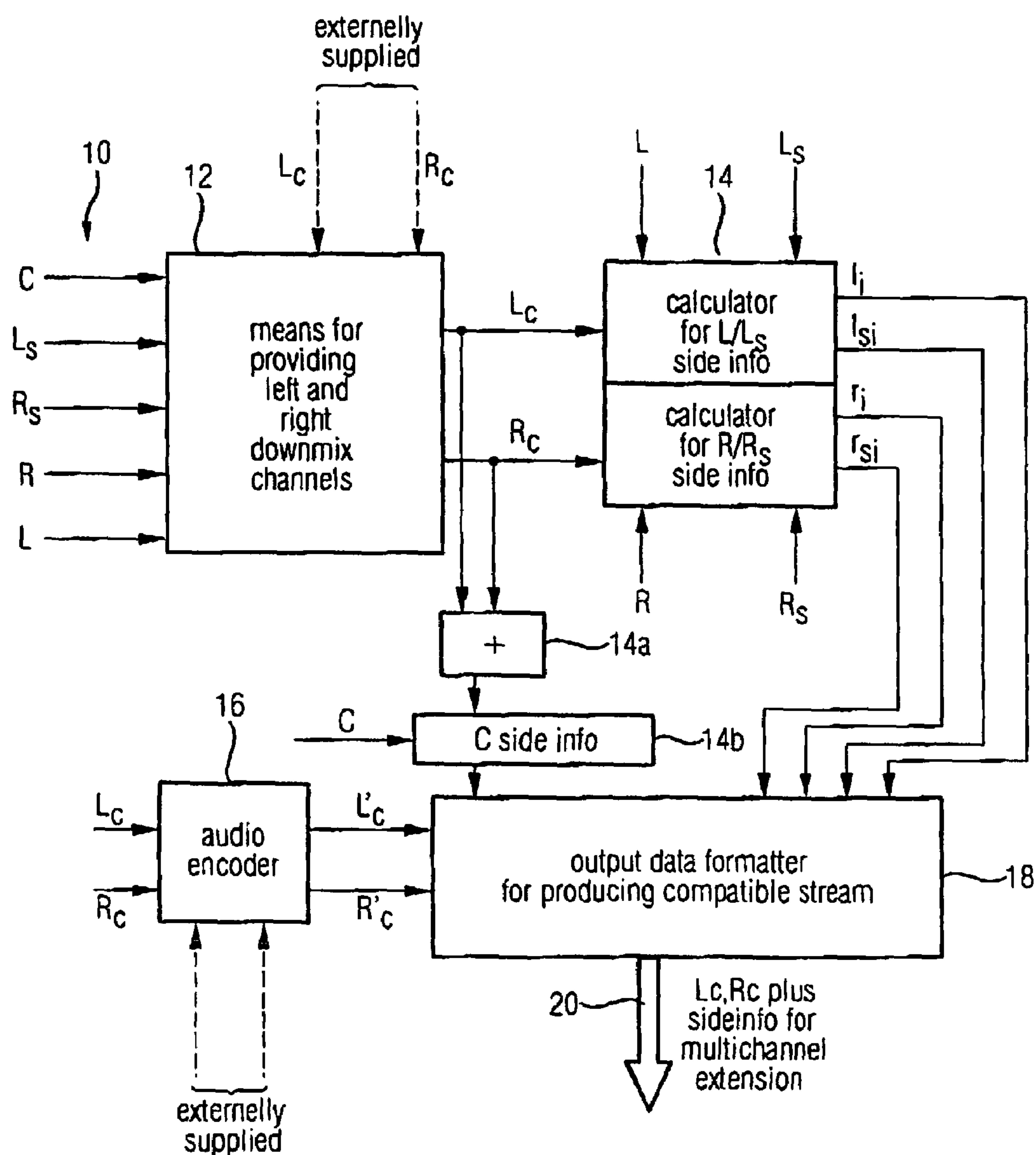
FIG 1 (Encoder)
