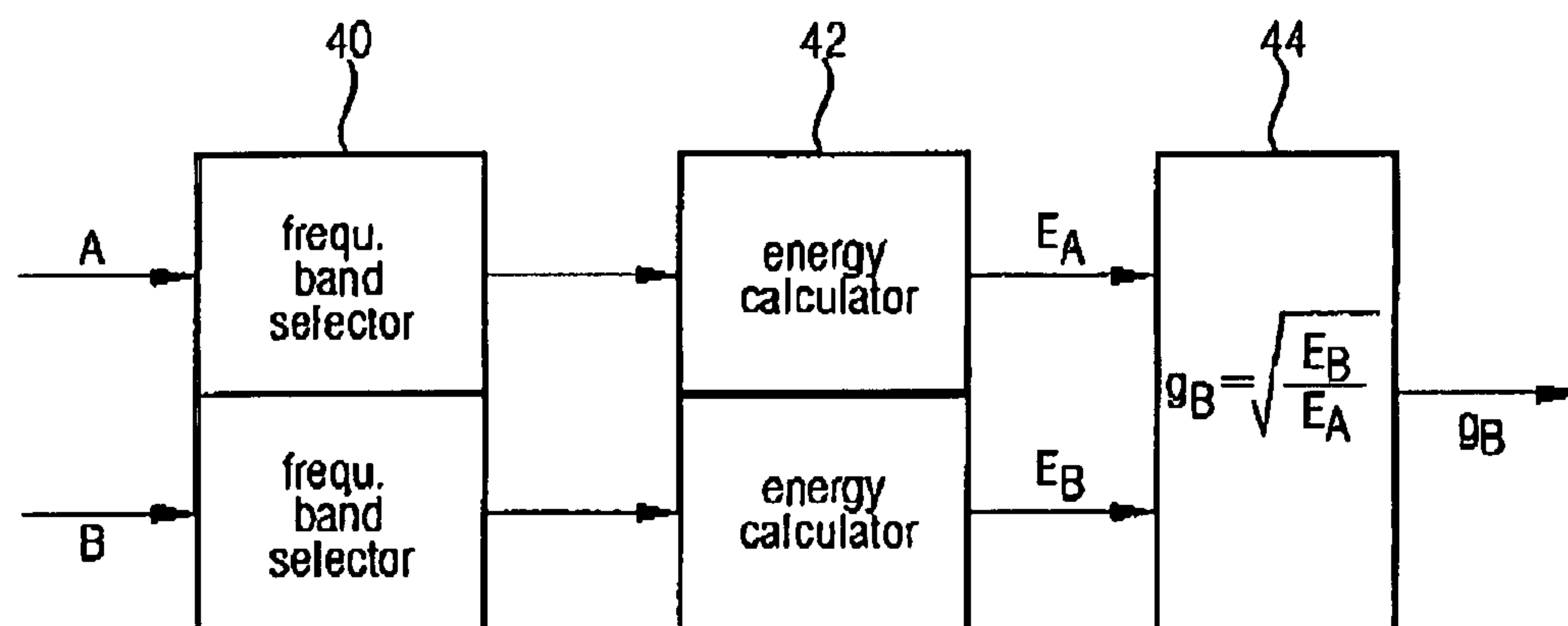
FIG 4 (encoder side)
