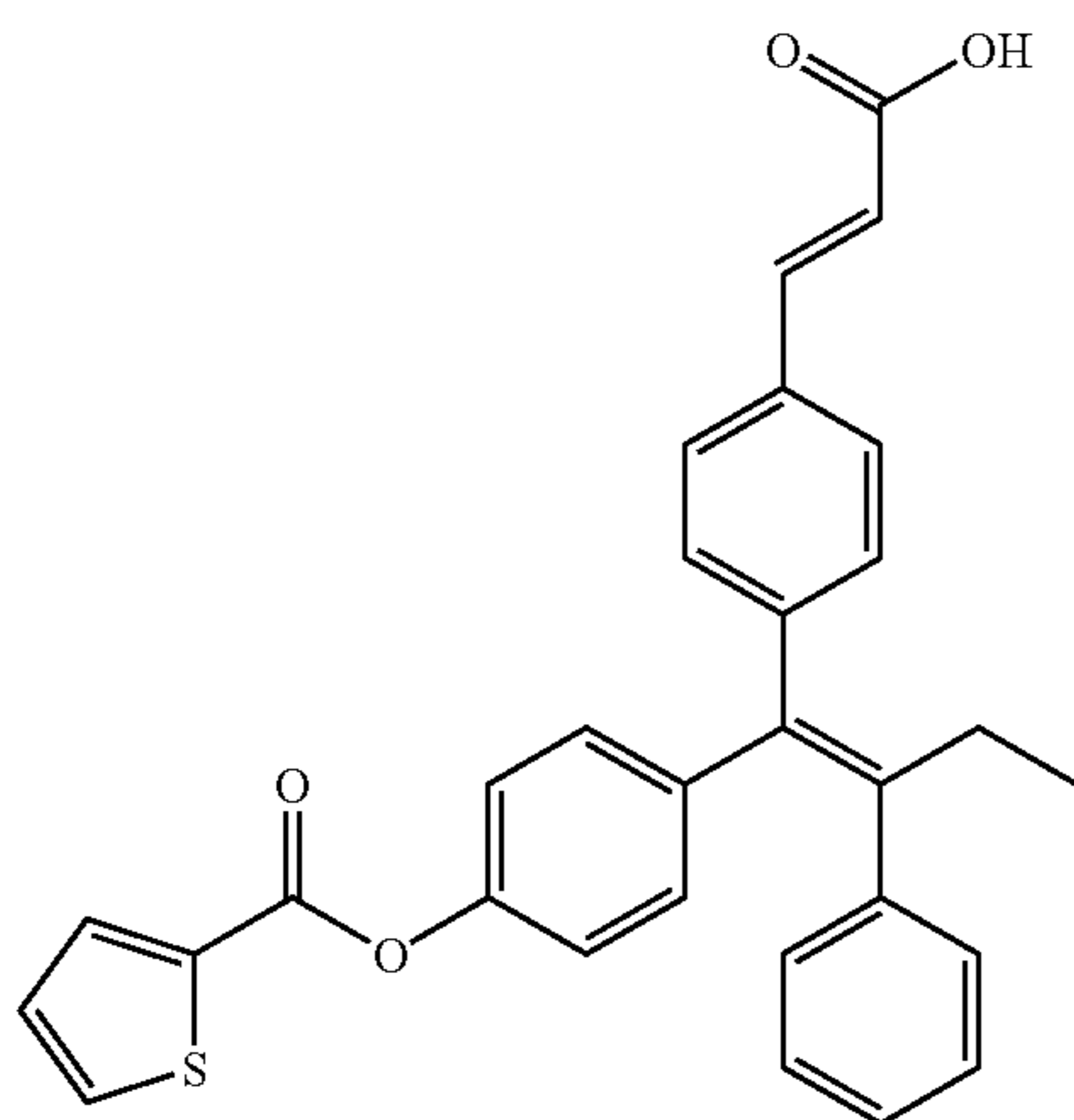
(2E)-3-[4-((1Z)-2-phenyl-1-{4-[(thien-2-ylcarbonyl)oxy]phenyl}but-1-enyl)phenyl]prop-2-enoic acid (25)
