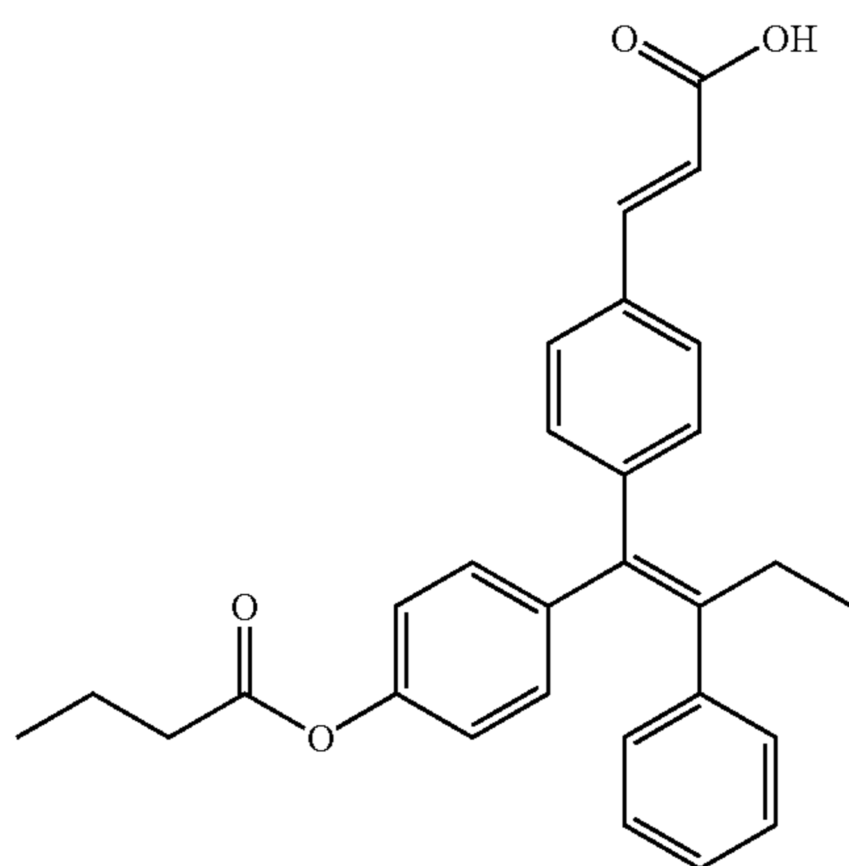
(2E)-3-(4-((1Z)-1-[4-(butyryloxy)phenyl]-2-phenylbut-1-enyl)phenyl)prop-2-enoic acid (21)
