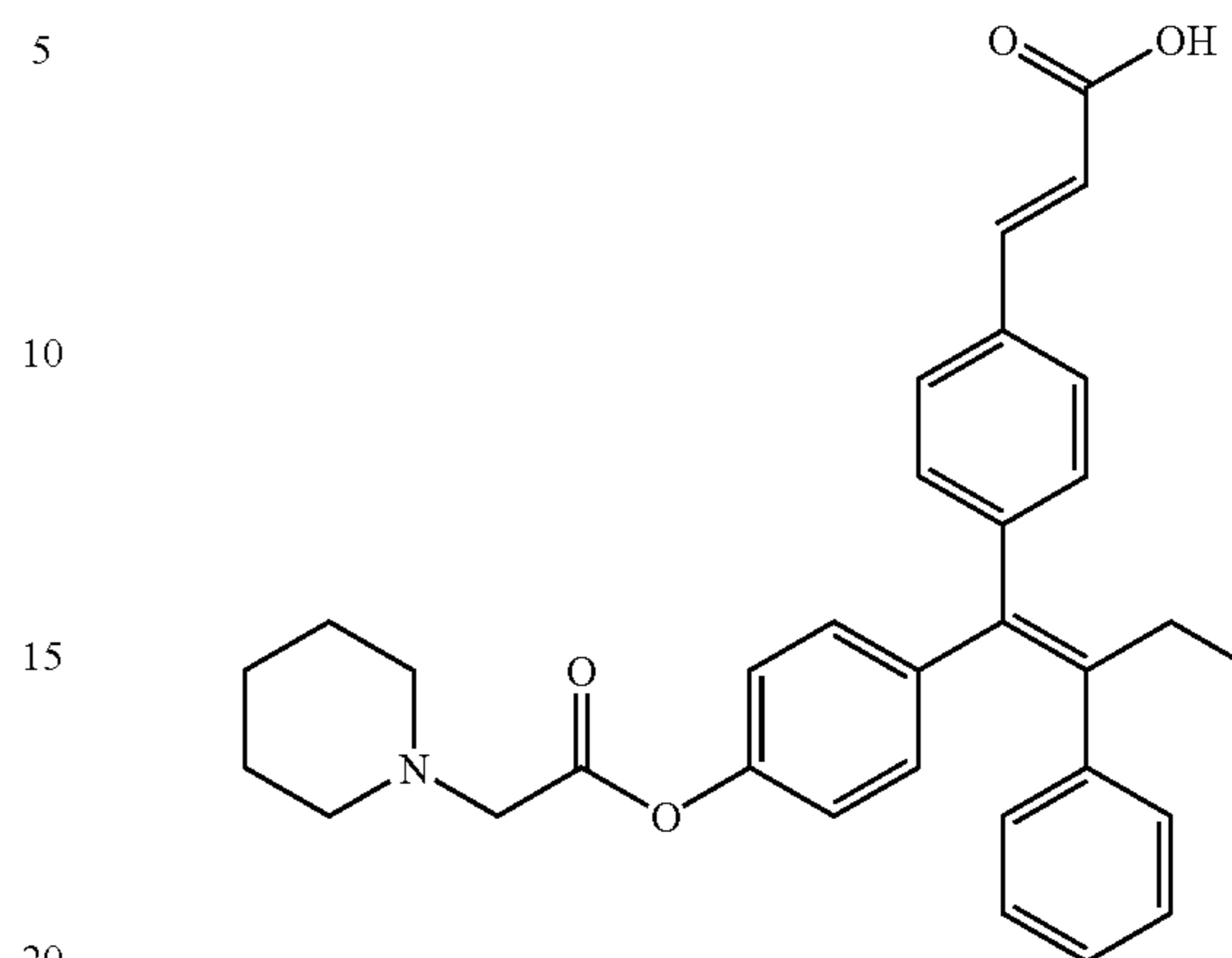
(2E)-3-[4-((1Z)-2-phenyl-1-{4-[(piperidin-1-ylacetyl)oxy]phenyl}but-1-enyl)phenyl]prop-2-enoic acid (33)
