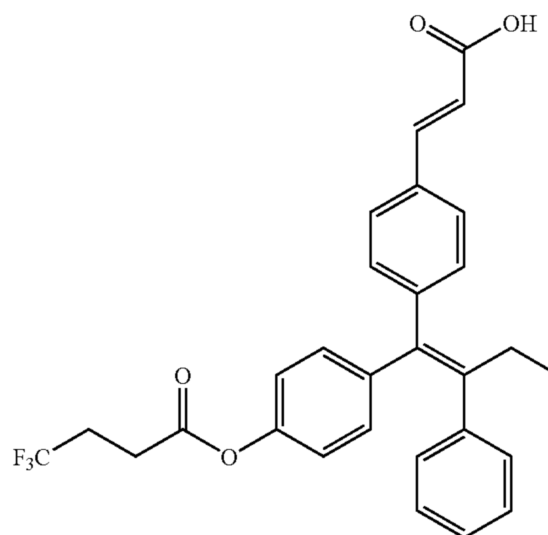
(2E)-3-[4-((1Z)-2-phenyl-1-{4-[(4,4,4-trifluorobutanoyl)oxy]phenyl}but-1-enyl)phenyl]prop-2-enoic acid (27)
