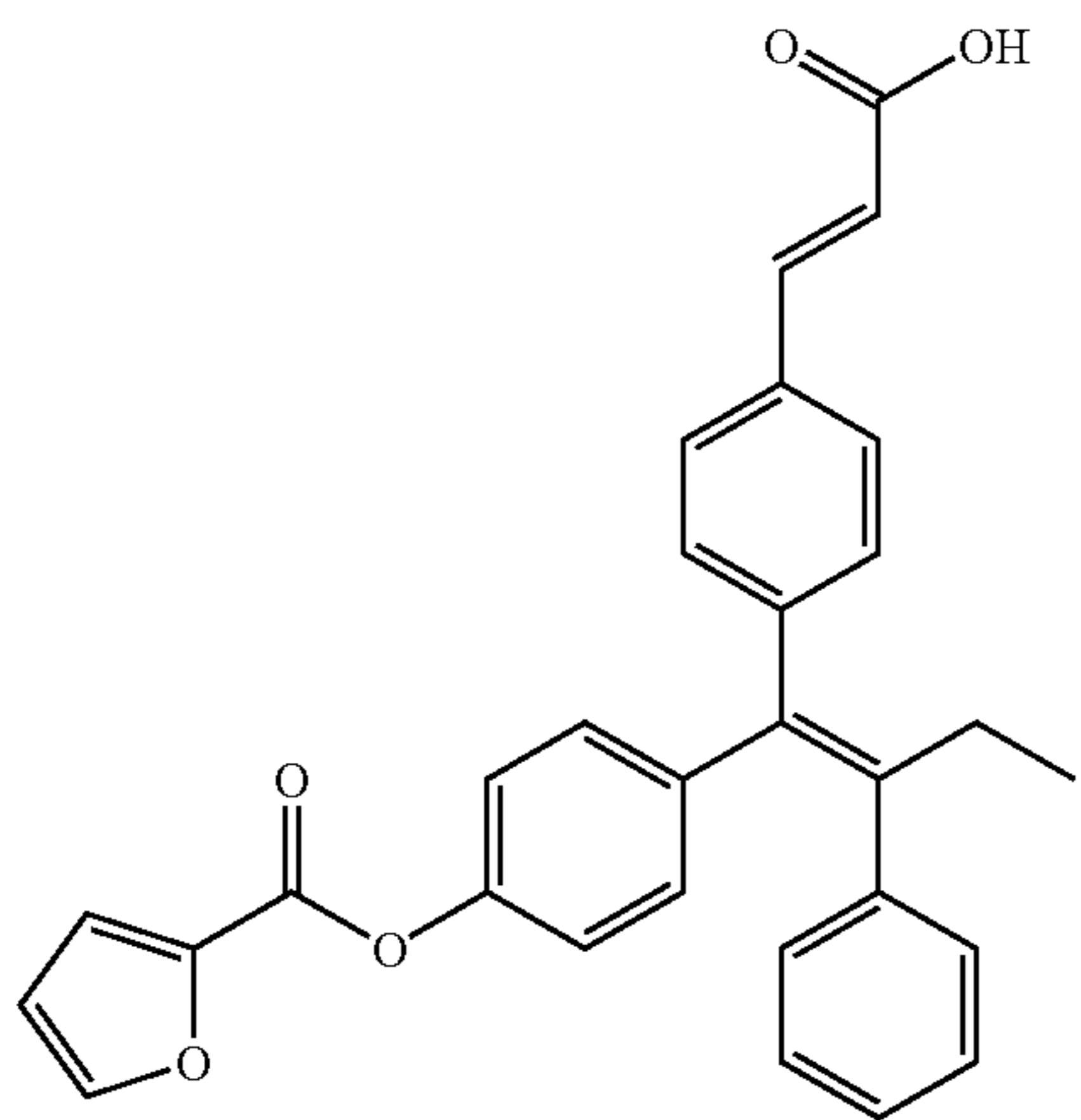
(2E)-3-(4-((1Z)-1-[4-(2-furoyloxy)phenyl]-2-phenyl-1-butenyl)phenyl)-2-propenoic acid (22)
