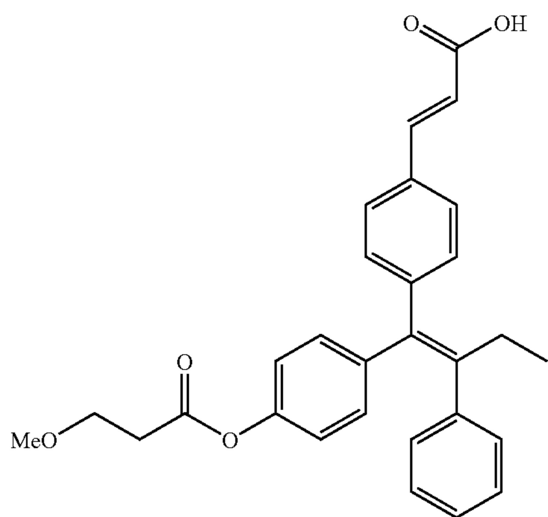
(2E)-3-[4-((1Z)-1-{4-[(methoxyacetyl)oxy]phenyl}-2-phenylbut-1-enyl)phenyl]prop-2-enoic acid (26)
