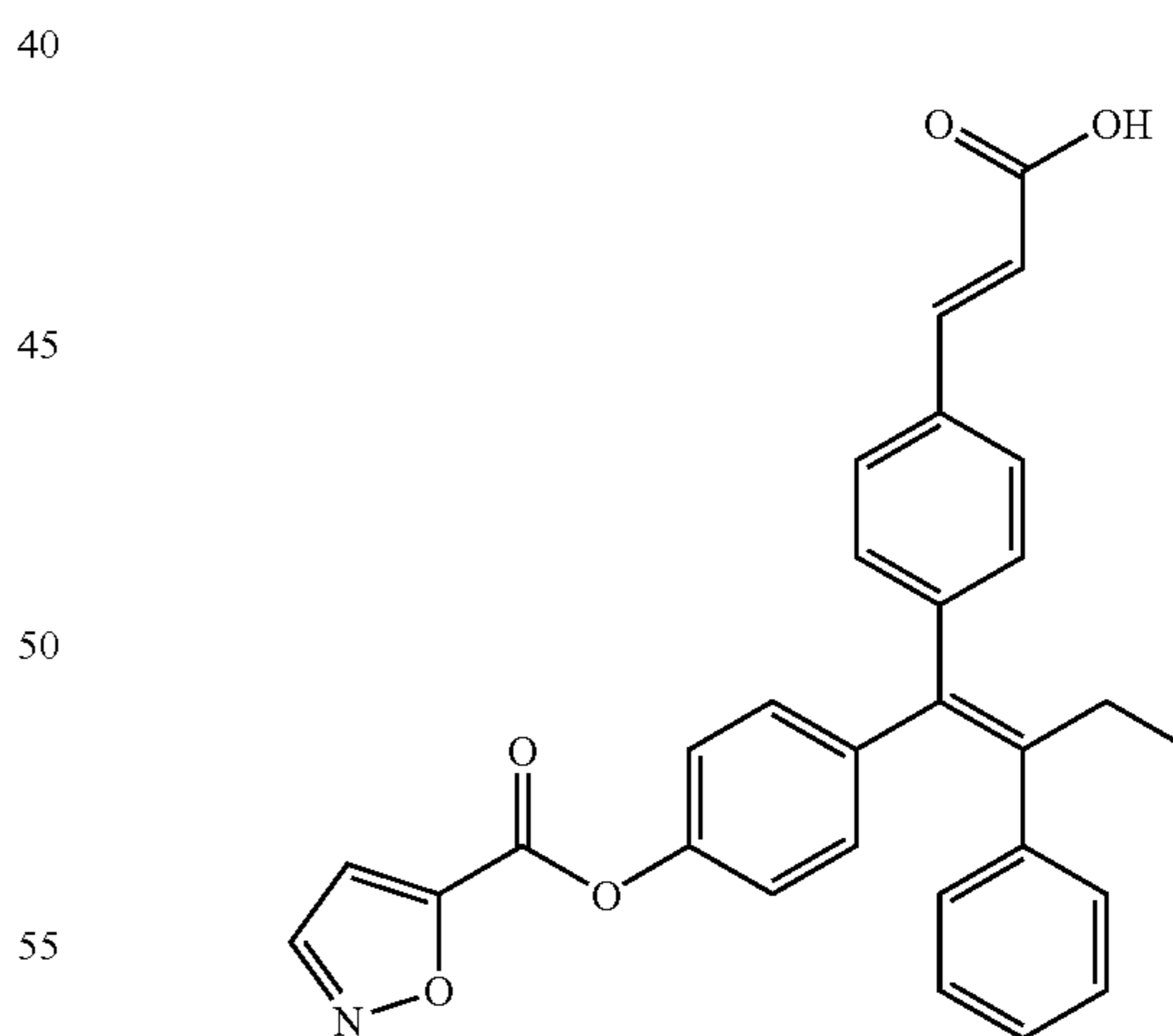
(2E)-3-[4-((1Z)-1-[4-[(5-isoxazolylcarbonyl)oxy]phenyl]-2-phenyl-1-butenyl)phenyl]-2-propenoic acid (24)
