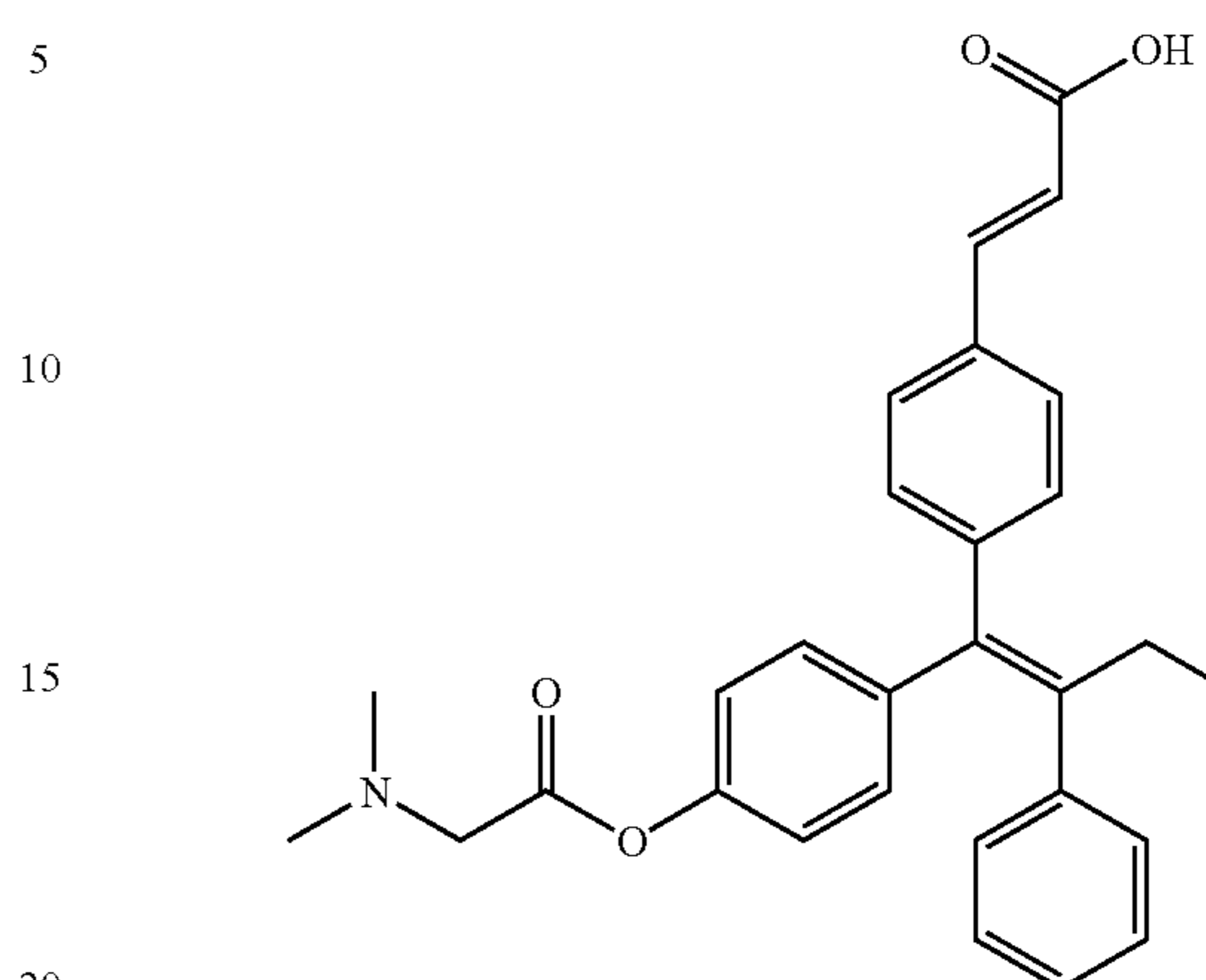
(2E)-3-[4-((1Z)-1-[4-[(N,N-dimethylglycyl)oxy]phenyl]-2-phenylbut-1-enyl)phenyl]prop-2-enoic acid (23)
