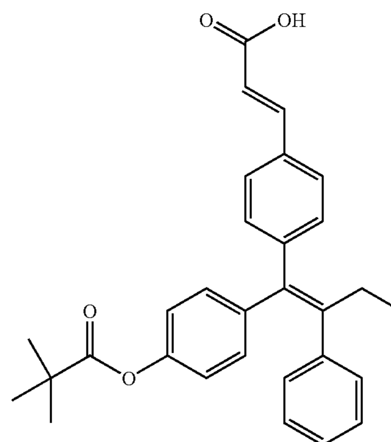
(2E)-3-[4-((1Z)-1-{4-[(2,2-dimethylpropanoyl)oxy]phenyl}-2-phenylbut-1-enyl)phenyl]prop-2-enoic acid (28)
