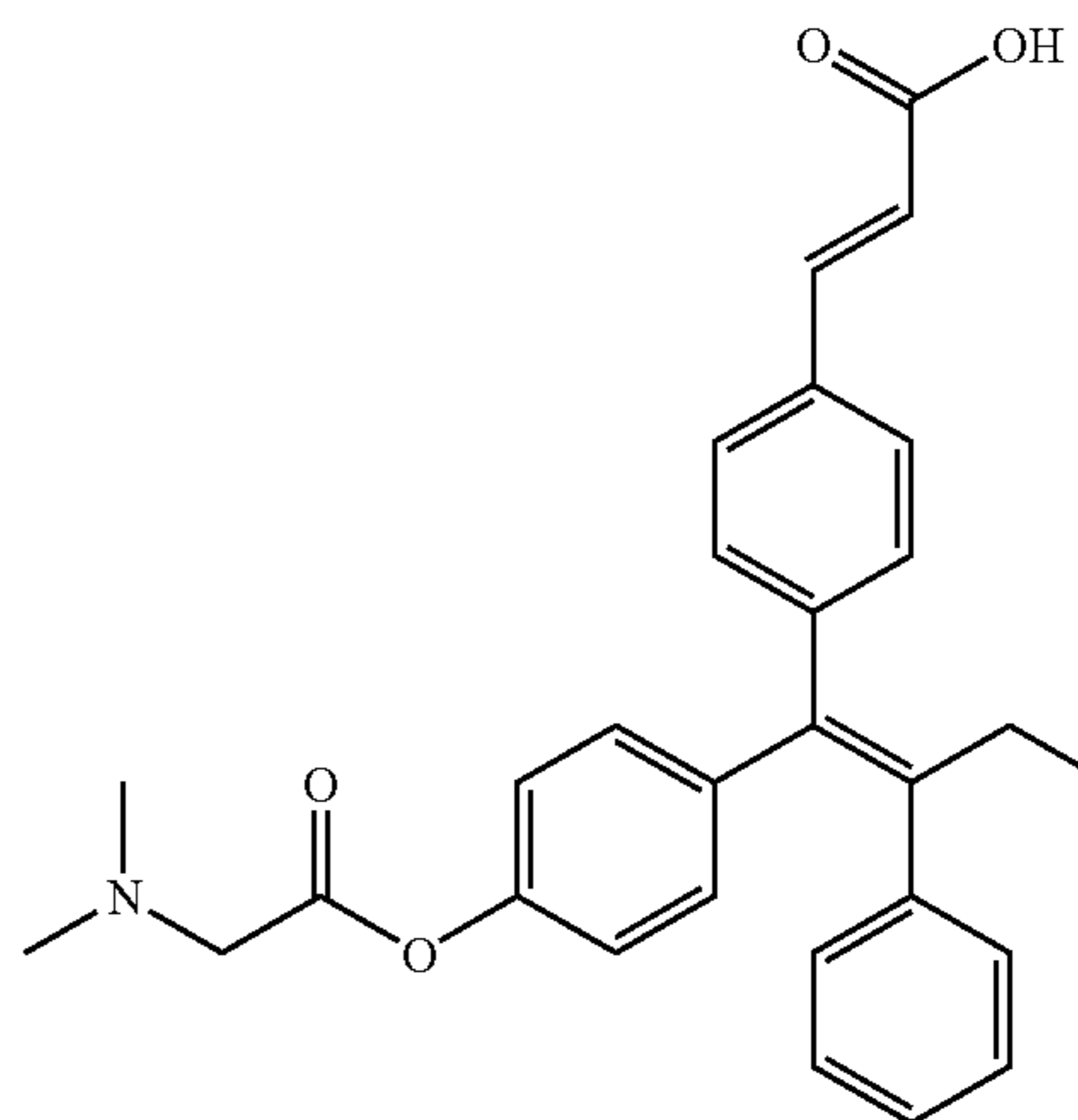
(2E)-3-[4-((1Z)-1-{4-[(N,N-dimethylglycyl)oxy]phenyl}-2-phenylbut-1-enyl)phenyl]prop-2-enoic acid (23)
