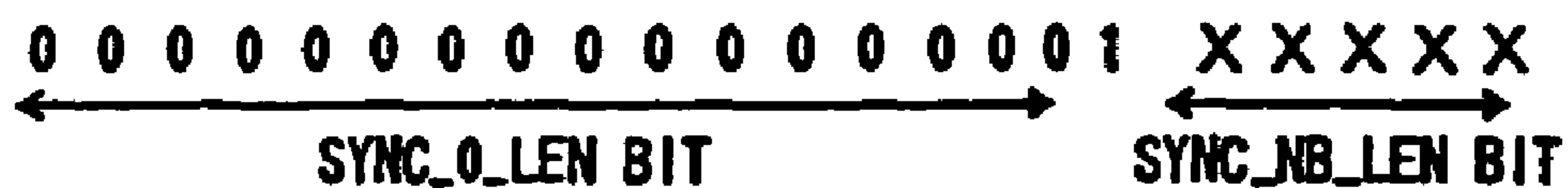
FIG. 6
