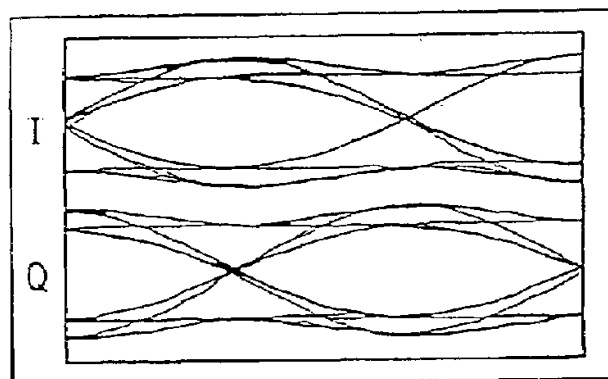
FQPSK-B MEAS.
