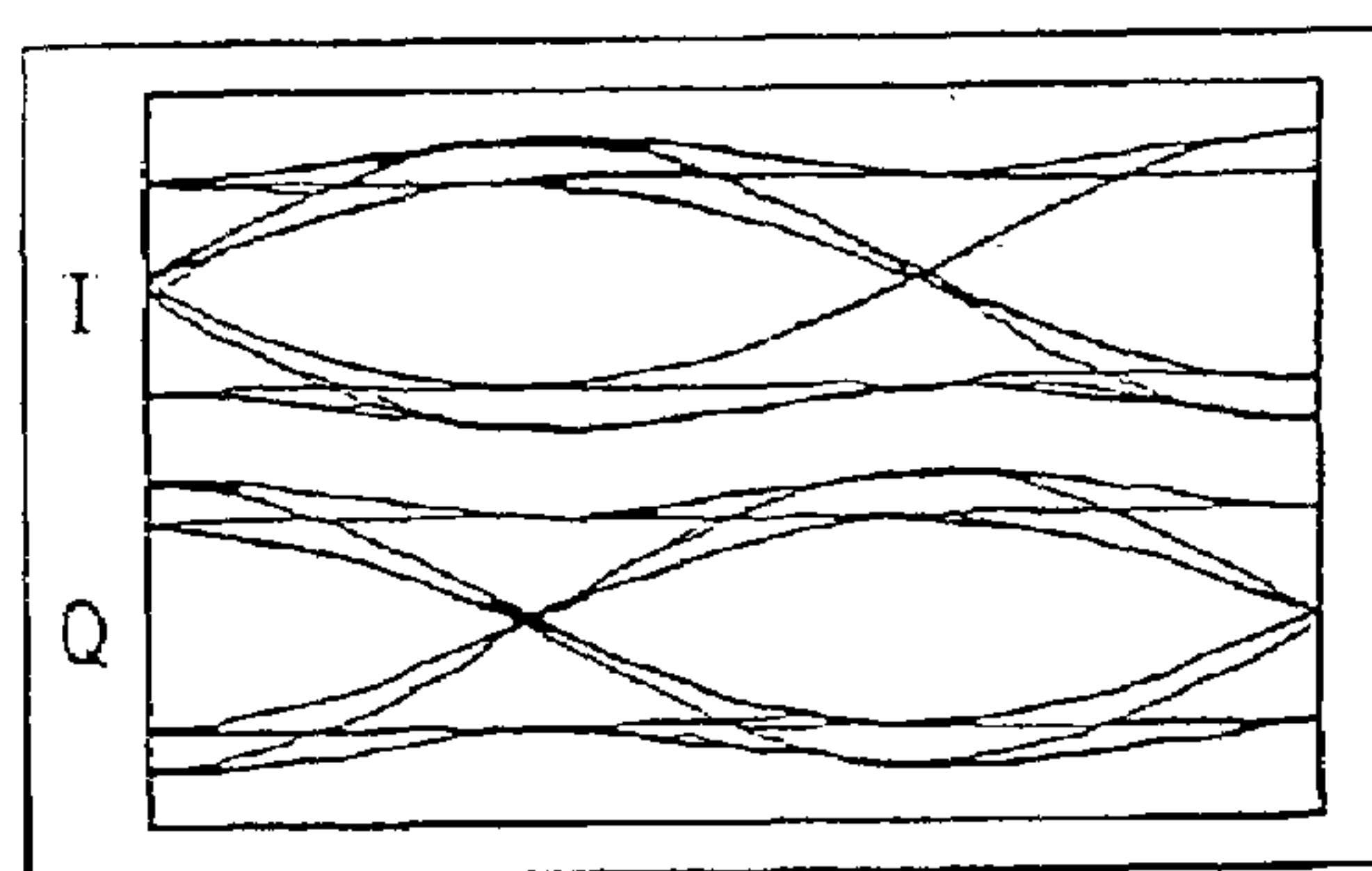
FQPSK-B MEAS.
