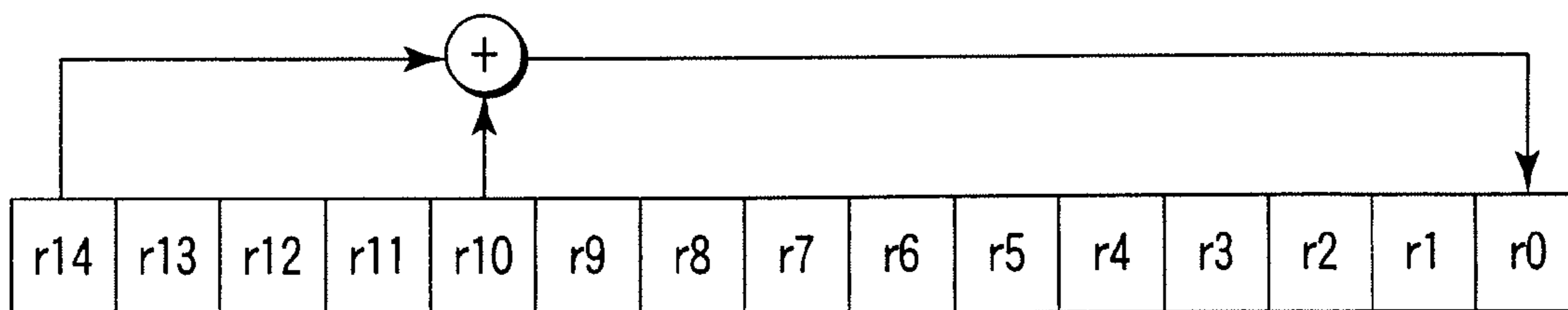
Feedback shift register
