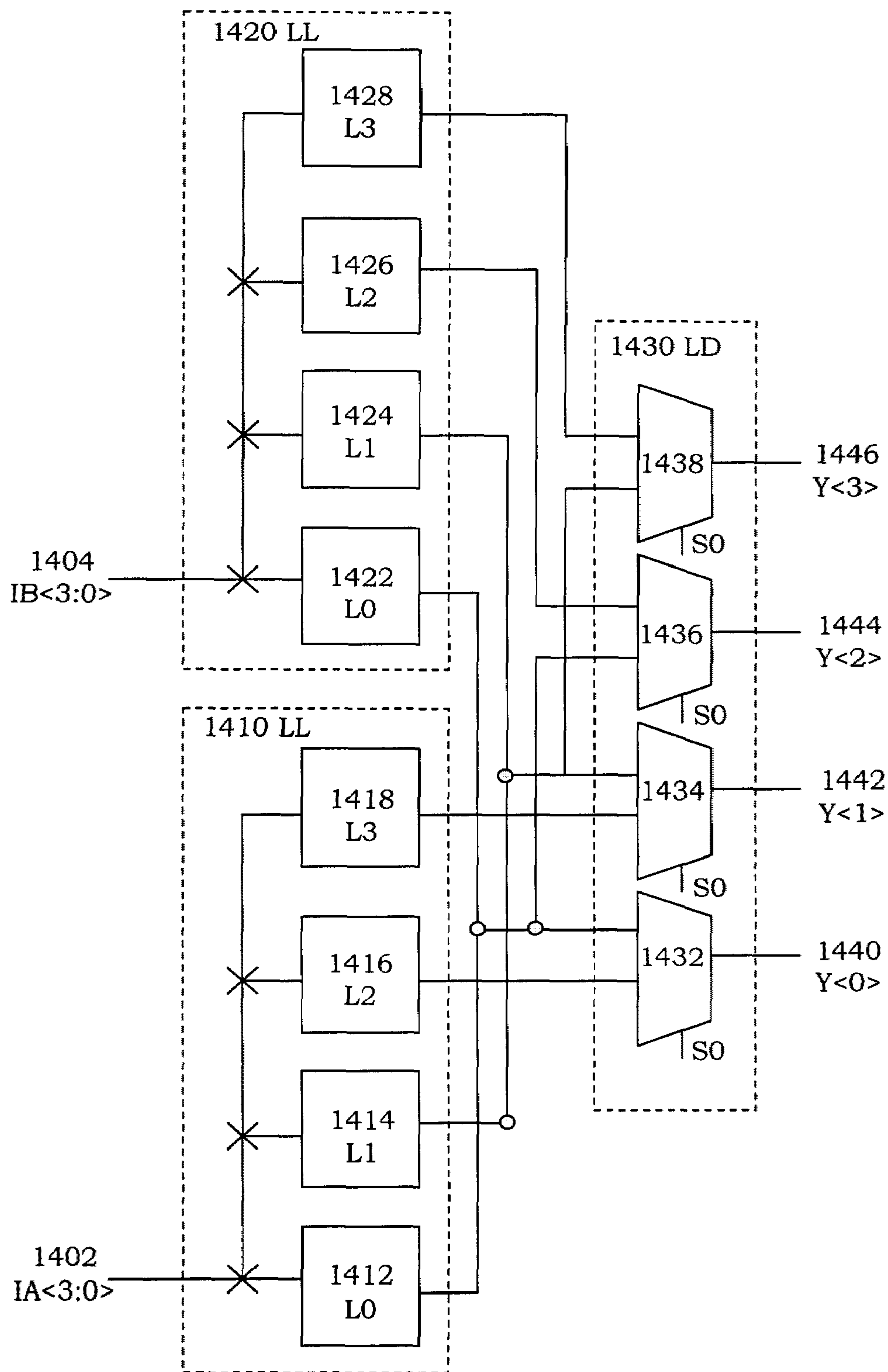
1400 4 2:1 multiplexer
