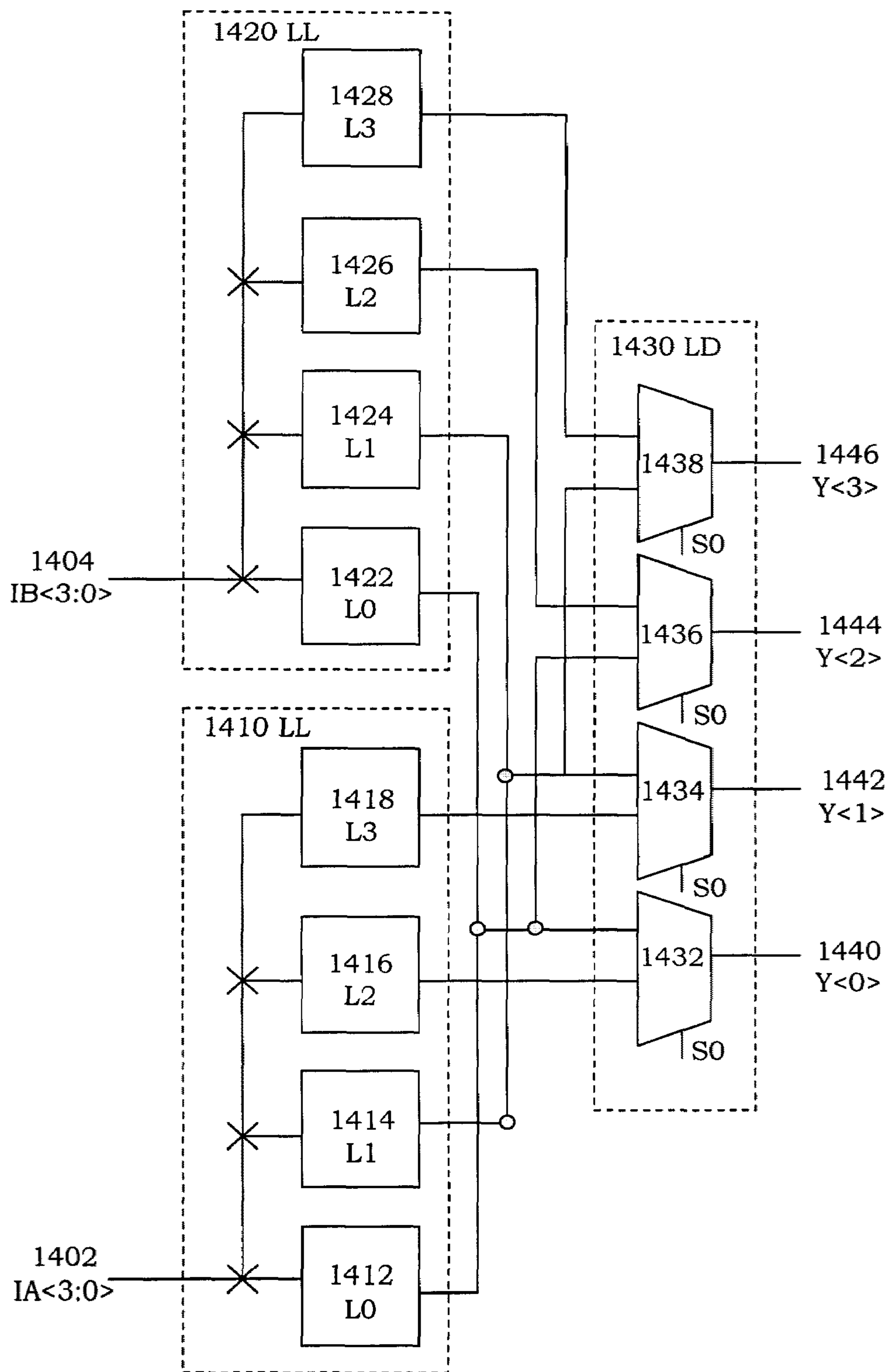
1400 4 2:1 multiplexer FIG. 14
