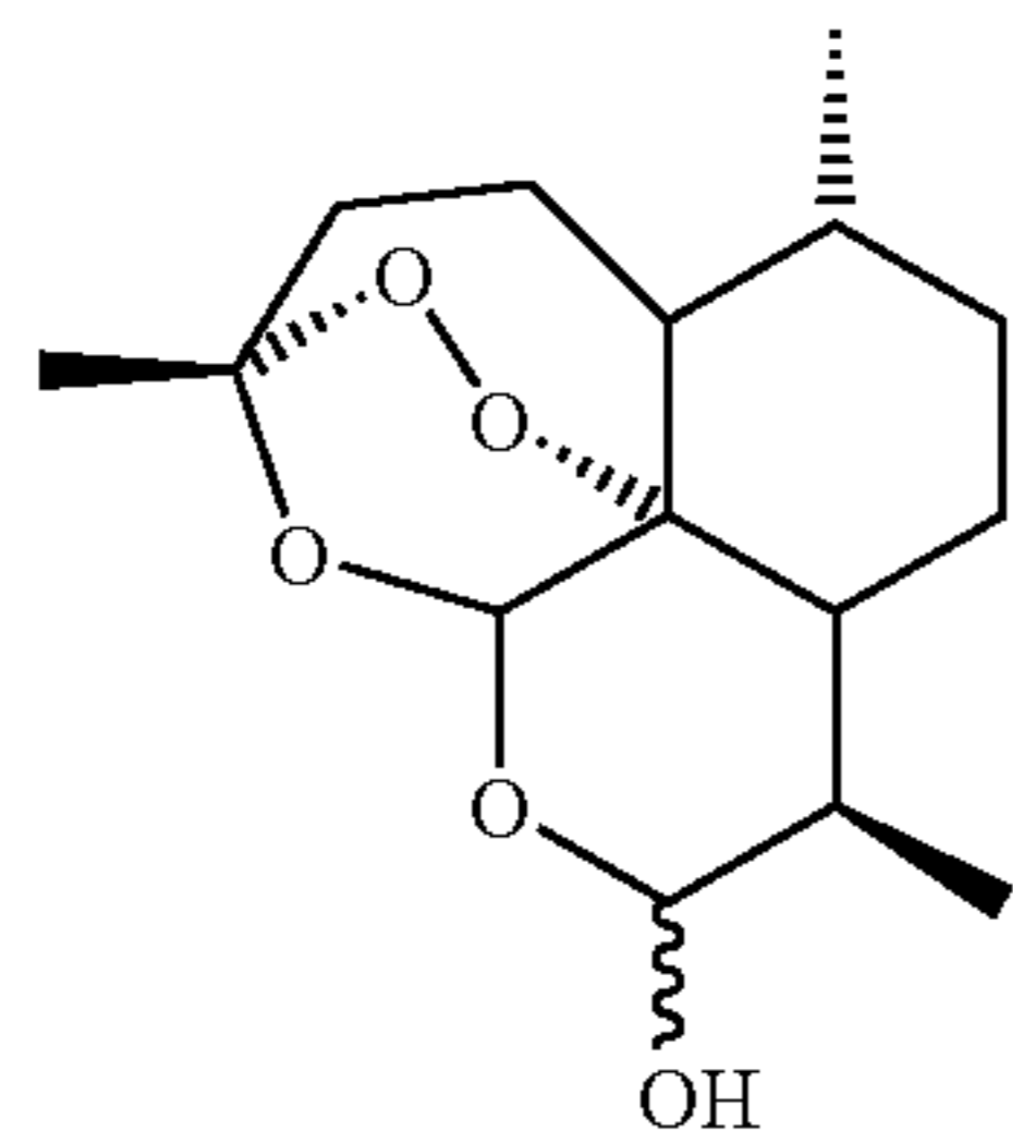
Artemisinin 1
