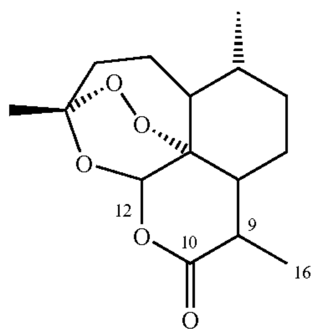
Artemisinin 1
