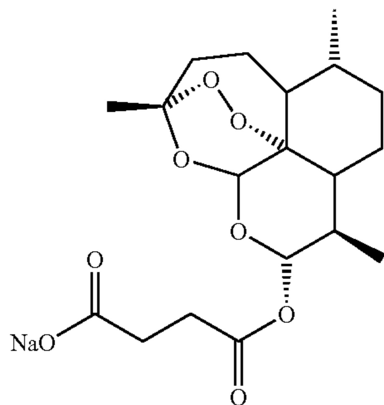
Sodium Artesunate 4
