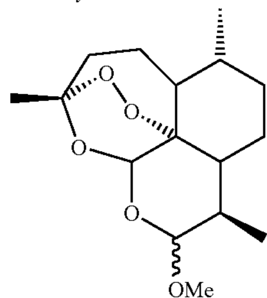
Artemether 3
