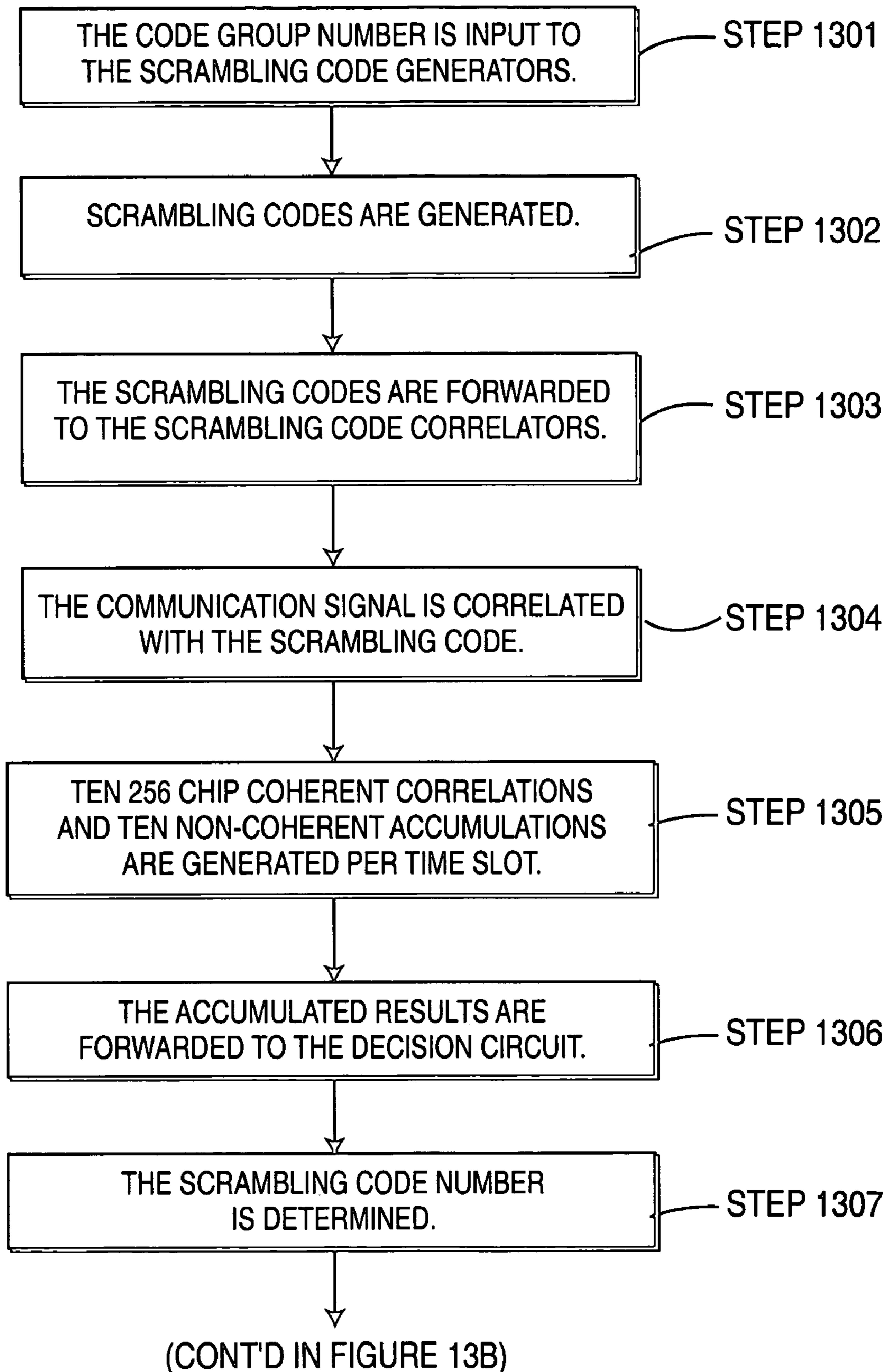
FIG. 13A
