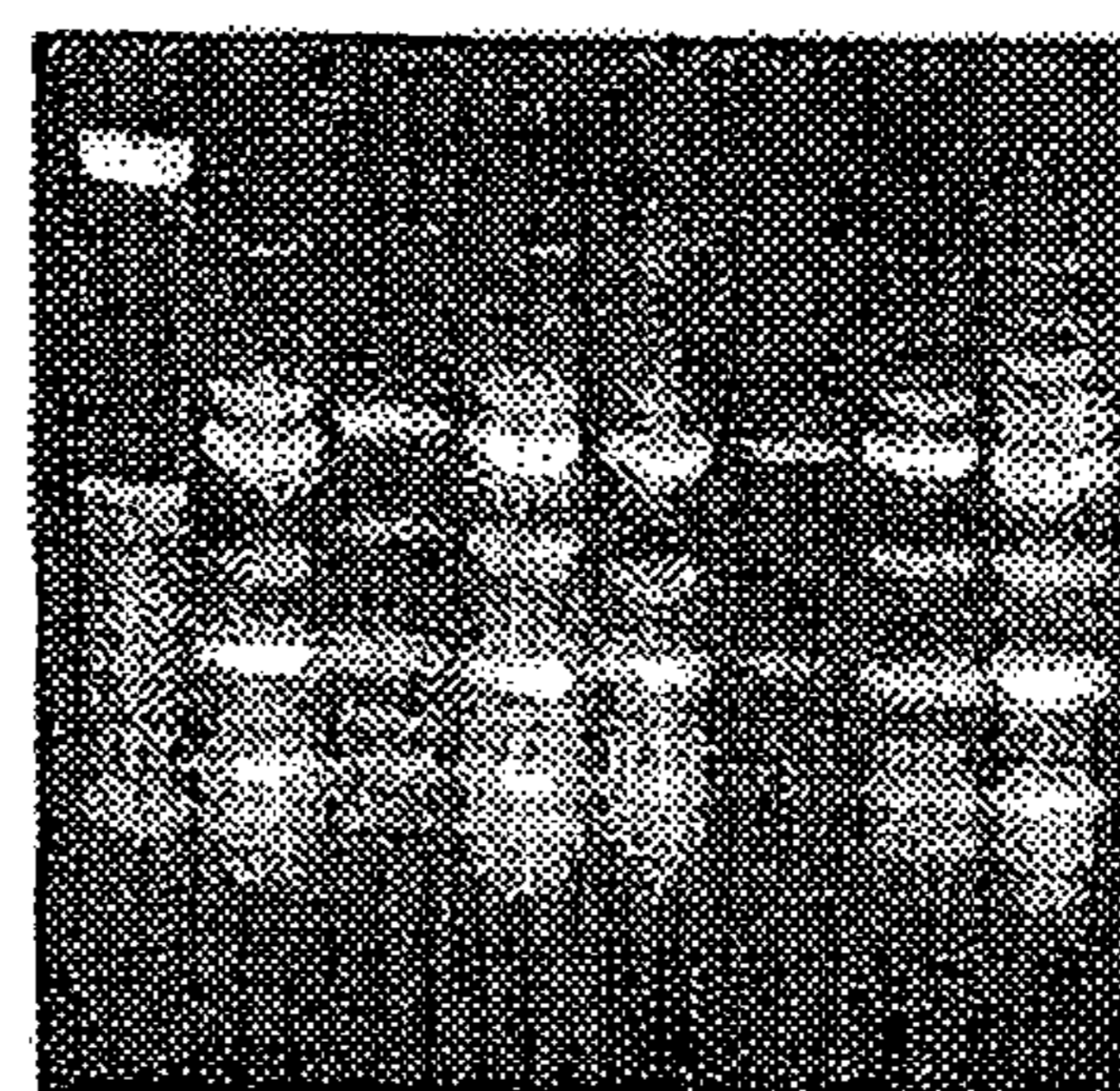
Gel II
