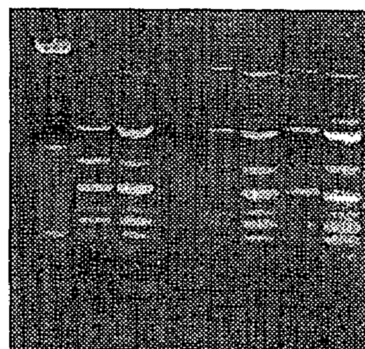
Gel III
