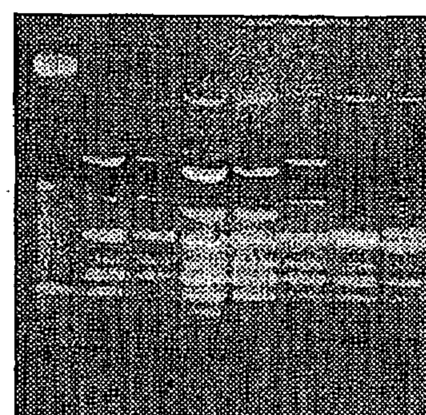
Gel IV
