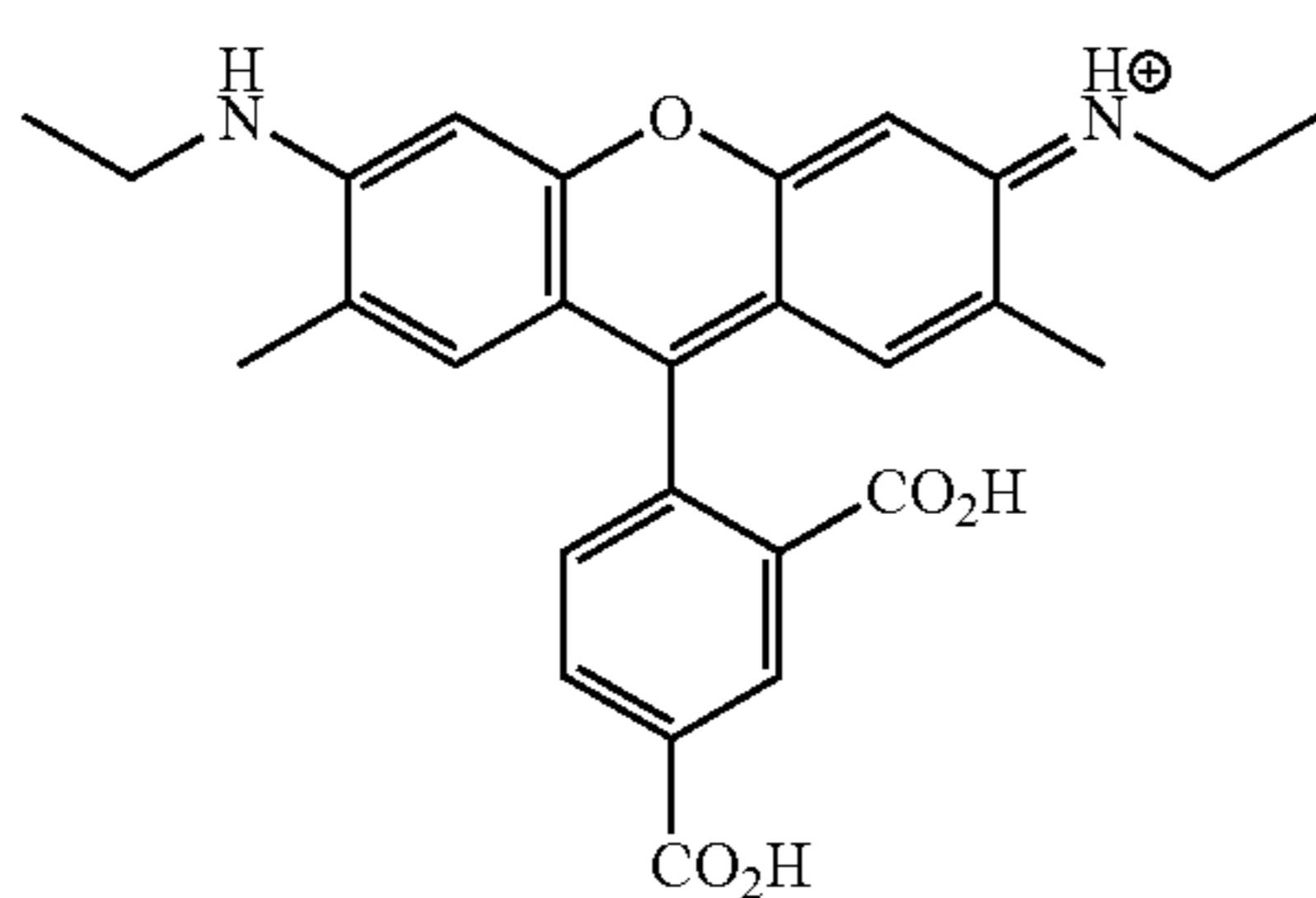
R6G
