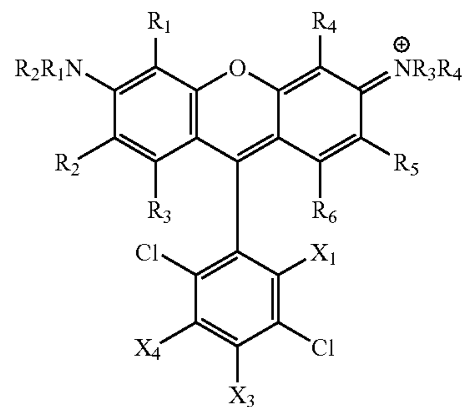
4,7-Dichlororhodamine
