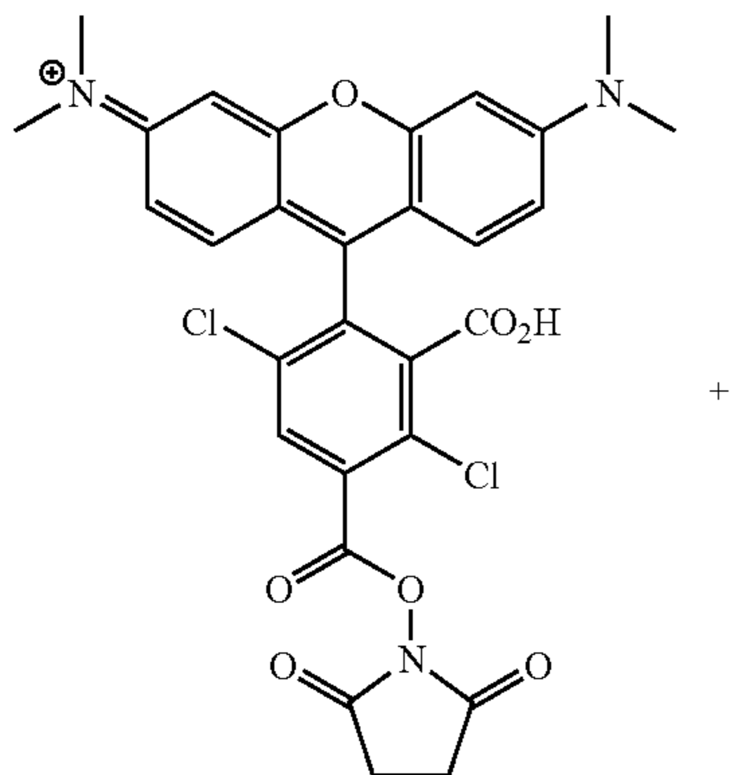
DTMR-2-NHS
