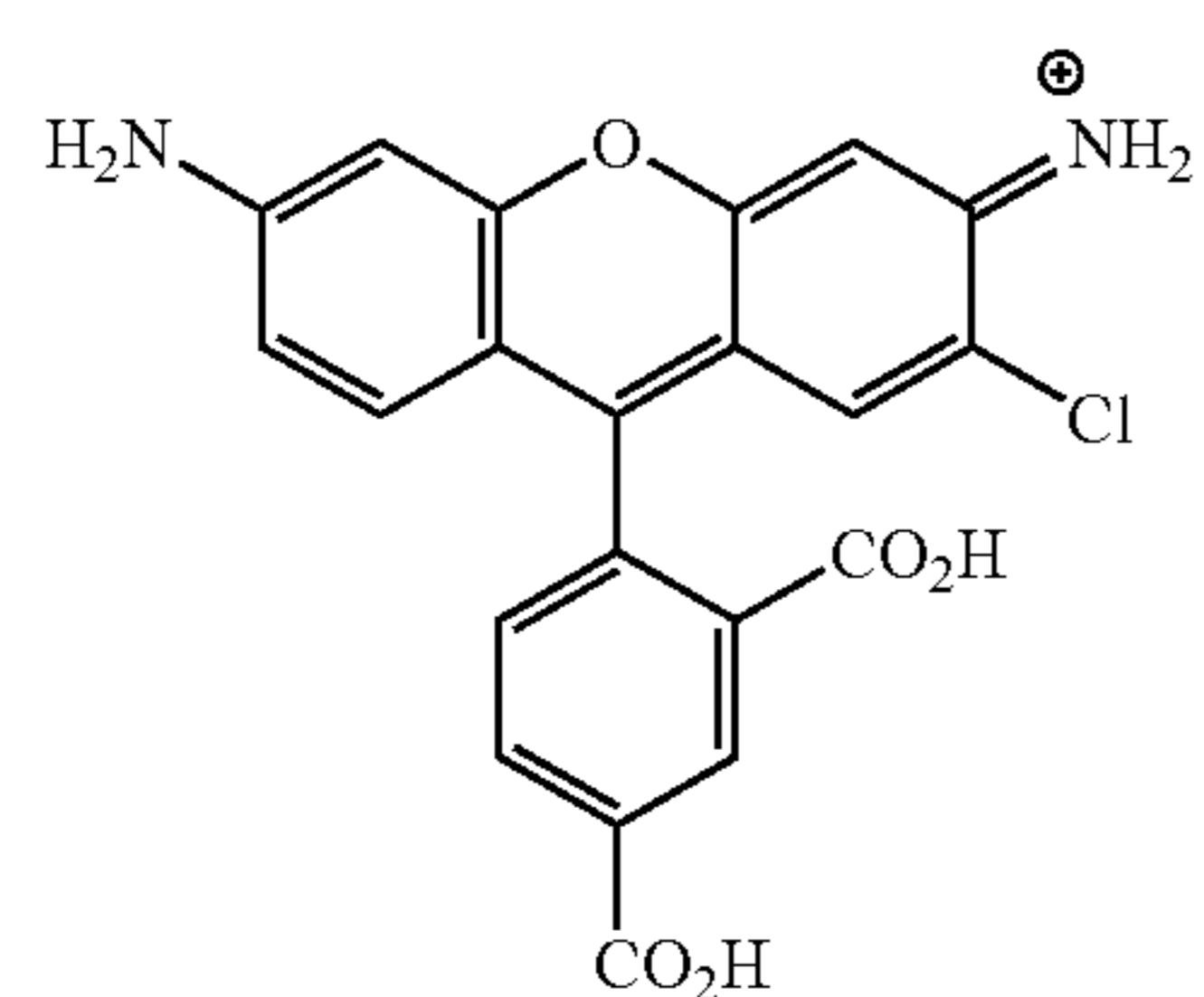
R110
