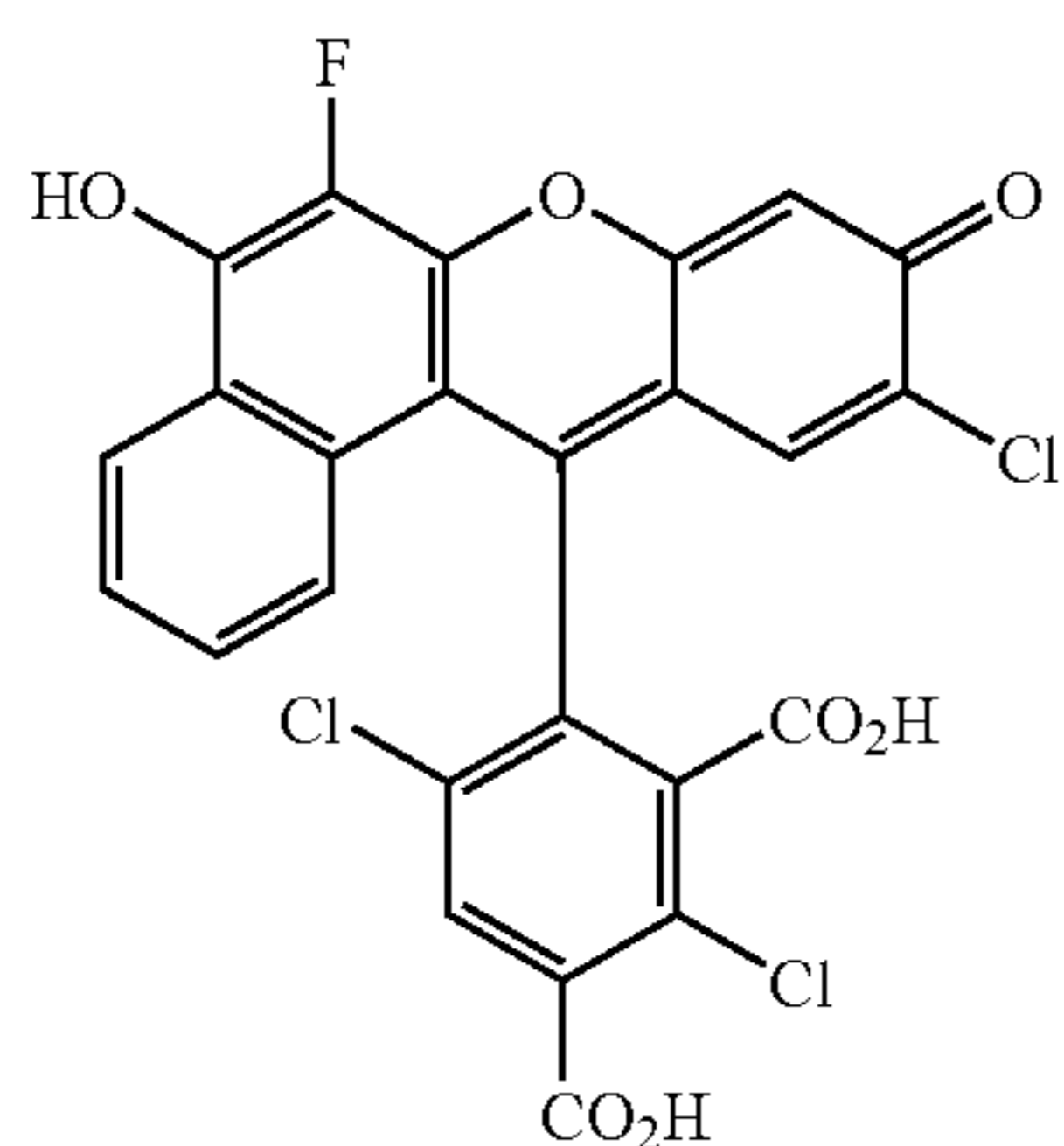
Cl-FLAN
