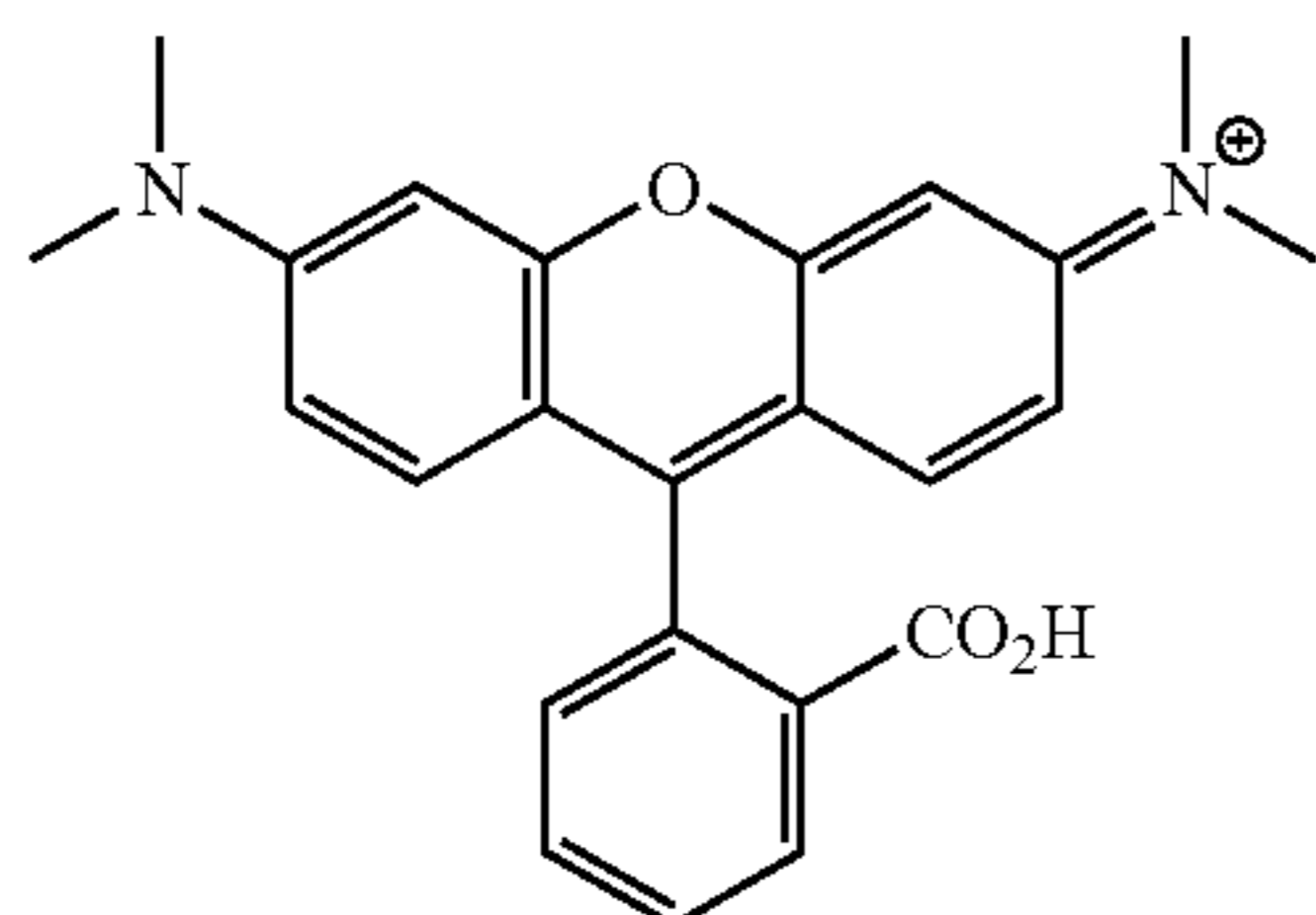
Rhodamine
