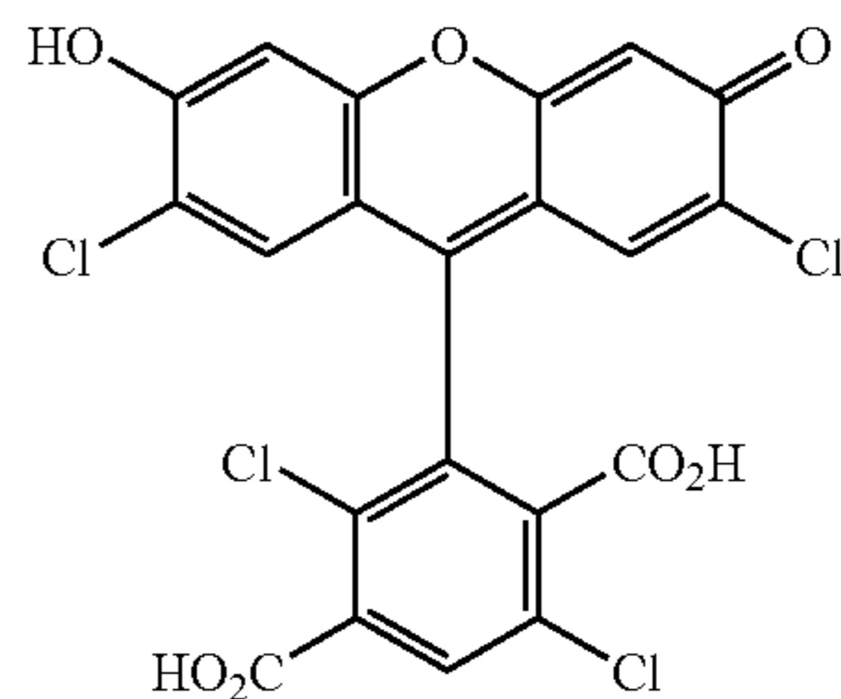
TET
