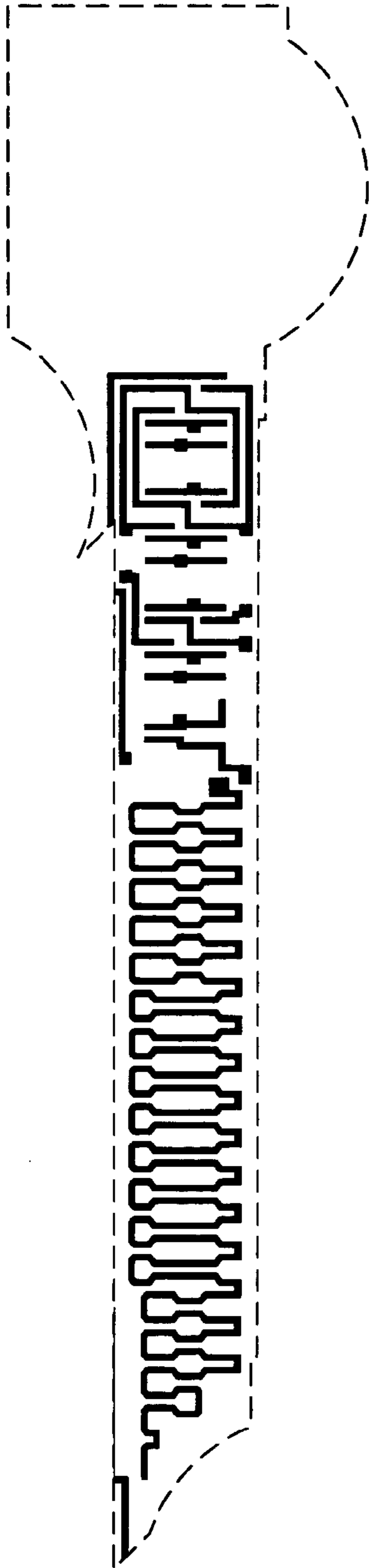
Poly mask
