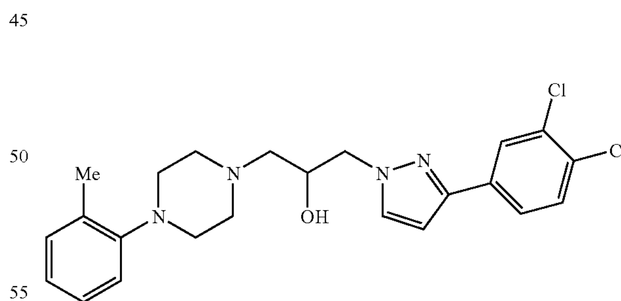
1-[3-(3,4-Dichloro-phenyl)-pyrazol-1-yl]-3-(4-o-tolyl-piperazin-1-yl)-propan-2-ol
