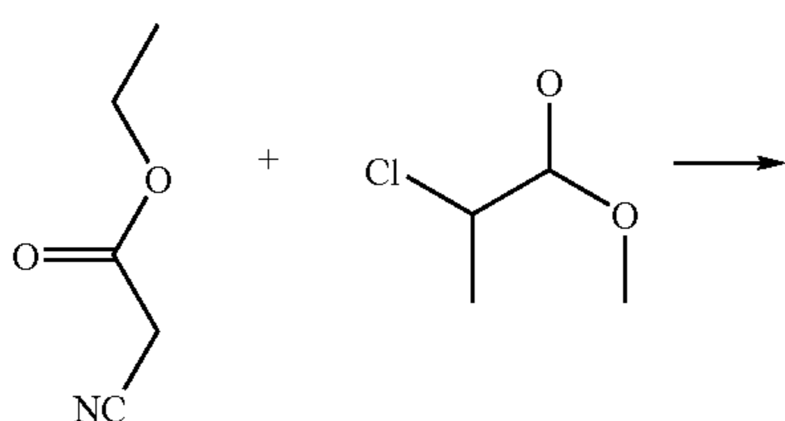
Scheme VI
