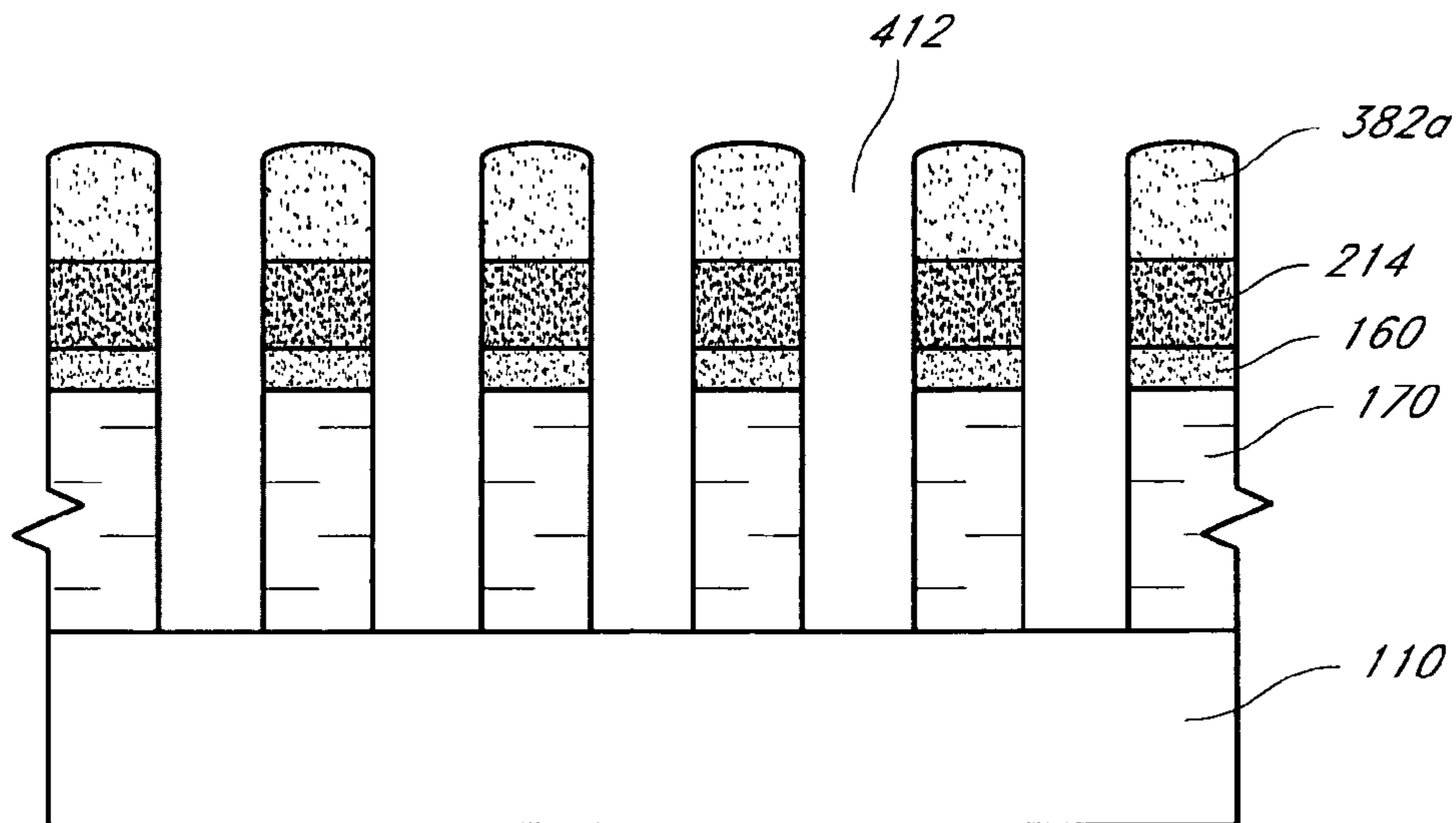
FIG. 19D
