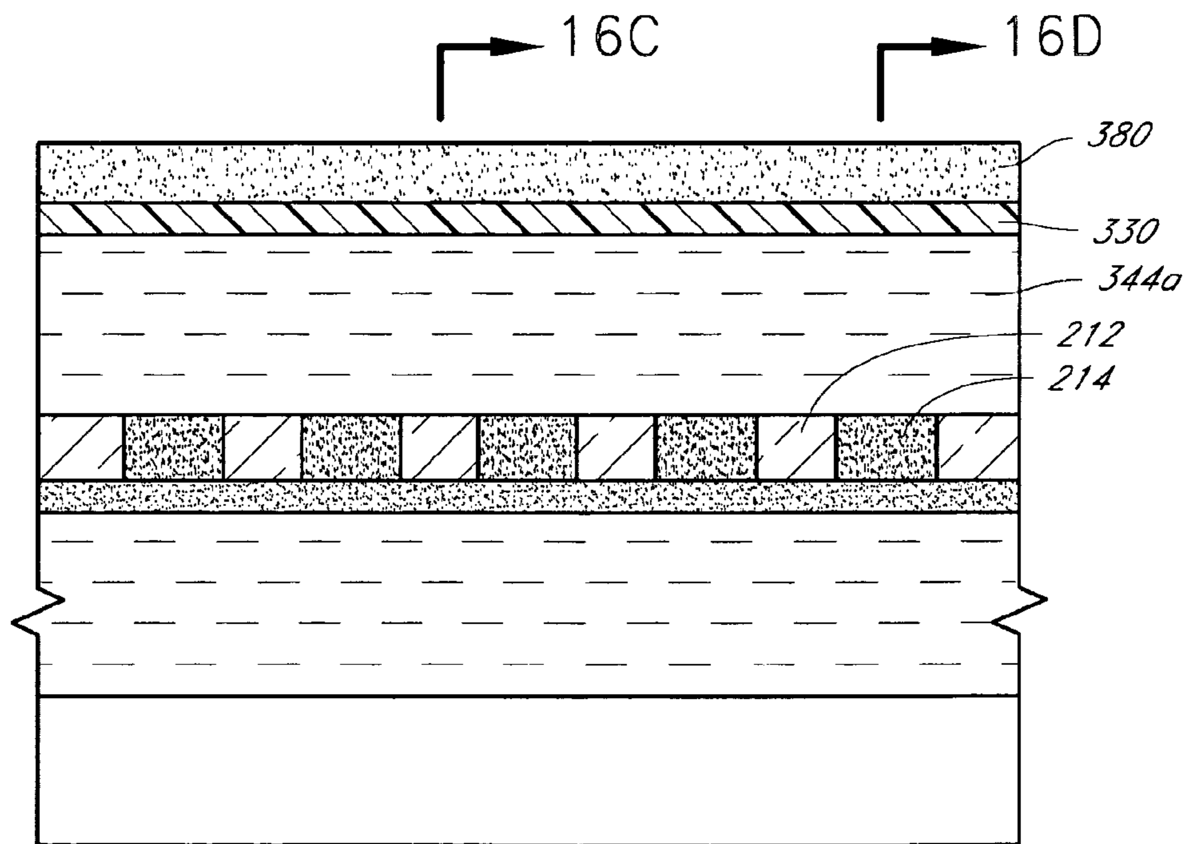
FIG. 16B
