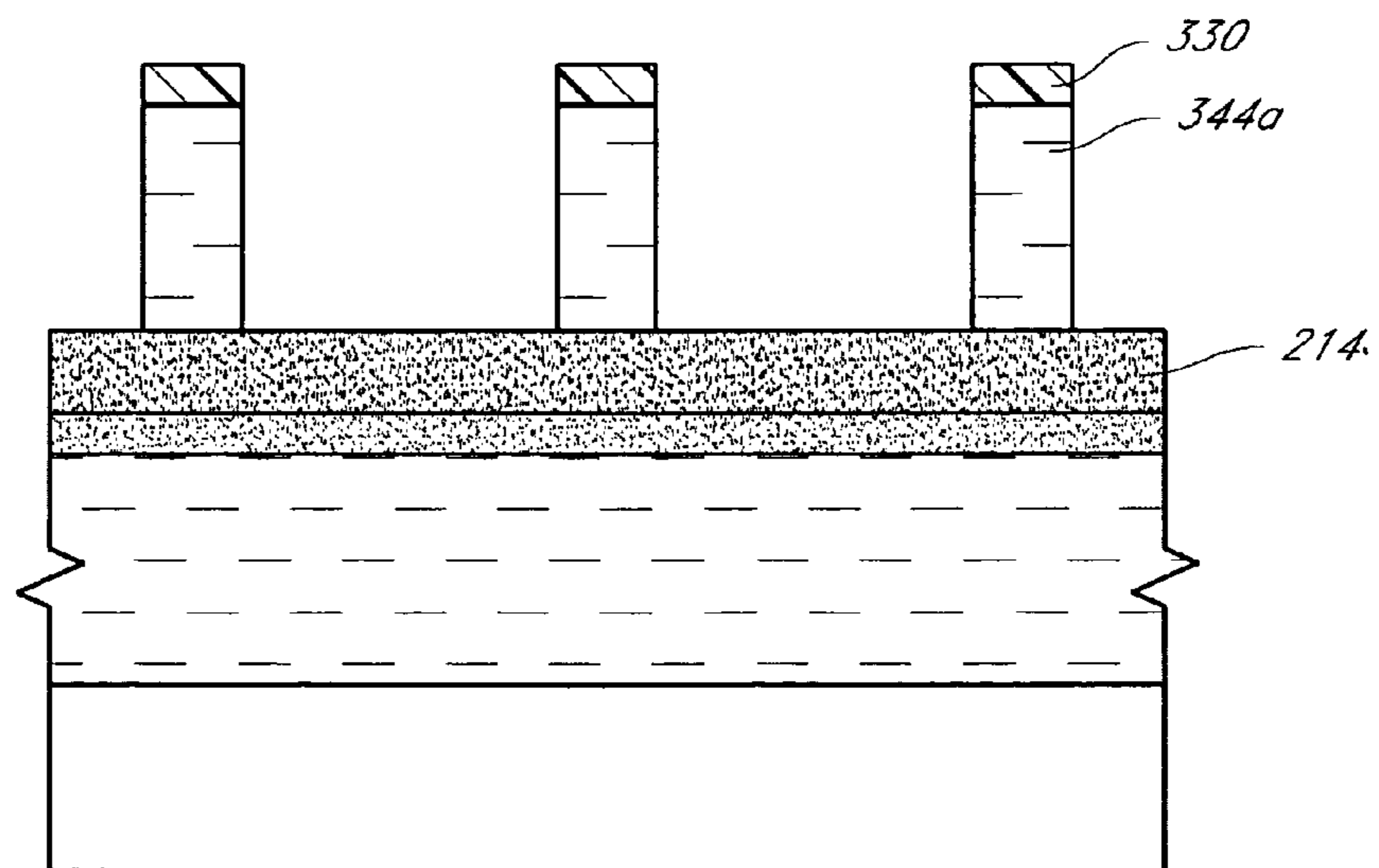
FIG. 15D
