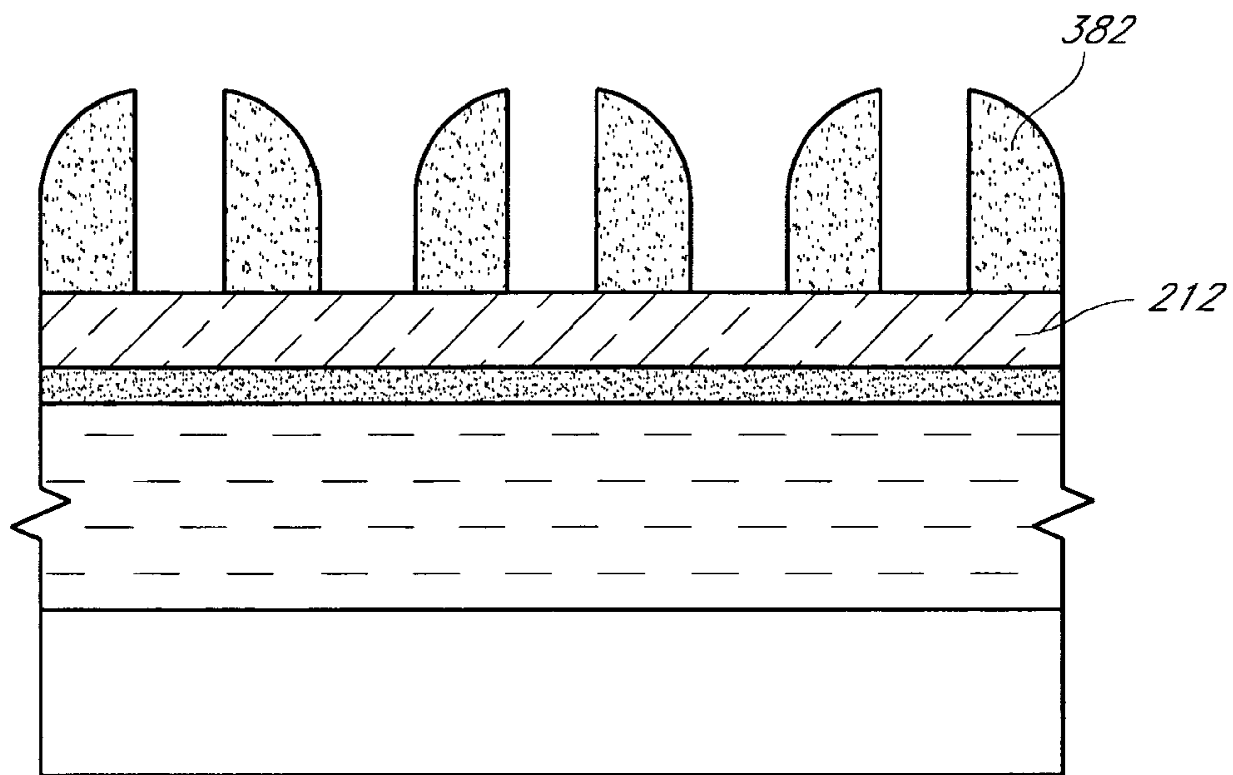
FIG. 17C
