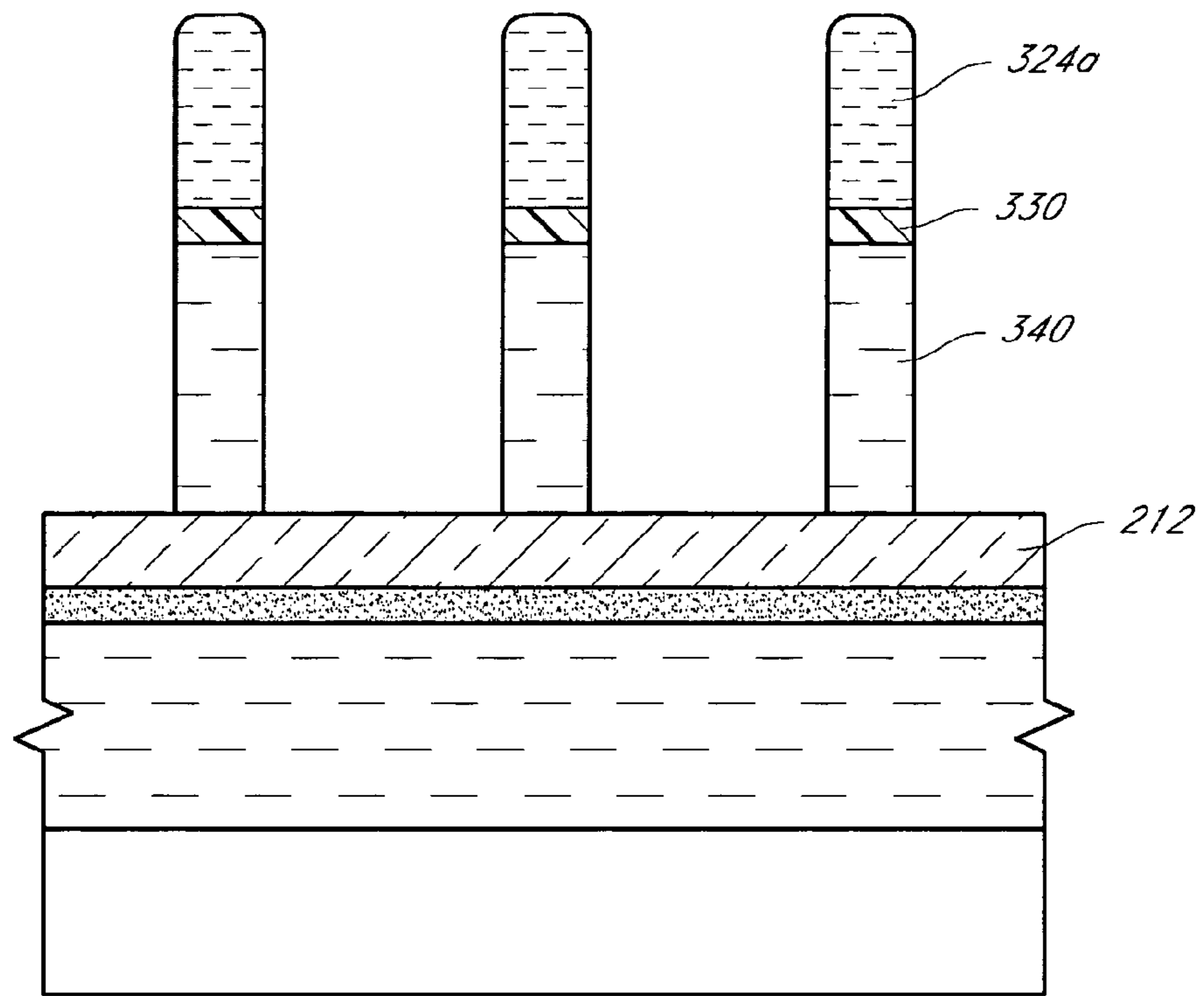
FIG. 14C
