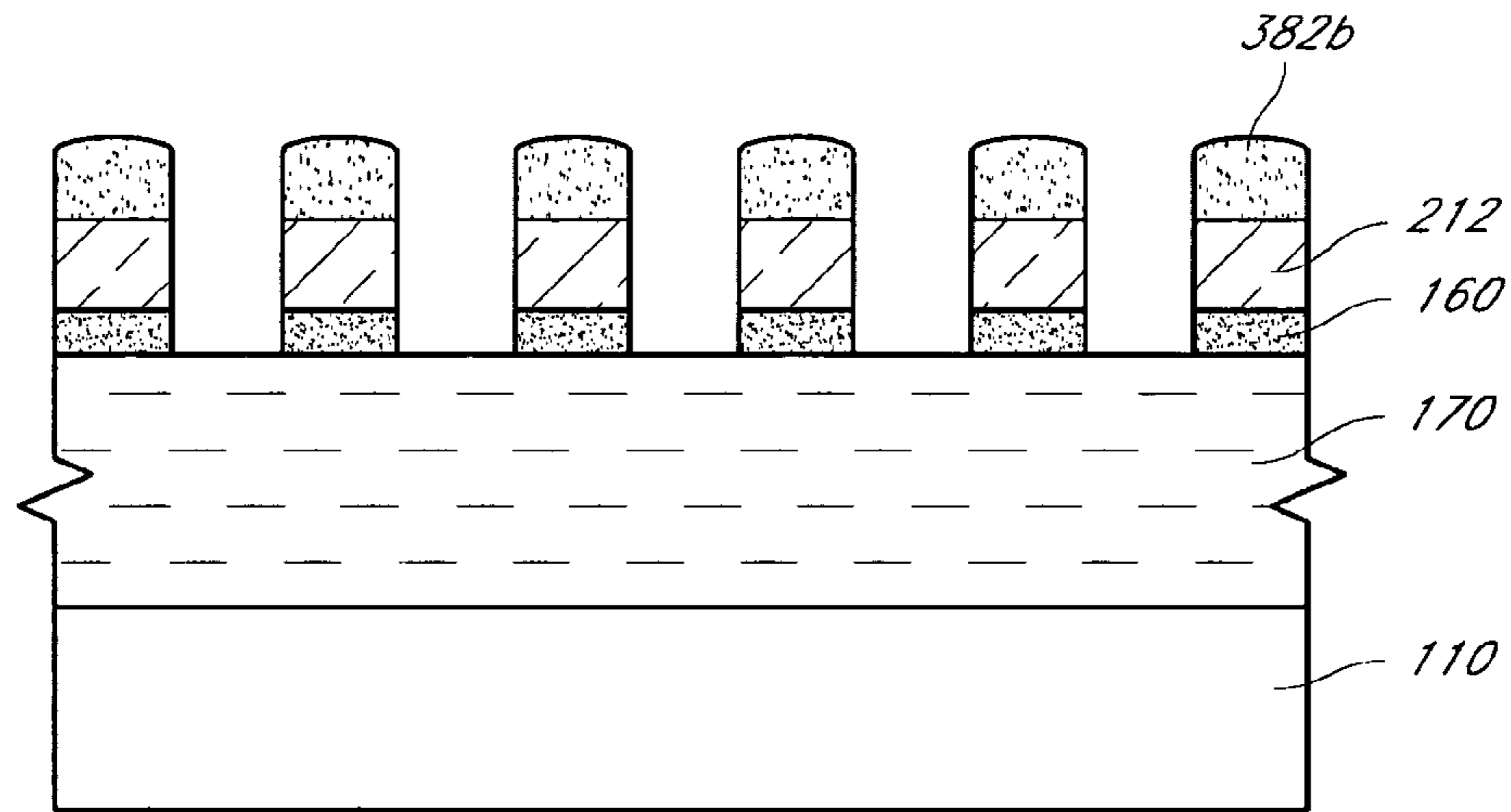
FIG. 26C
