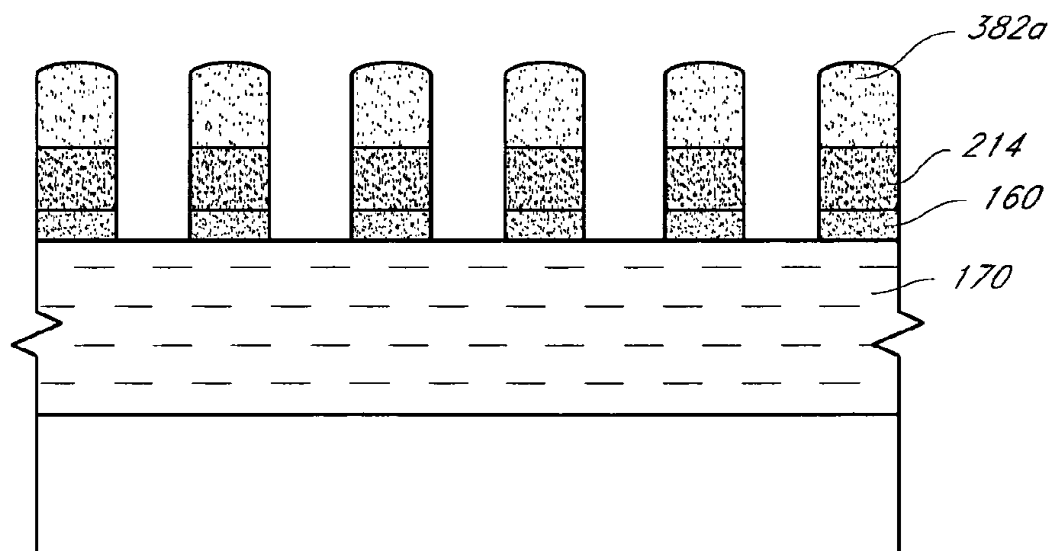
FIG. 18D
