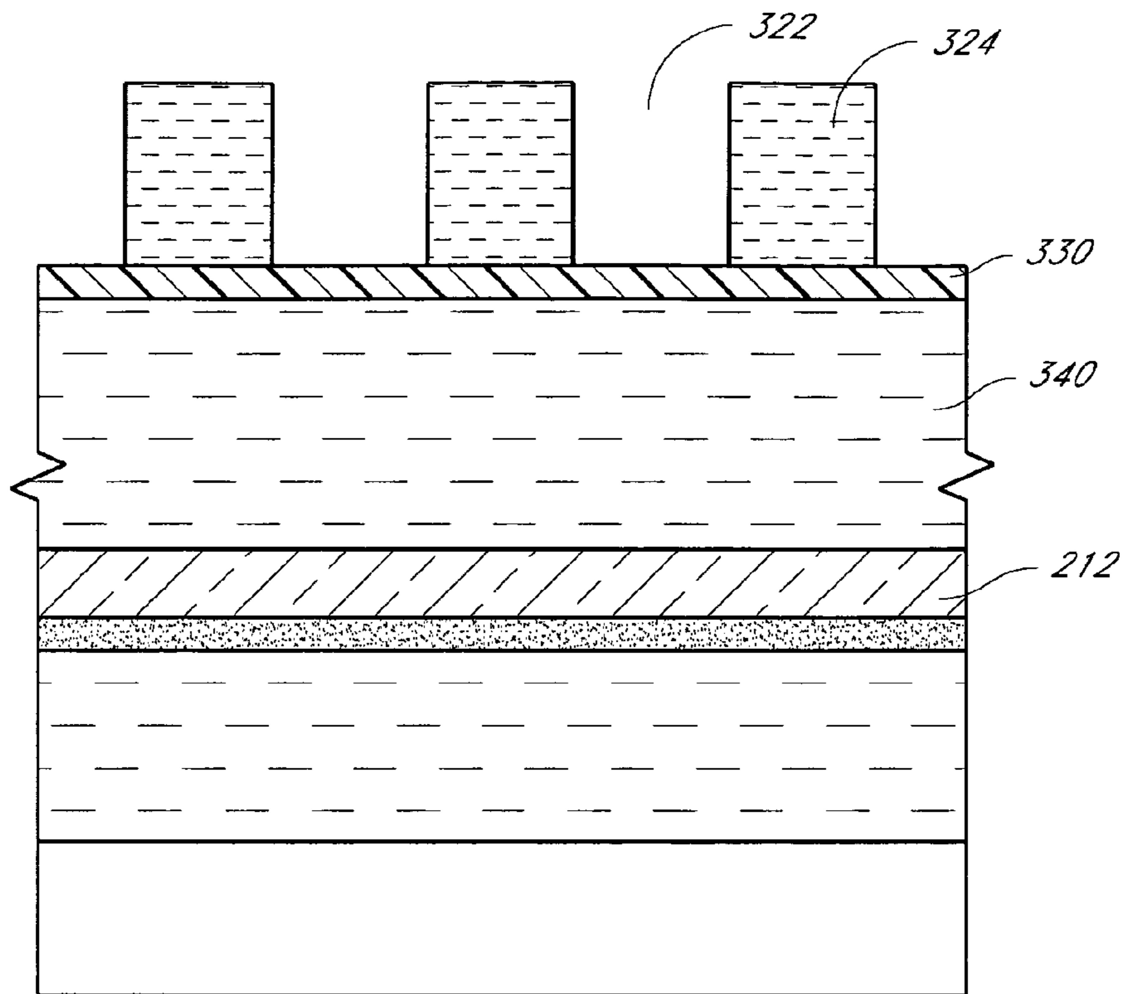
FIG. 12C
