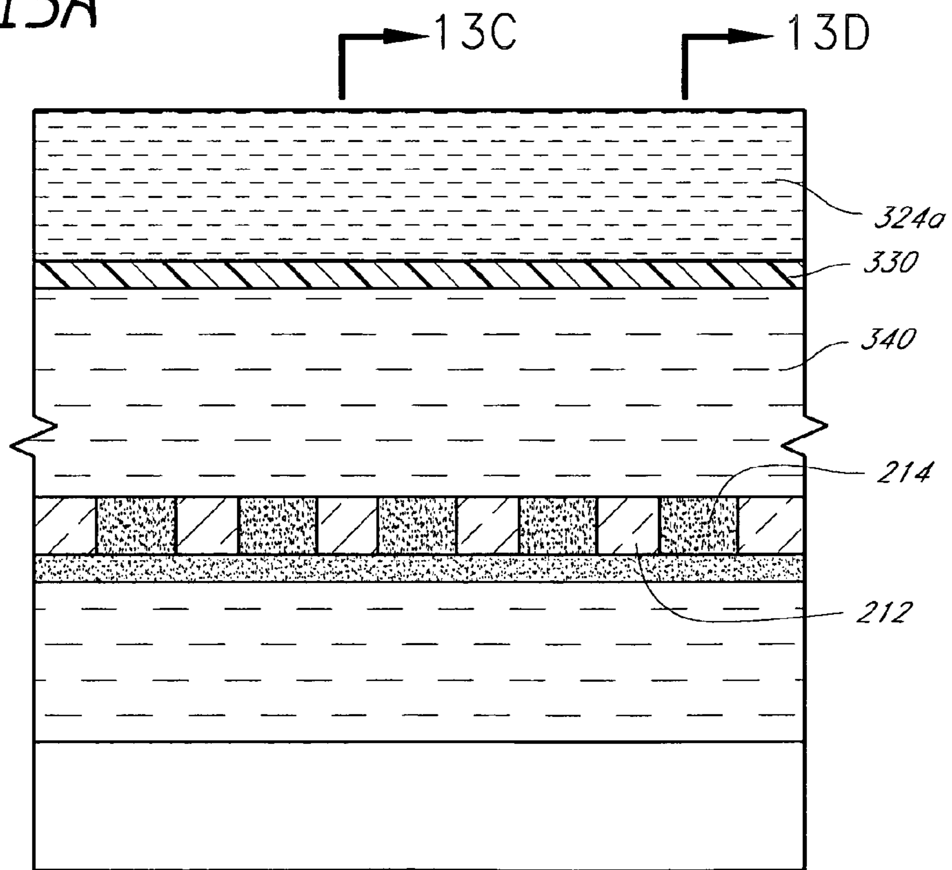
FIG. 13B
