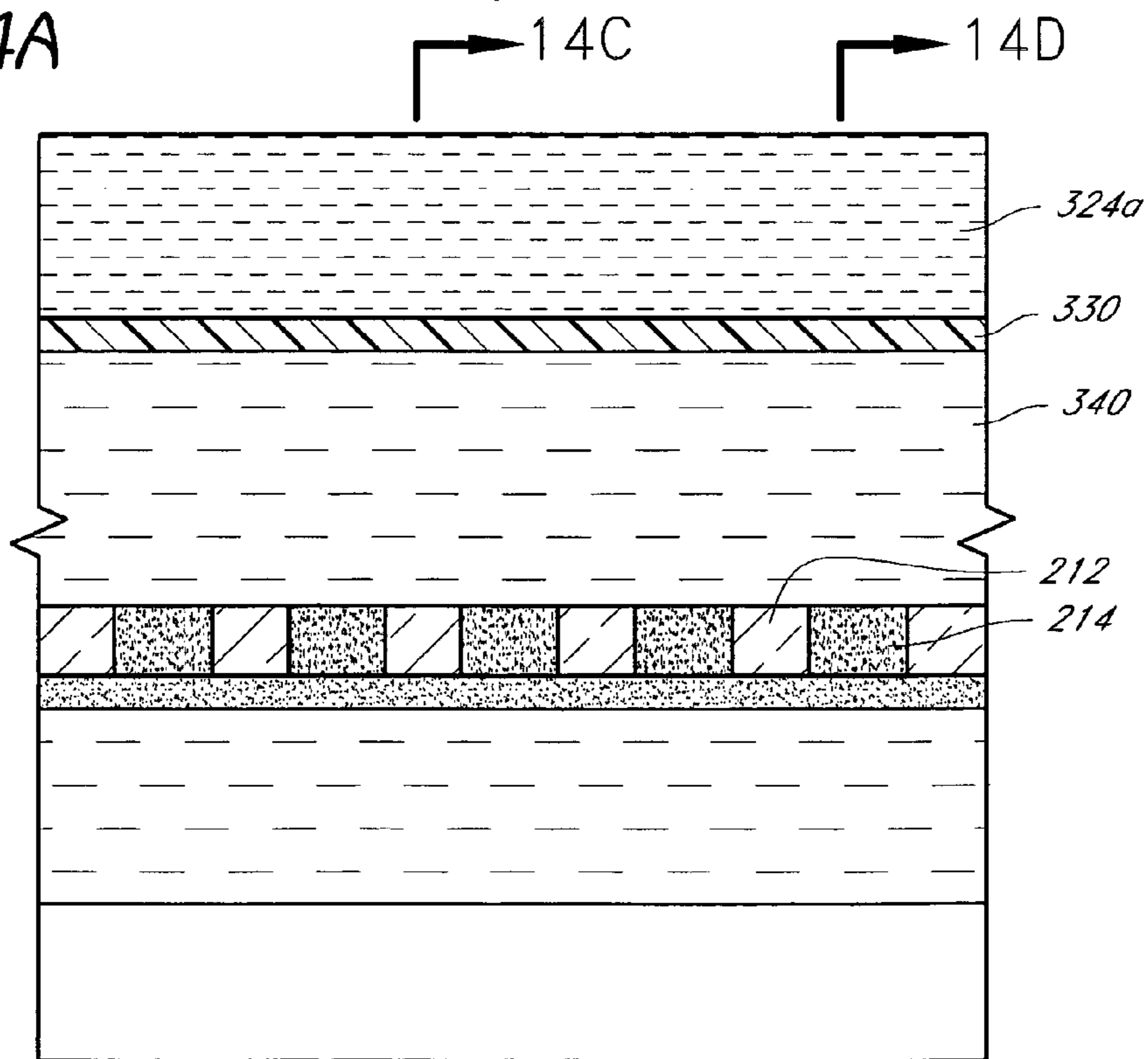
FIG. 14B
