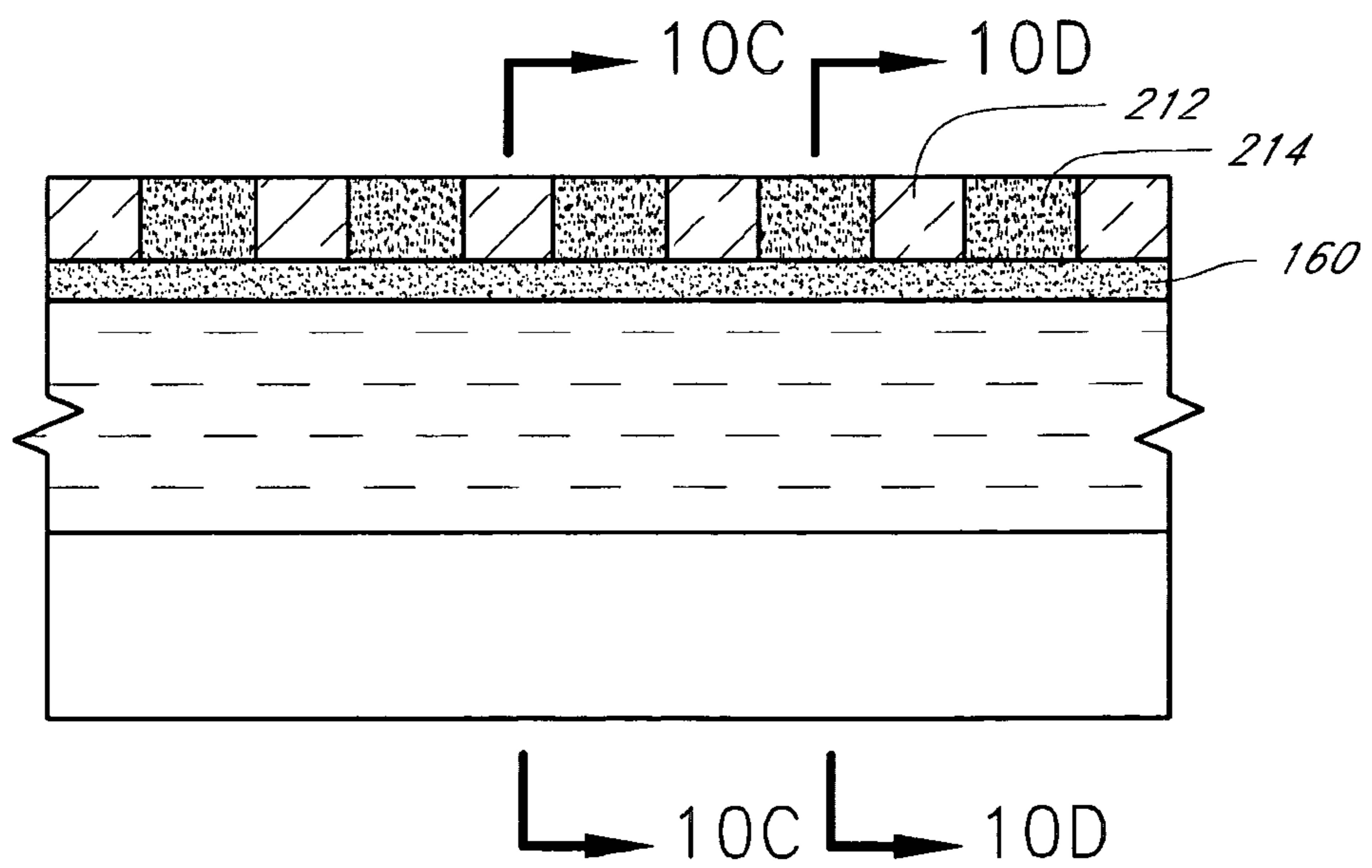
FIG. 10B
