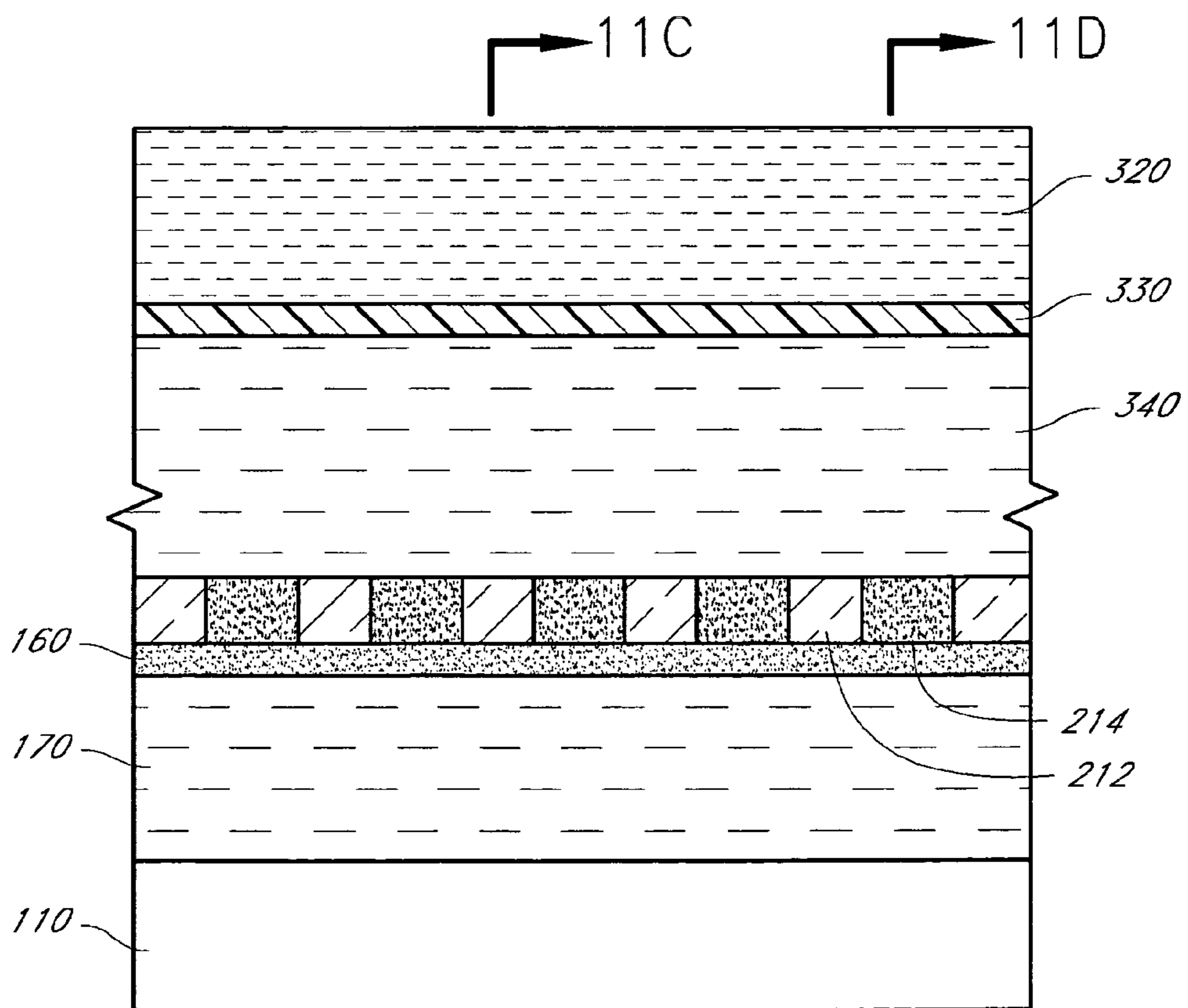
FIG. 11B
