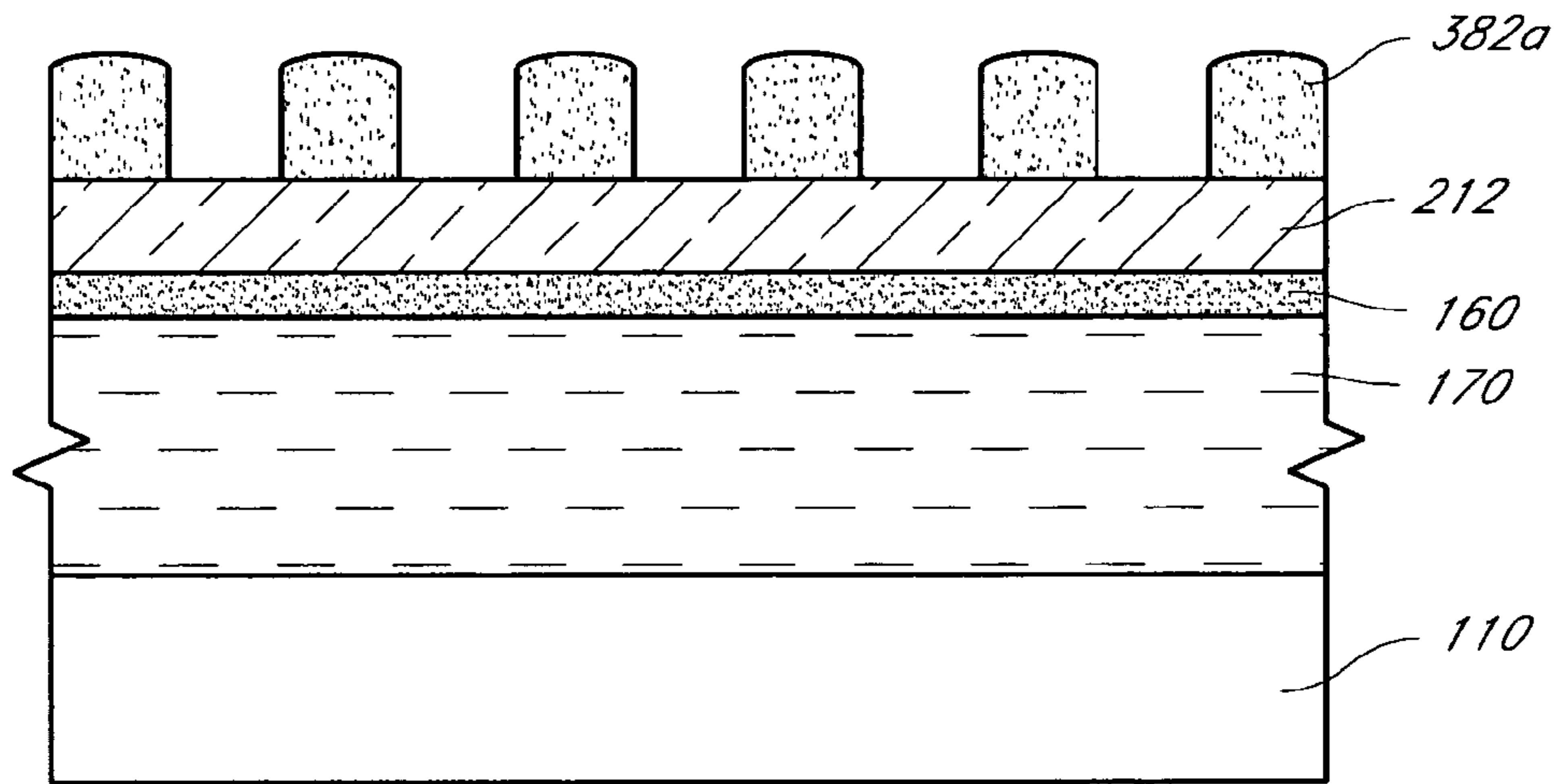
FIG. 19C
