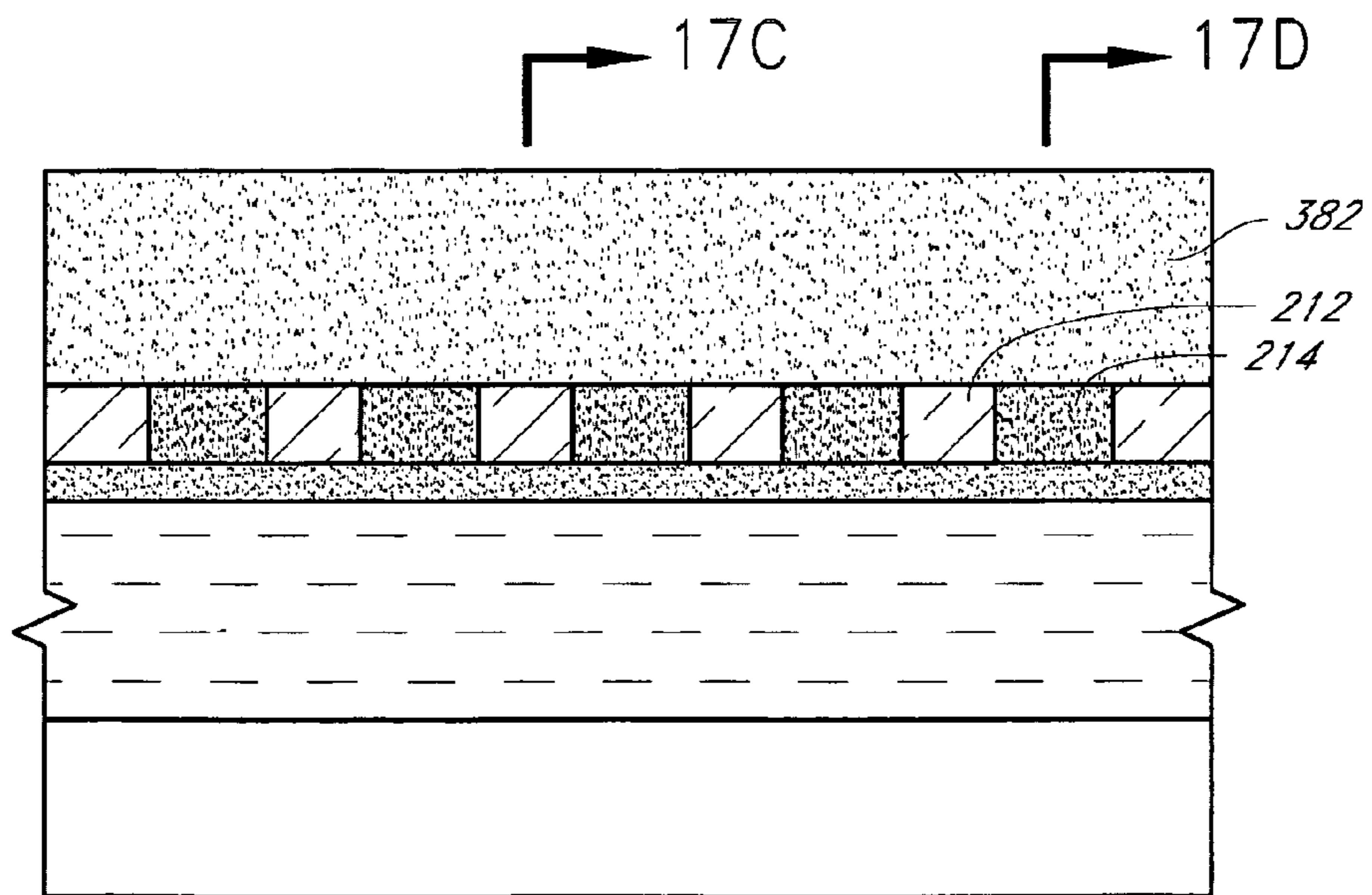
FIG. 17B
