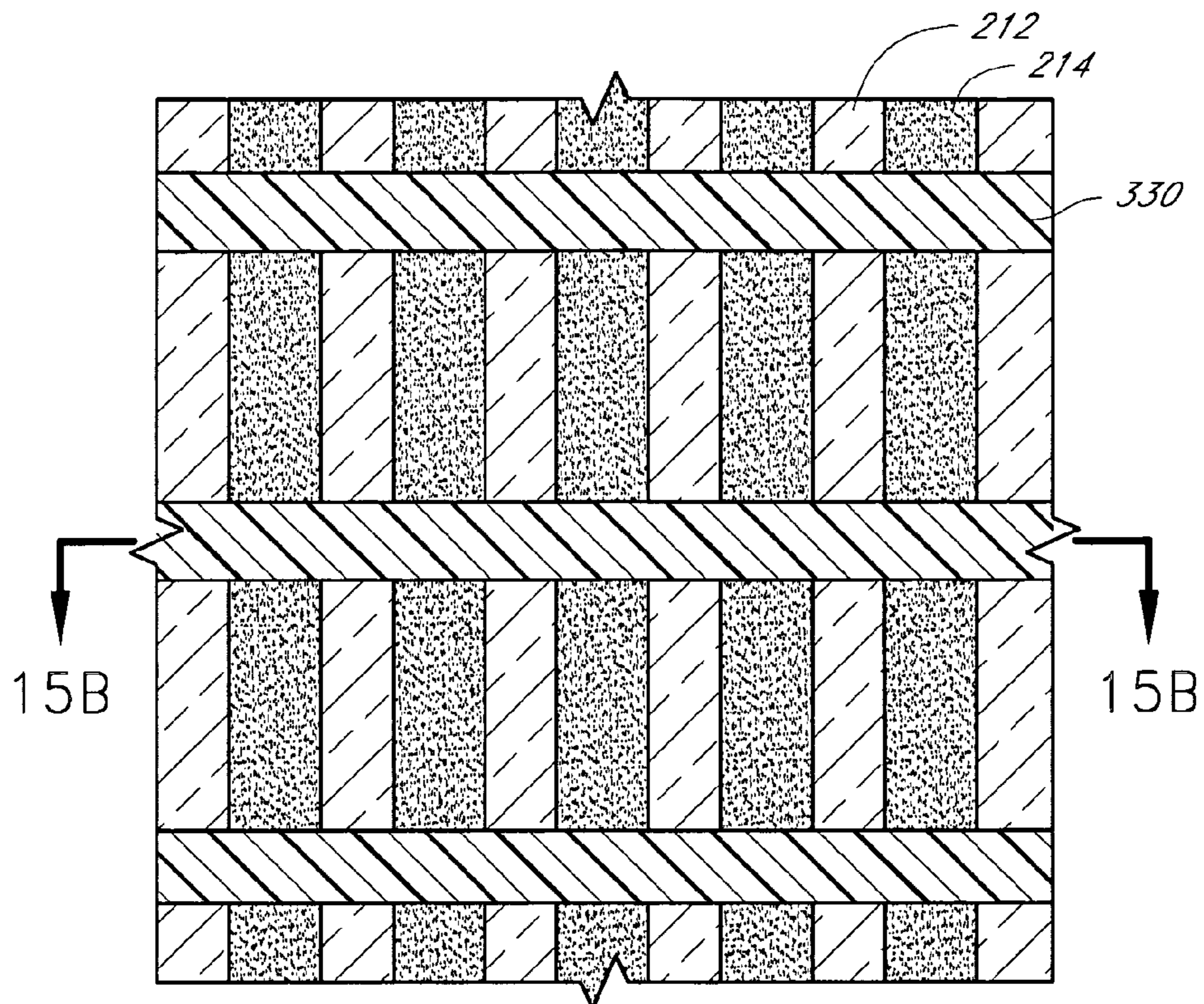
FIG. 15A
