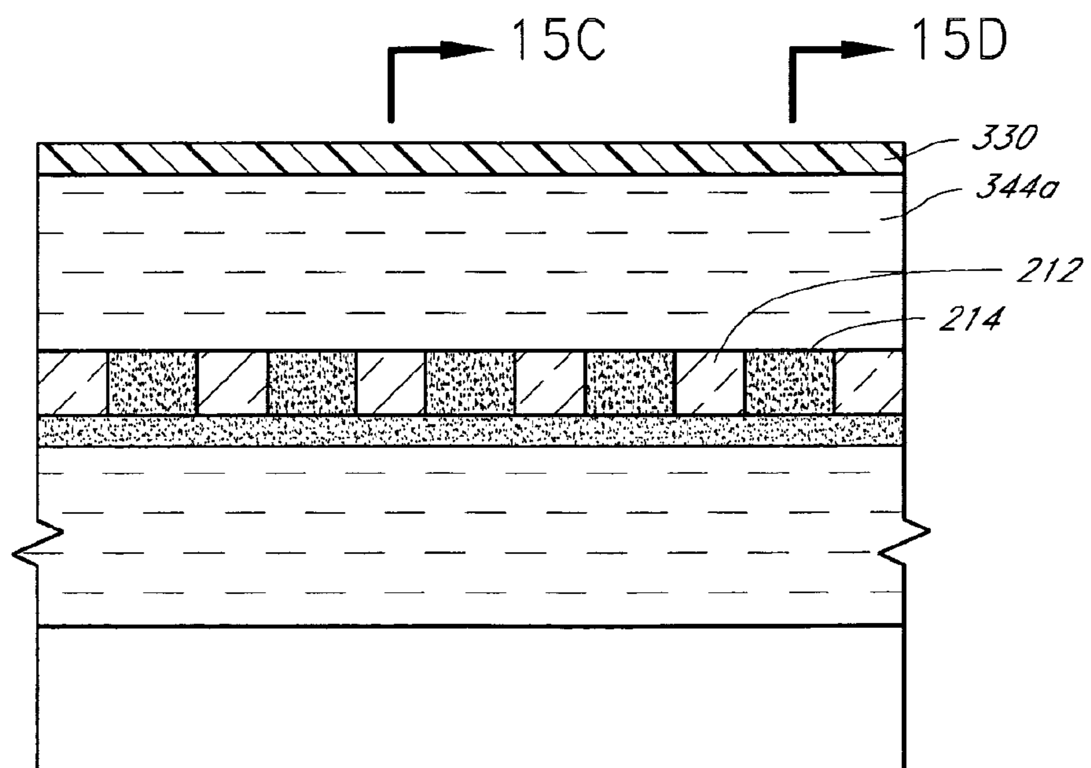
FIG. 15A
