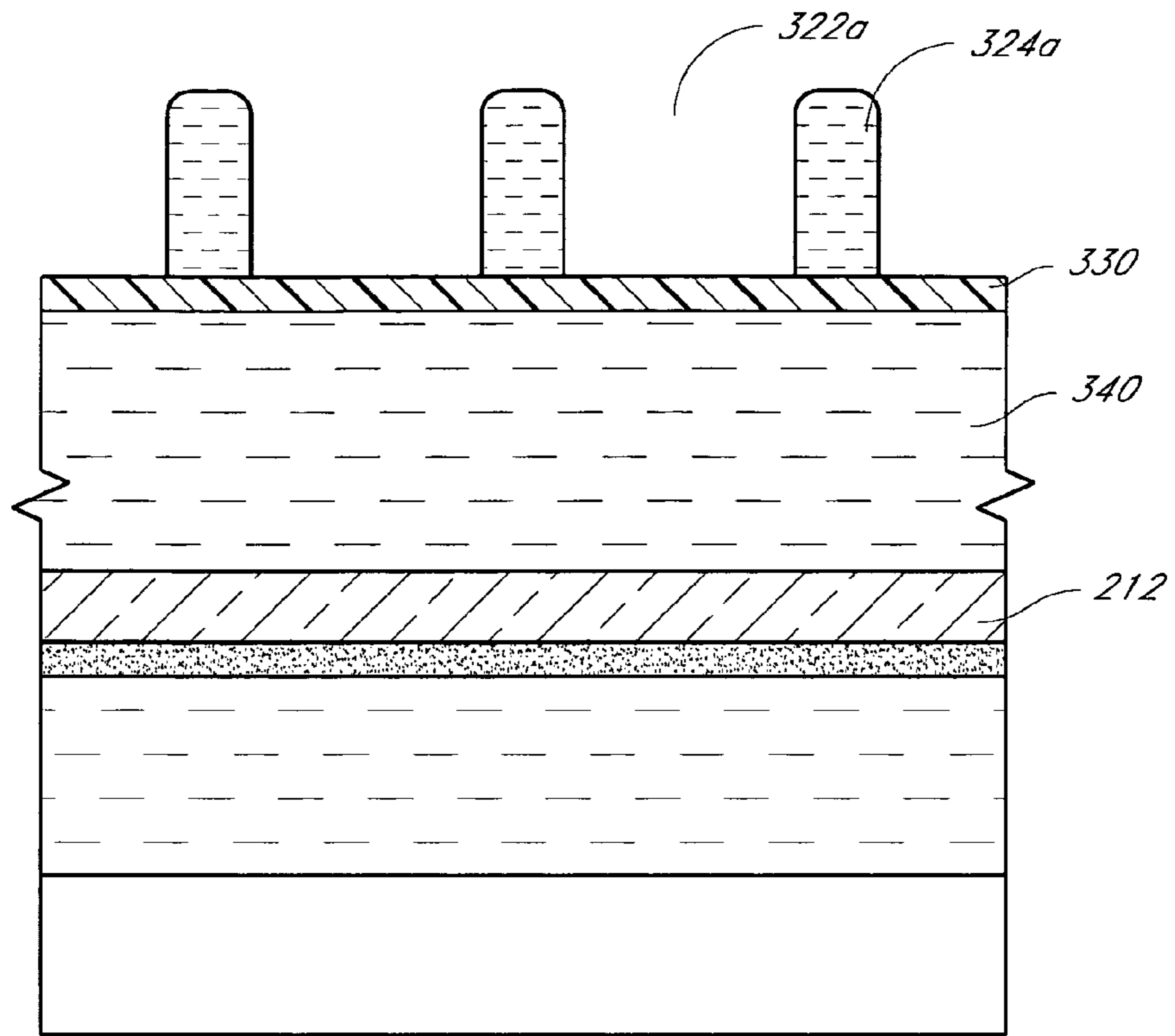
FIG. 13C
