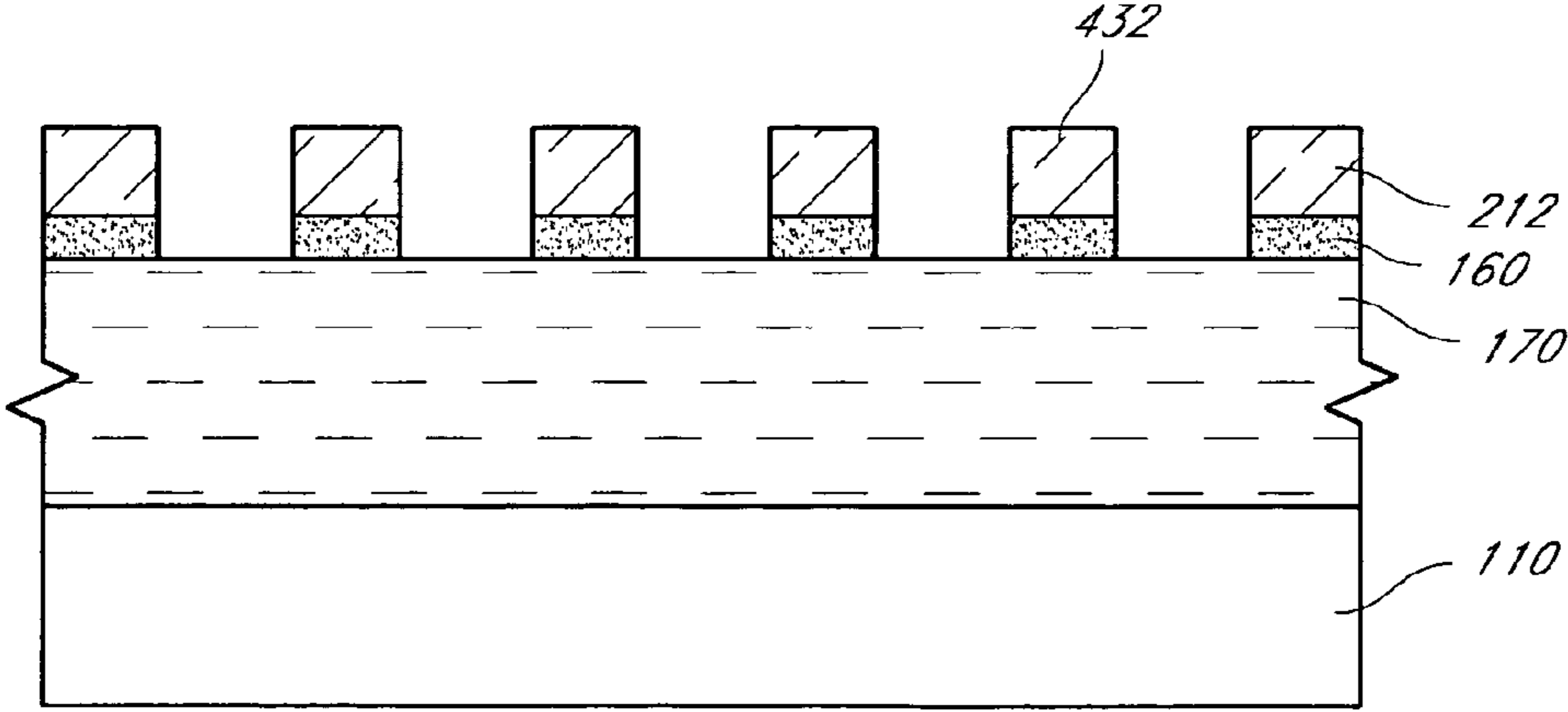
FIG. 23B
