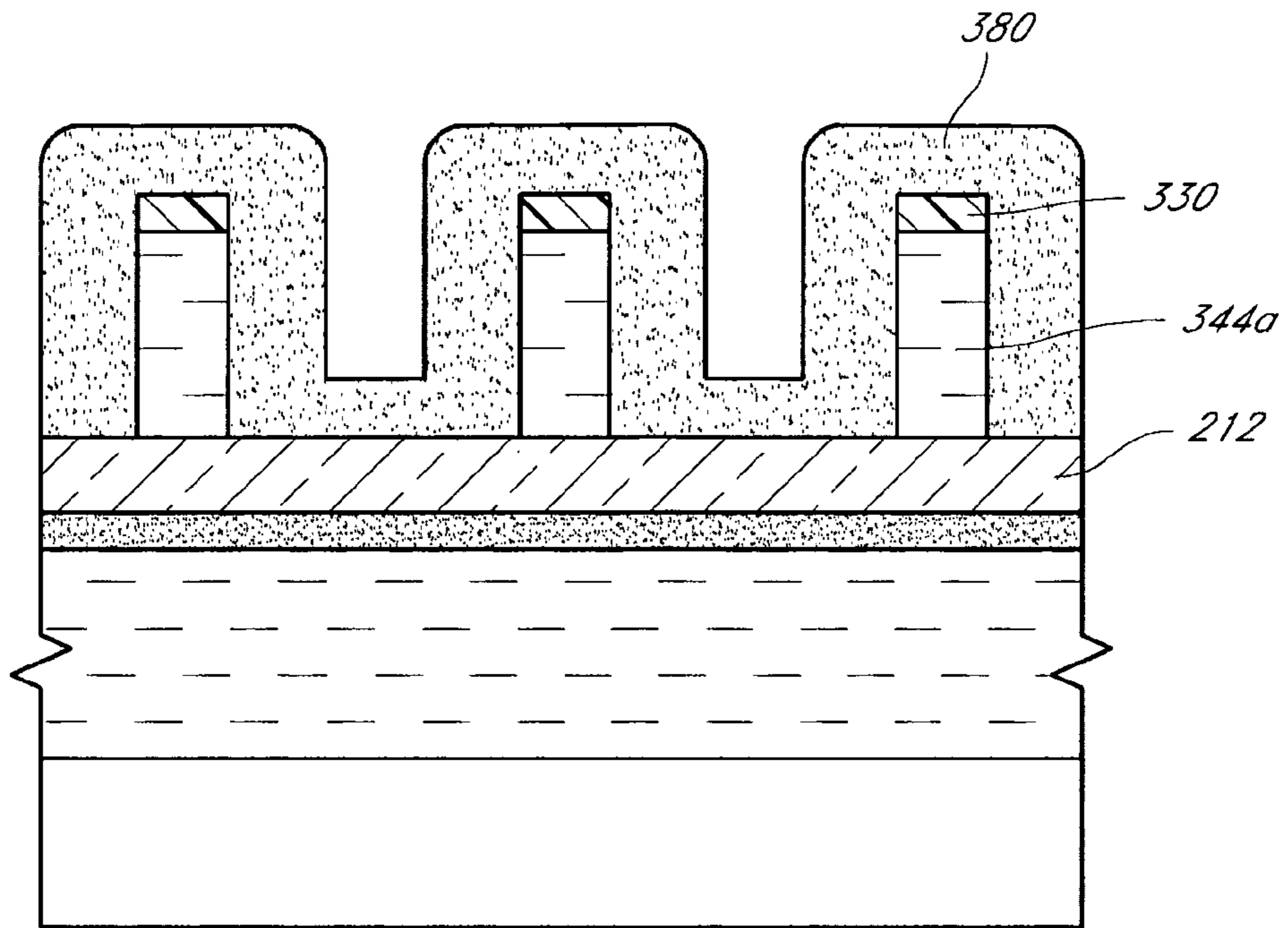
FIG. 16C
