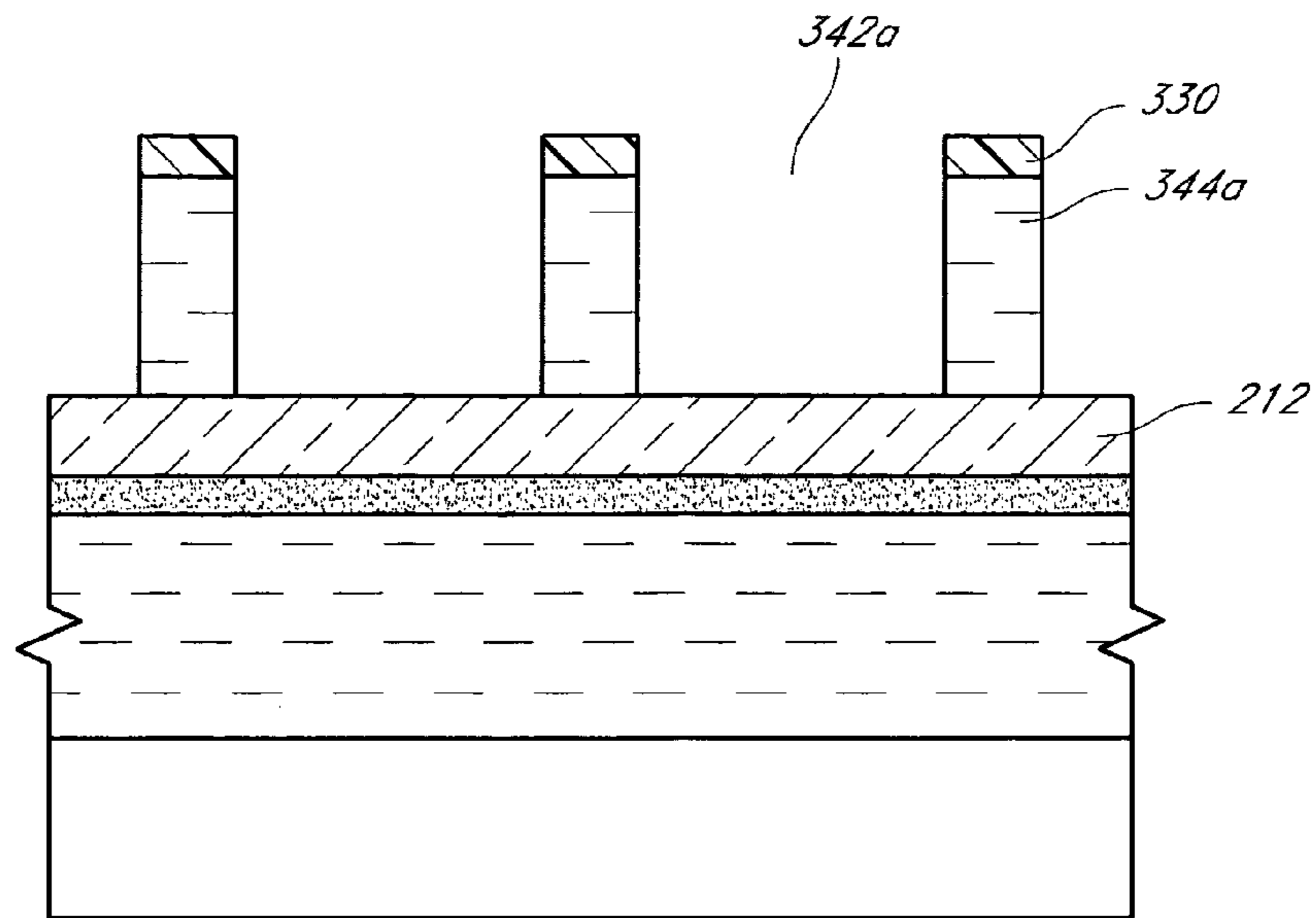
FIG. 15C
