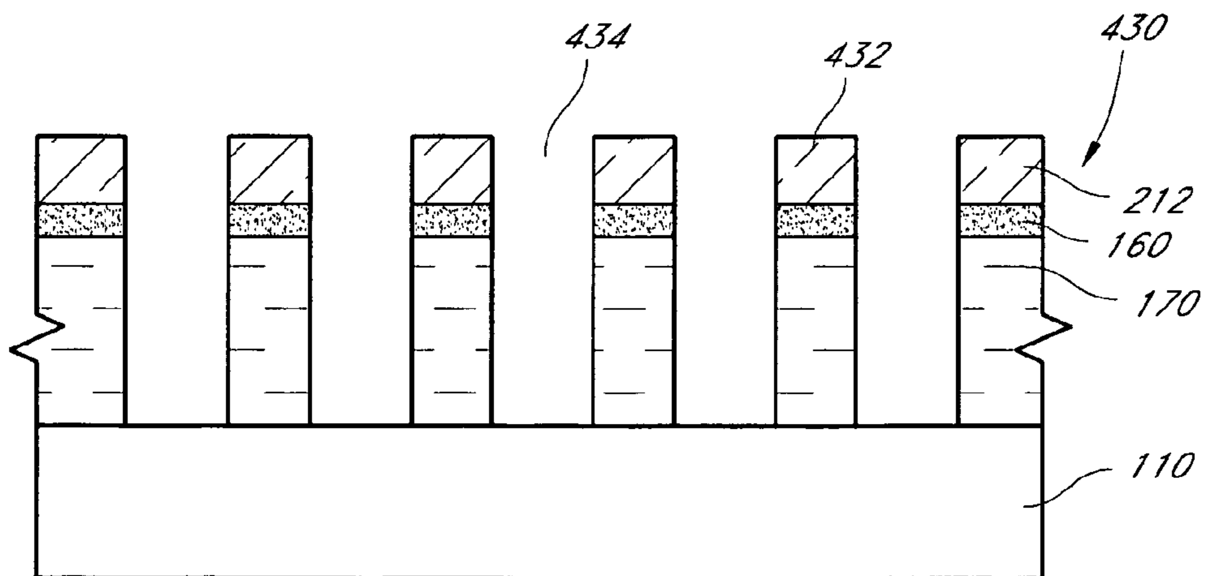
FIG. 24B
