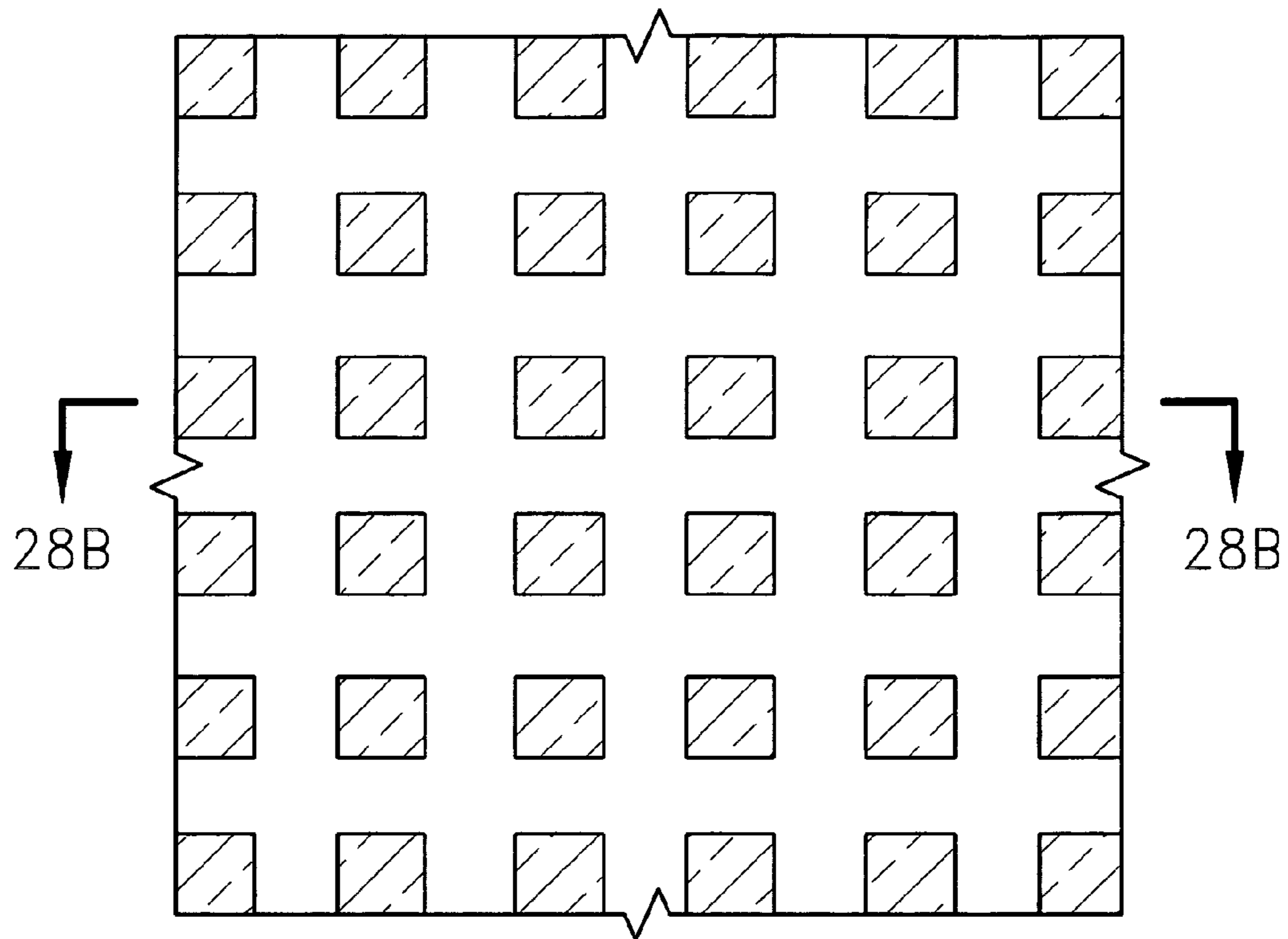
FIG. 28A
