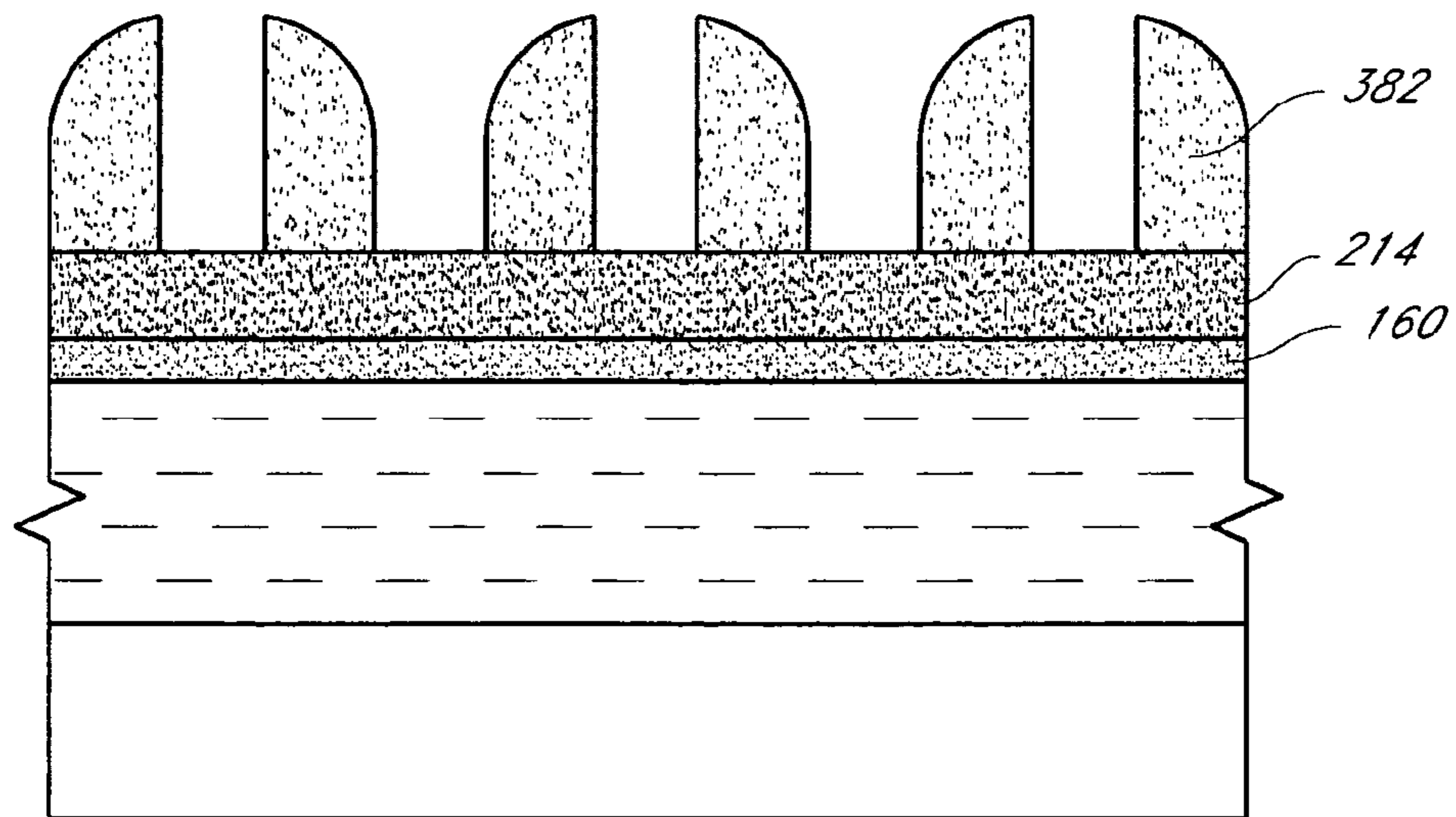
FIG. 22D
