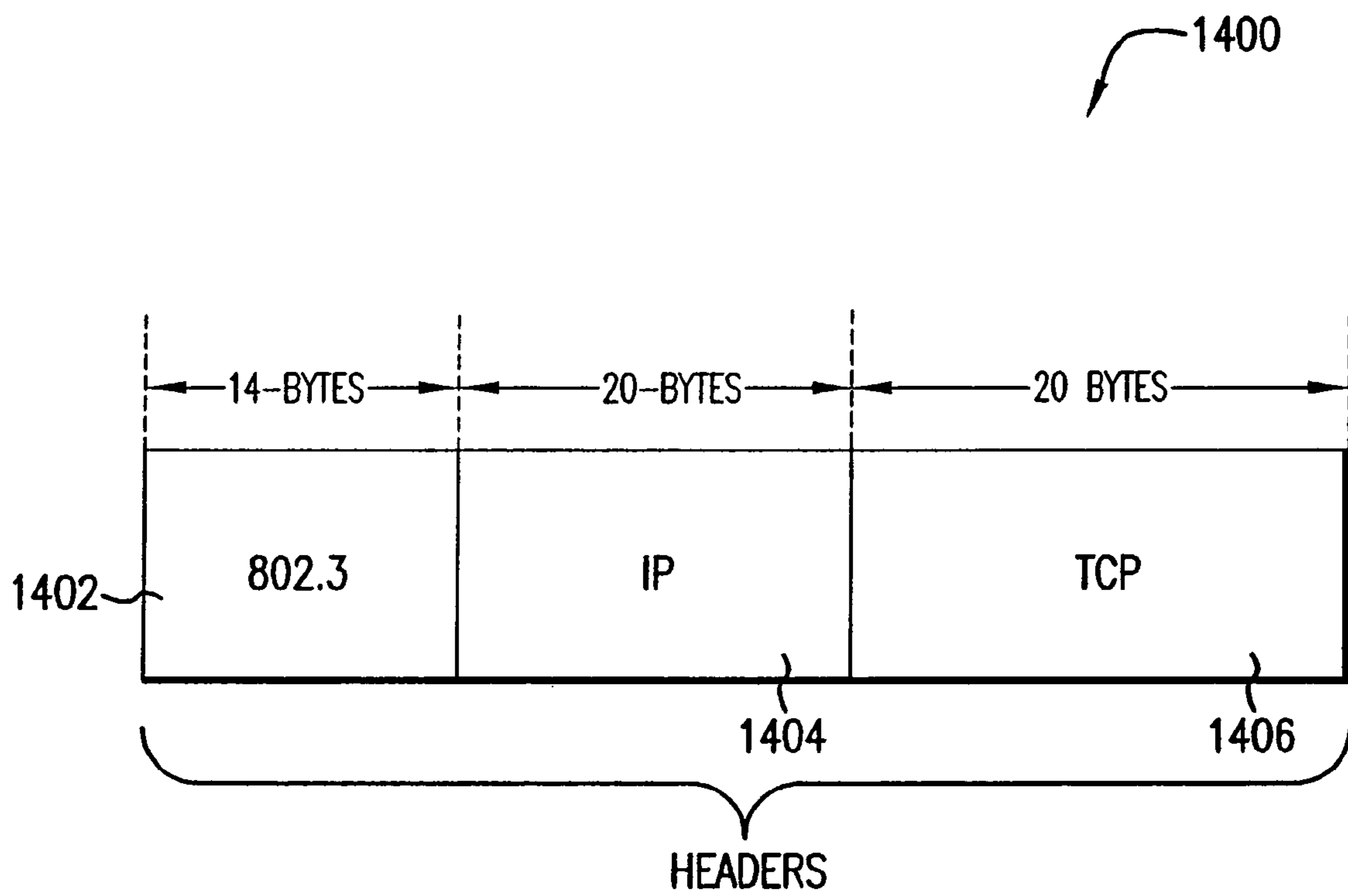
FIG. 14A
