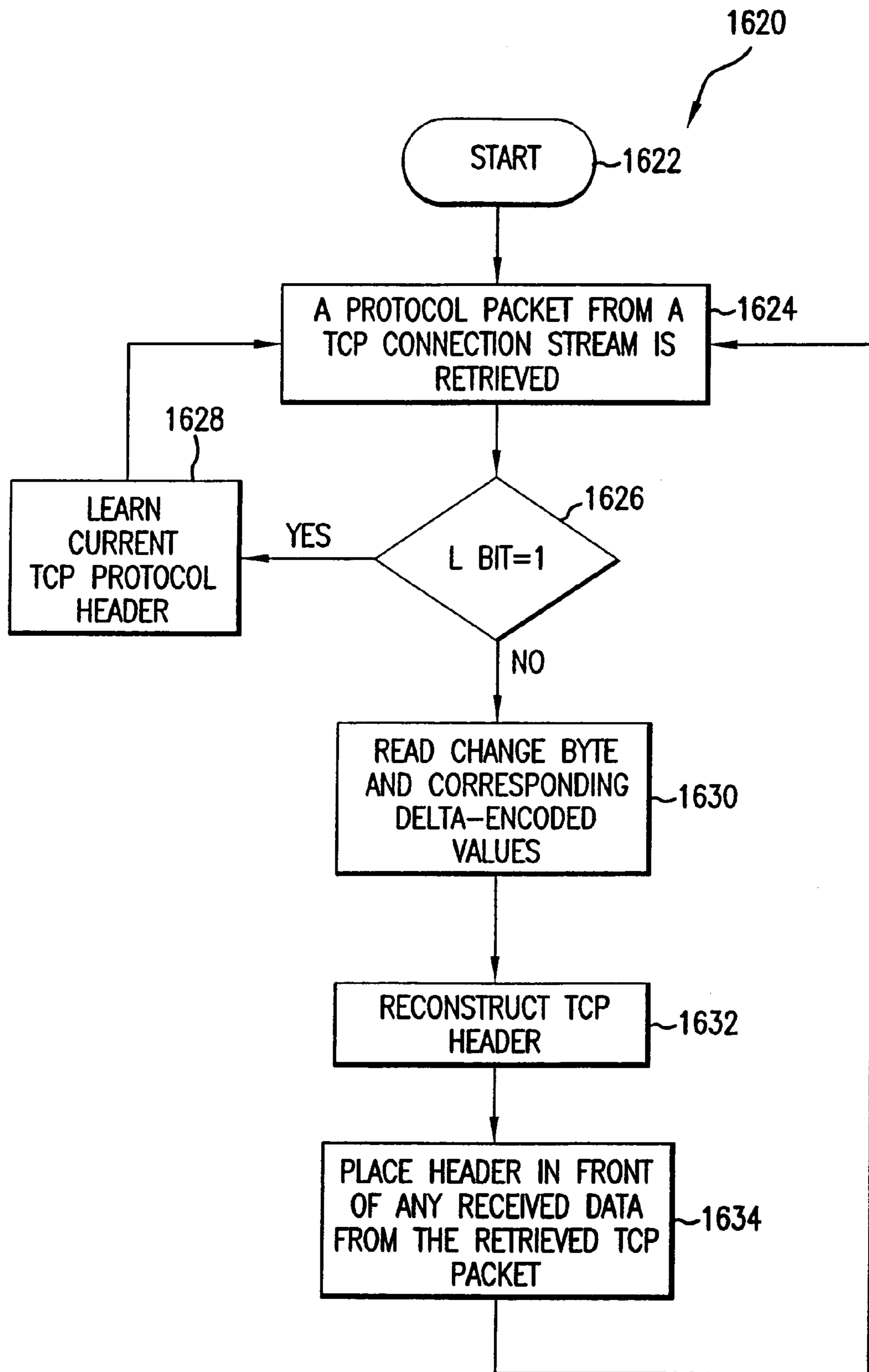
FIG. 16B
