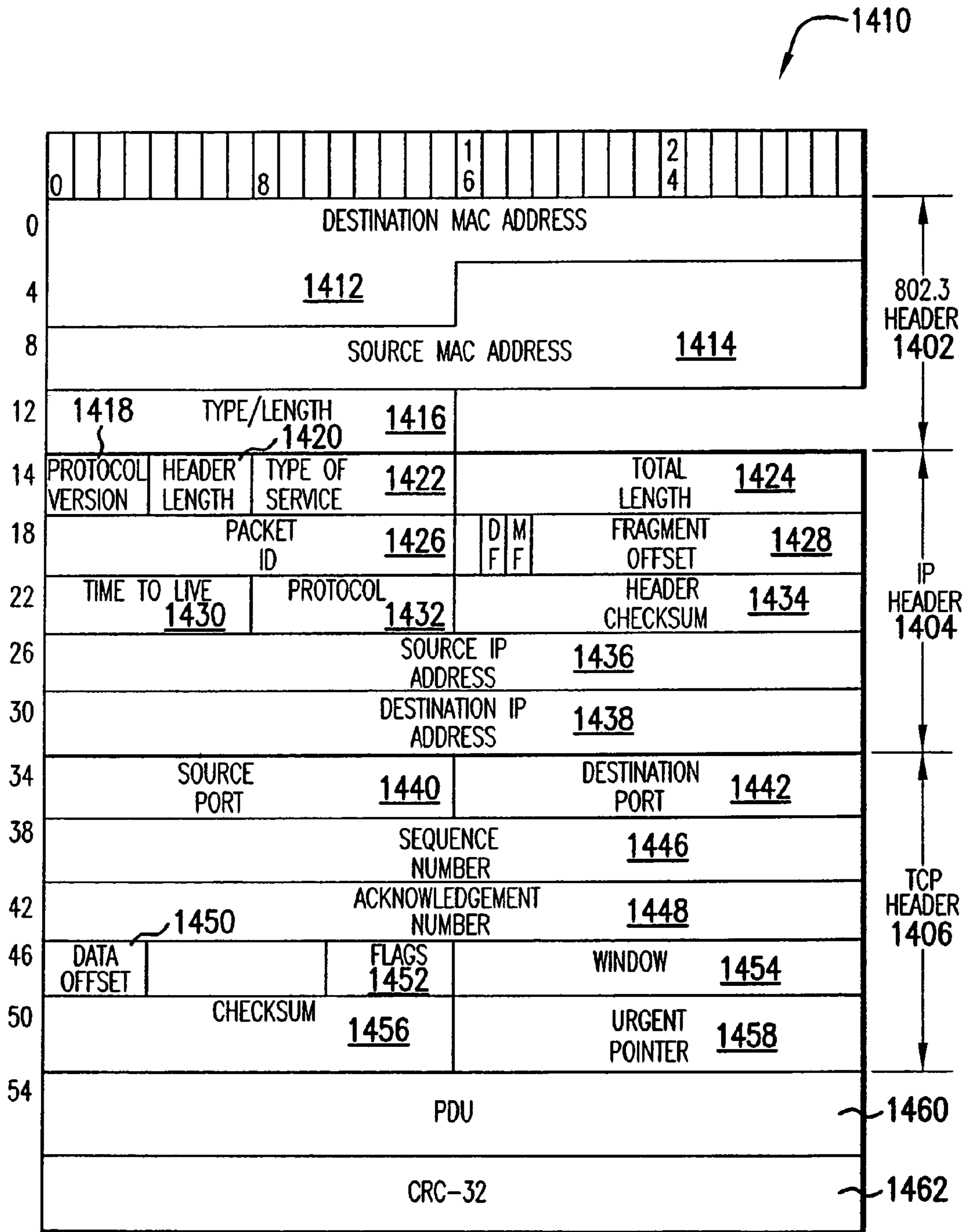
FIG.14B
