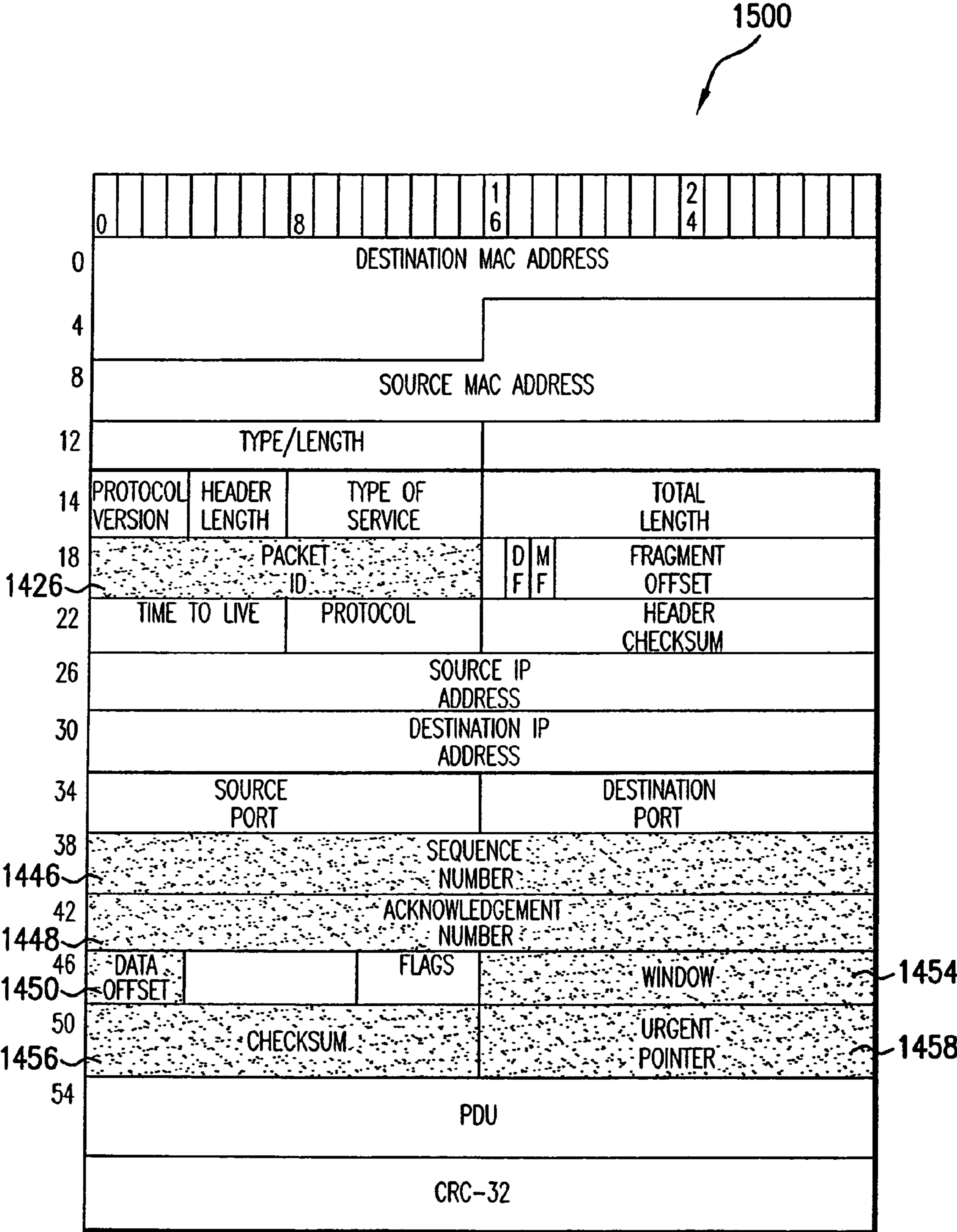
FIG.15
