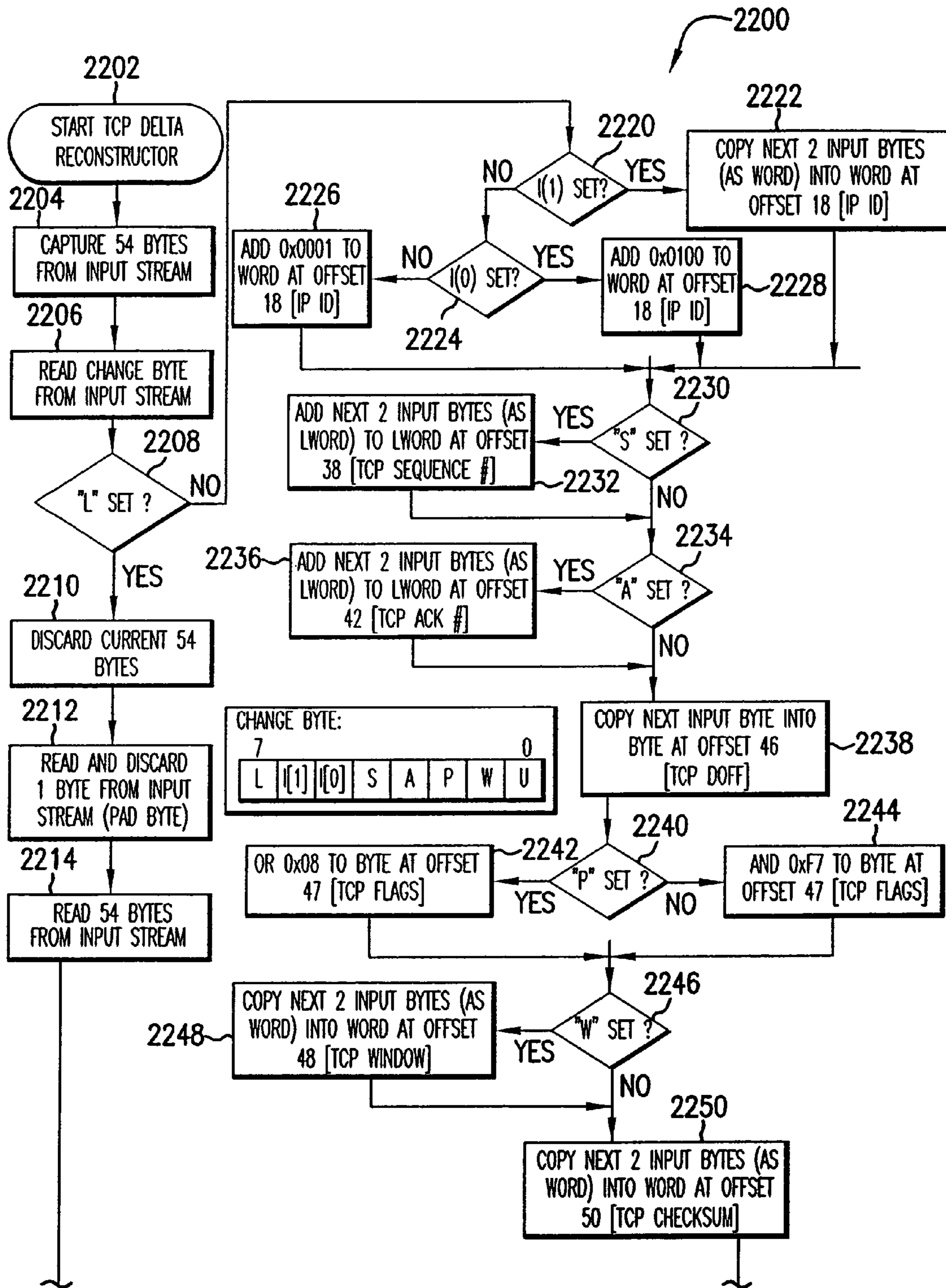
FIG.22A
