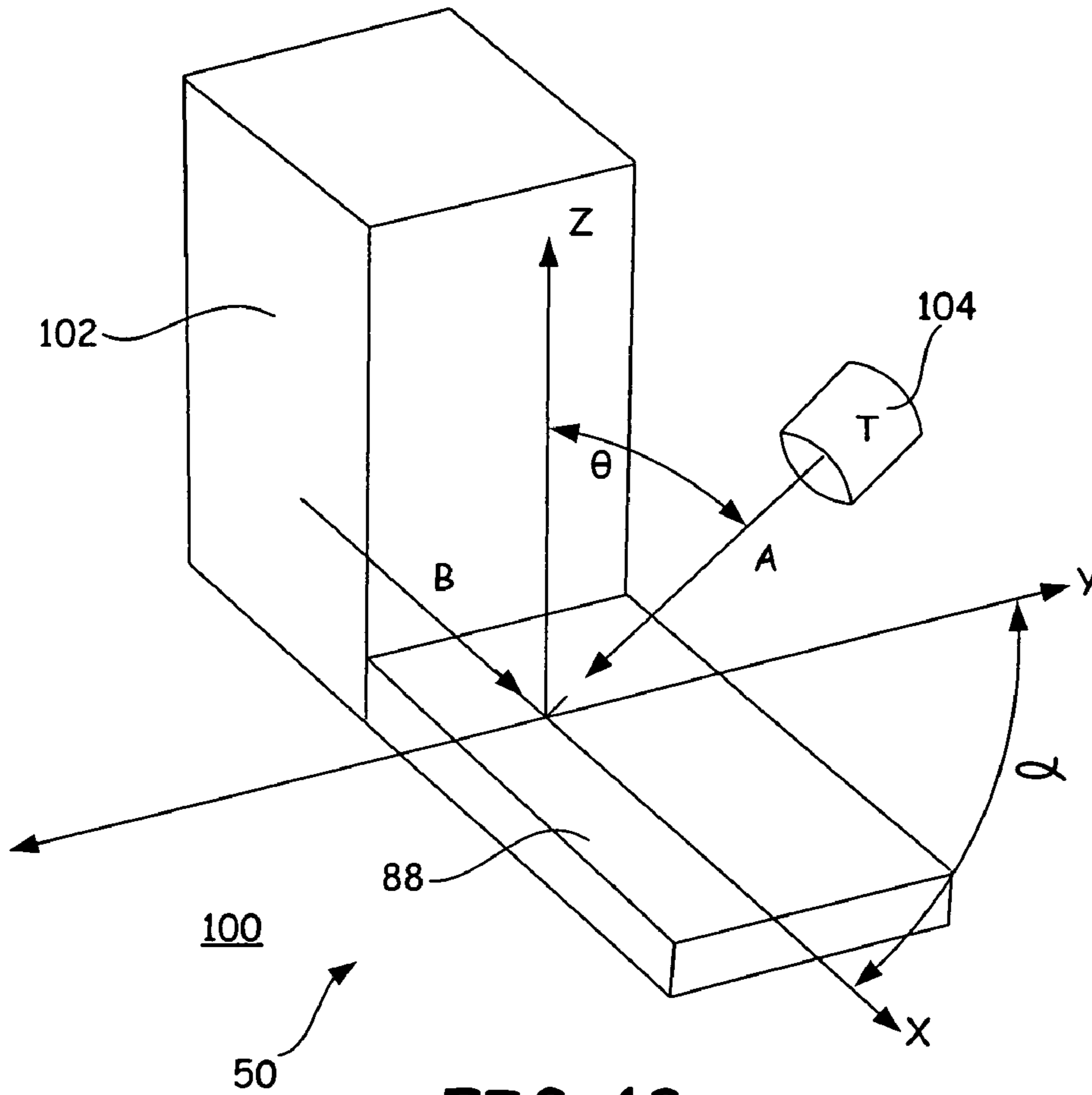
FIG. 13
