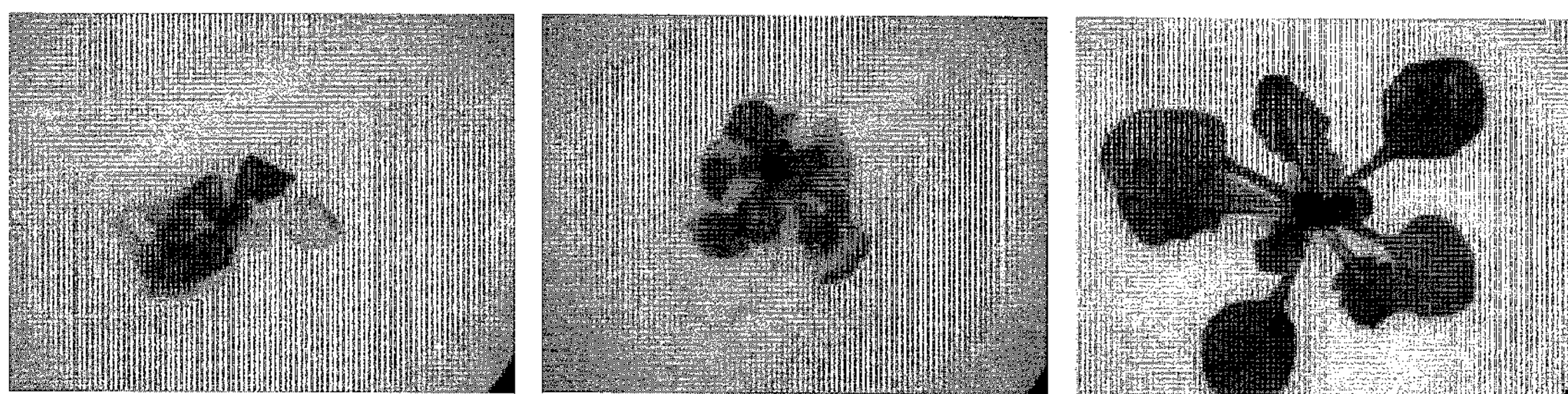
PpMYB-1
