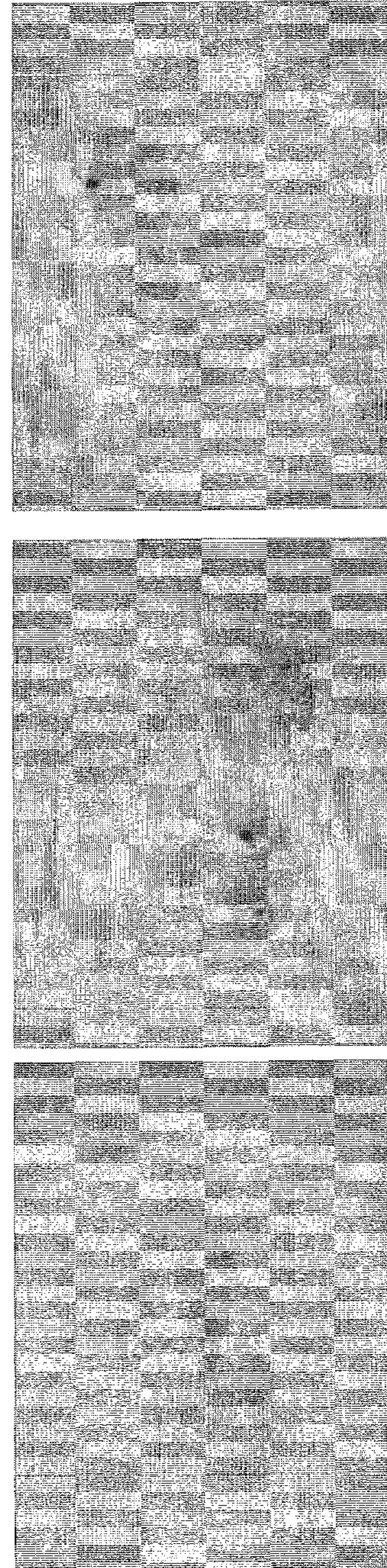
Wild Type
