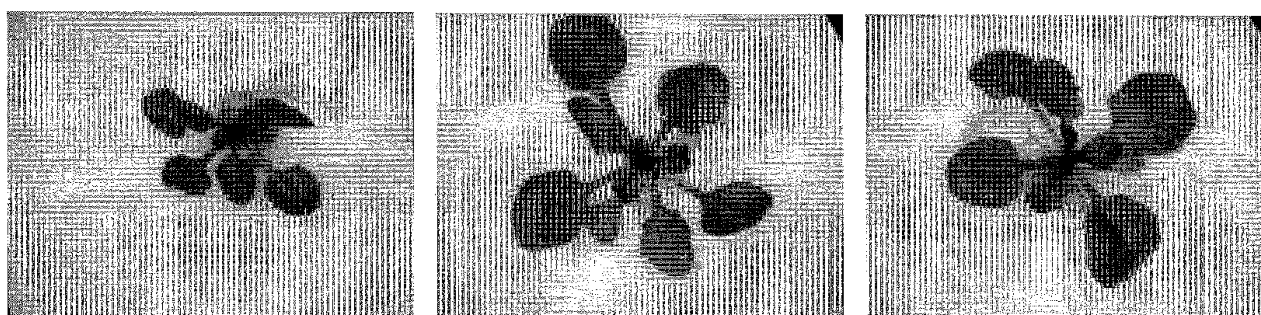
PpCABF-3
