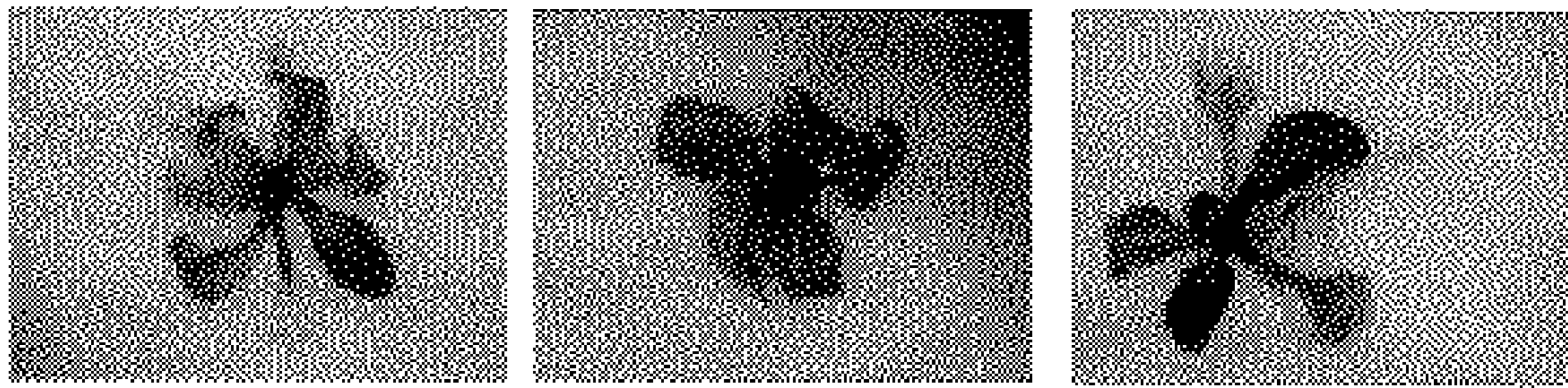
PpZF-3
