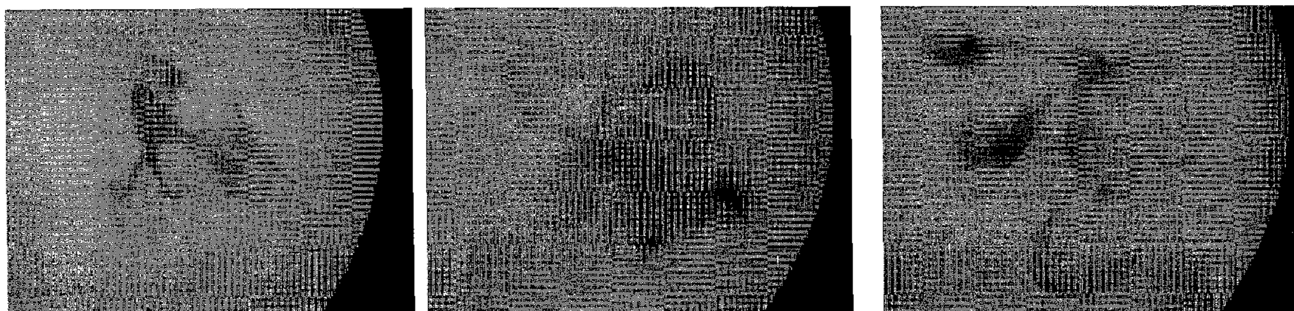
Wild Type
