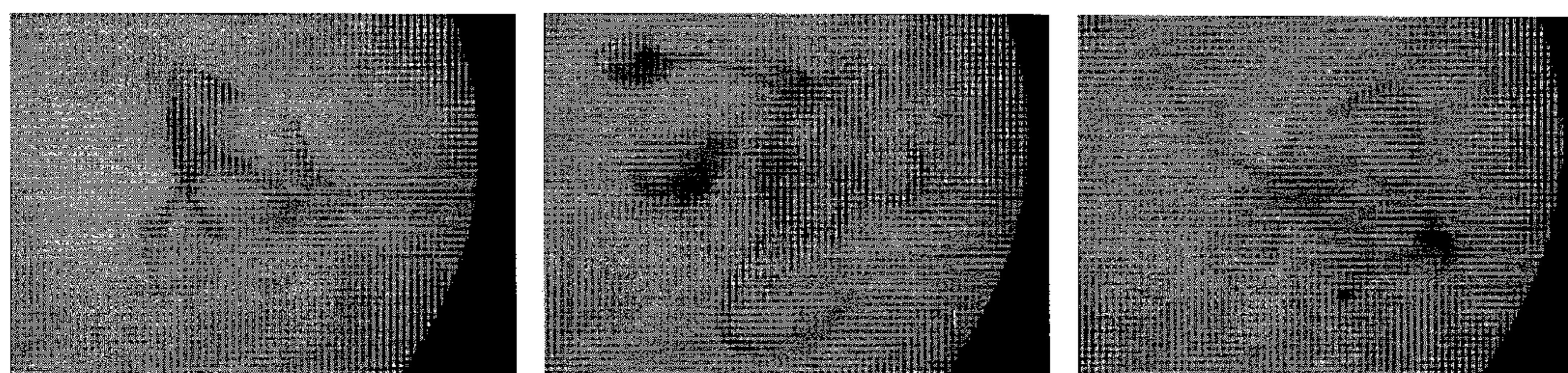
Wild Type
