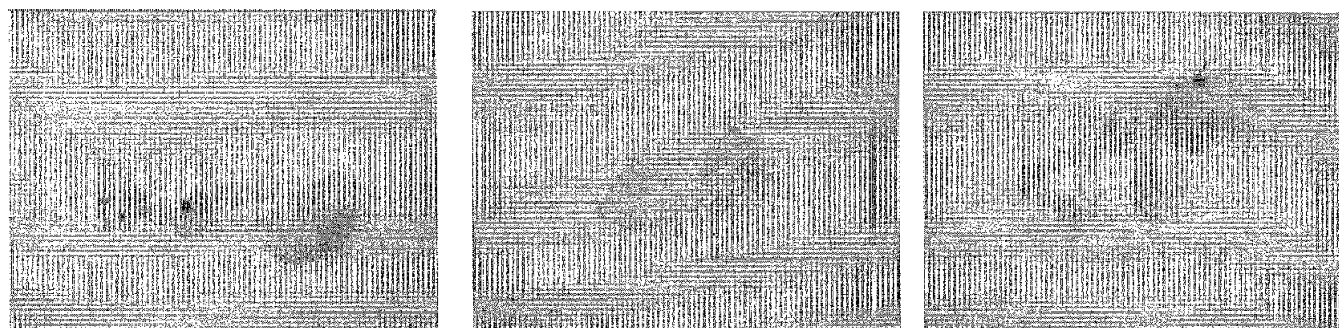
Wild Type
