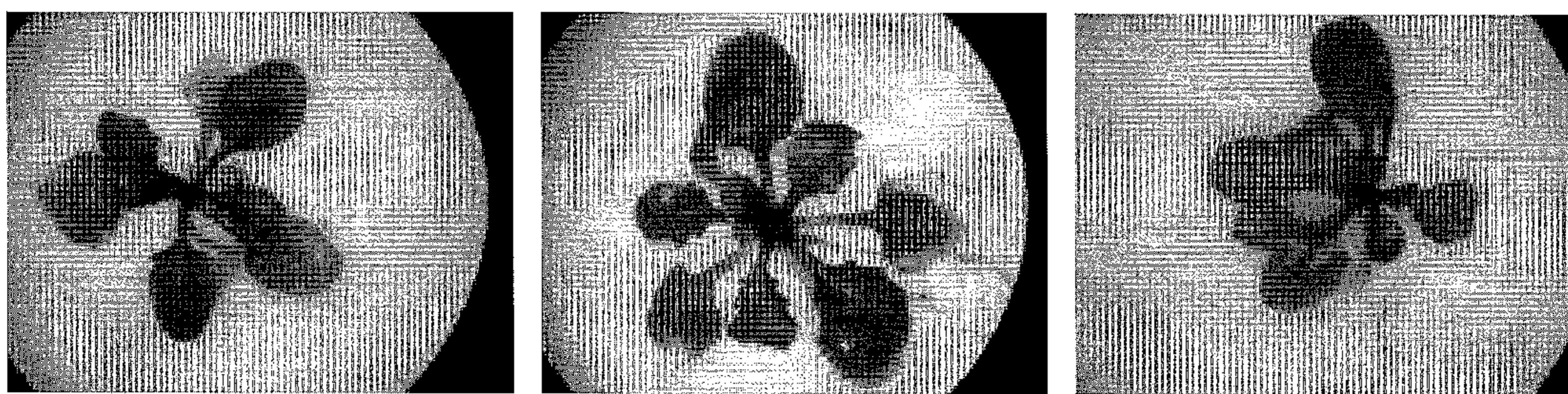
PpSFL-1
