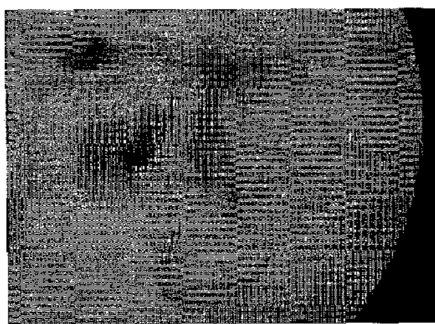
Wild Type
