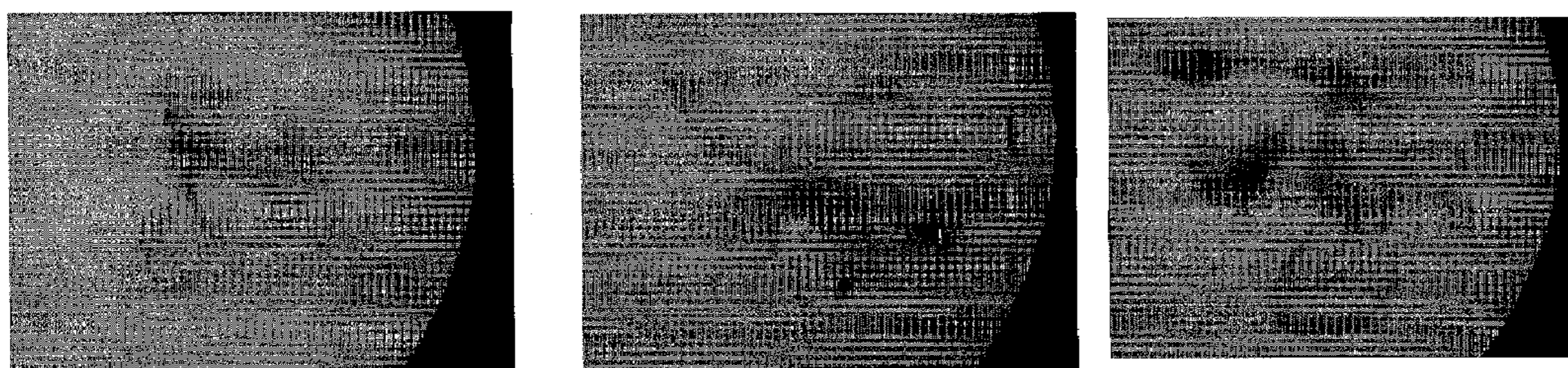
Wild Type
