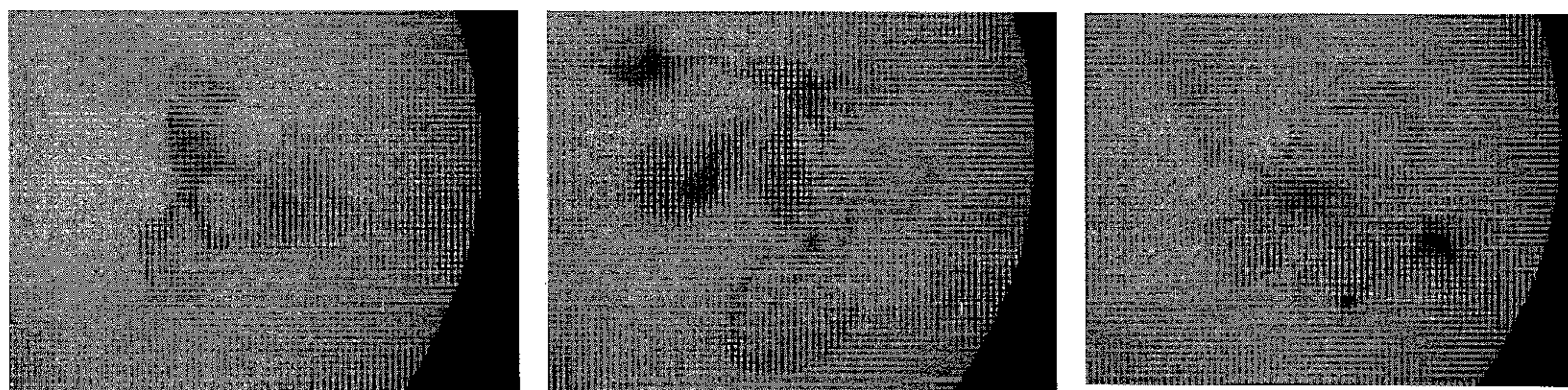
Wild Type
