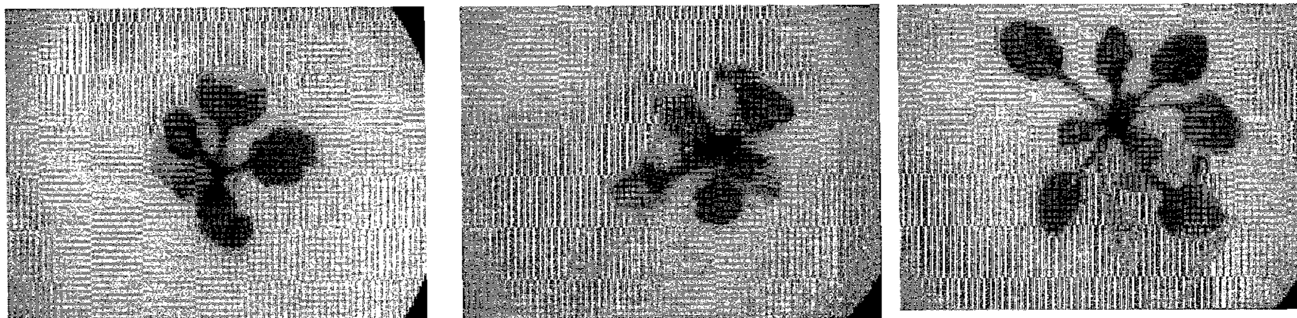
PpAPS-2
