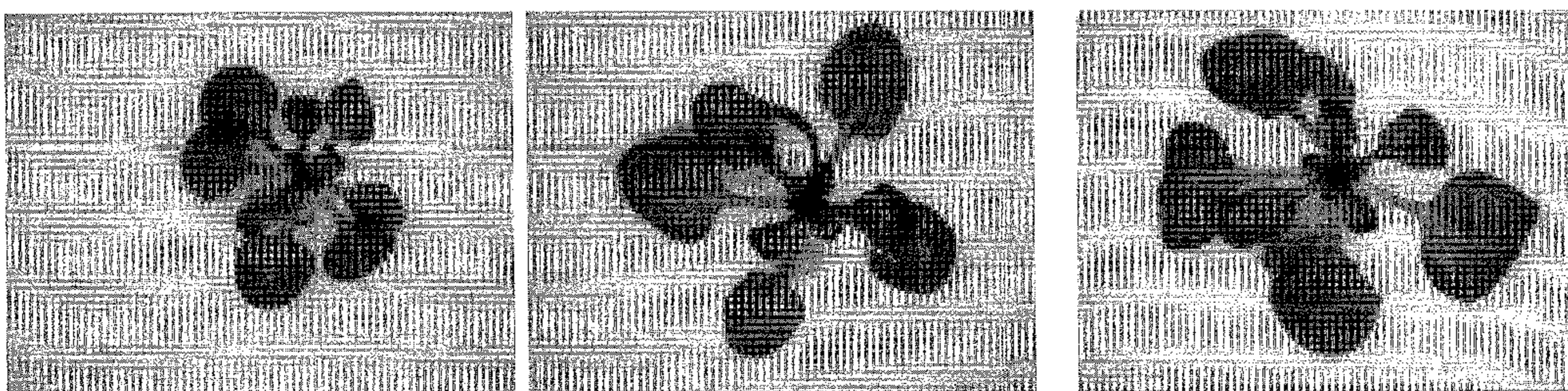
PpZF-3
