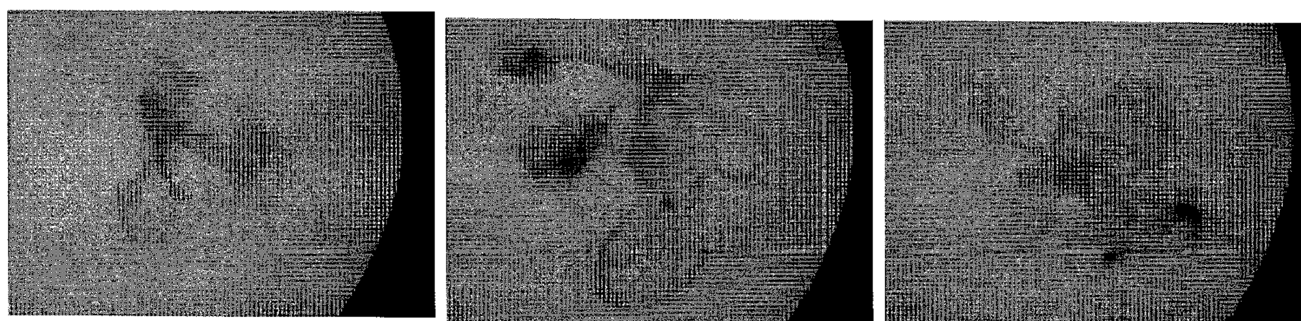
Wild Type
