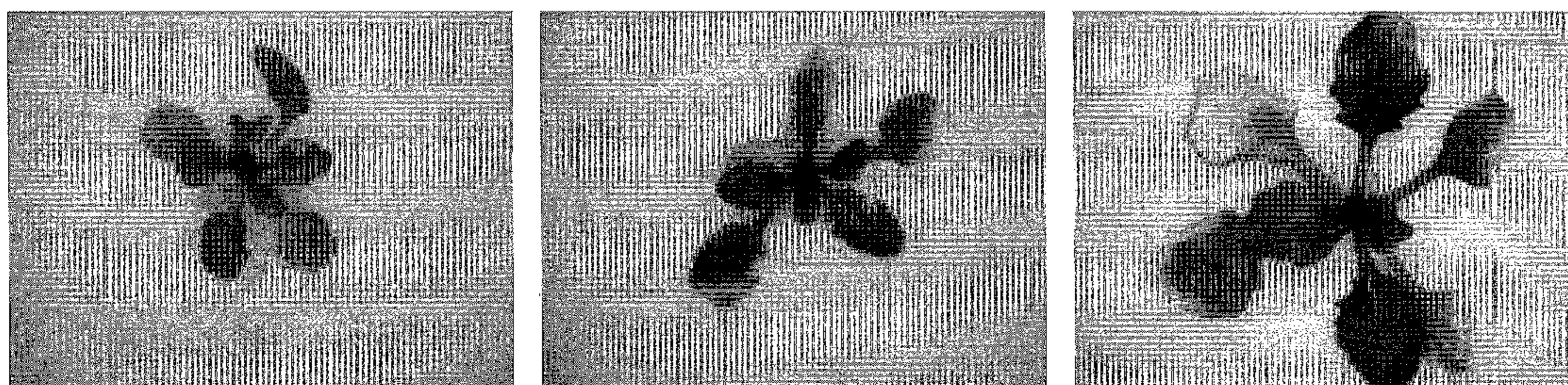
PpZF-5
