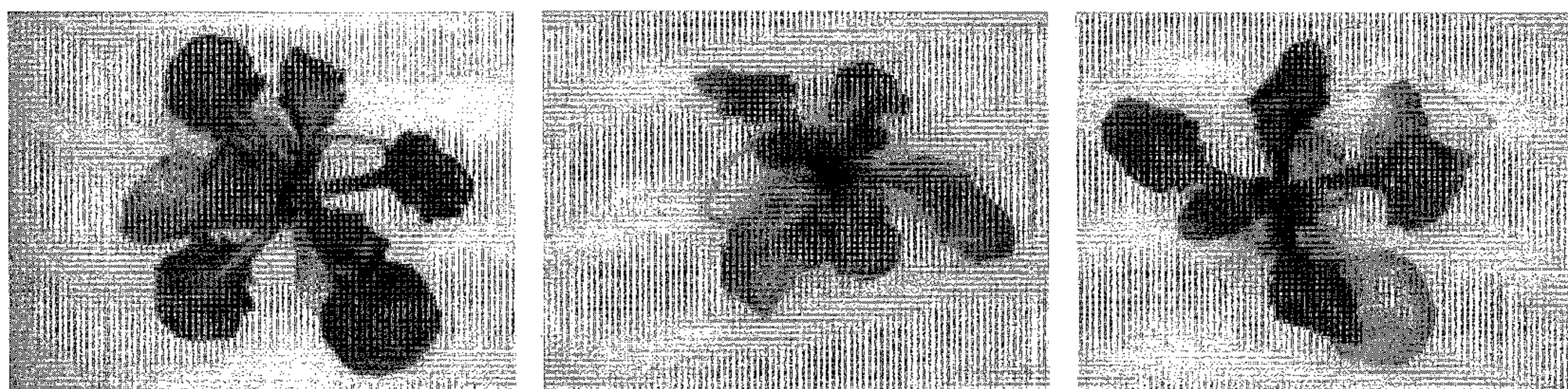
PpCABF-3
