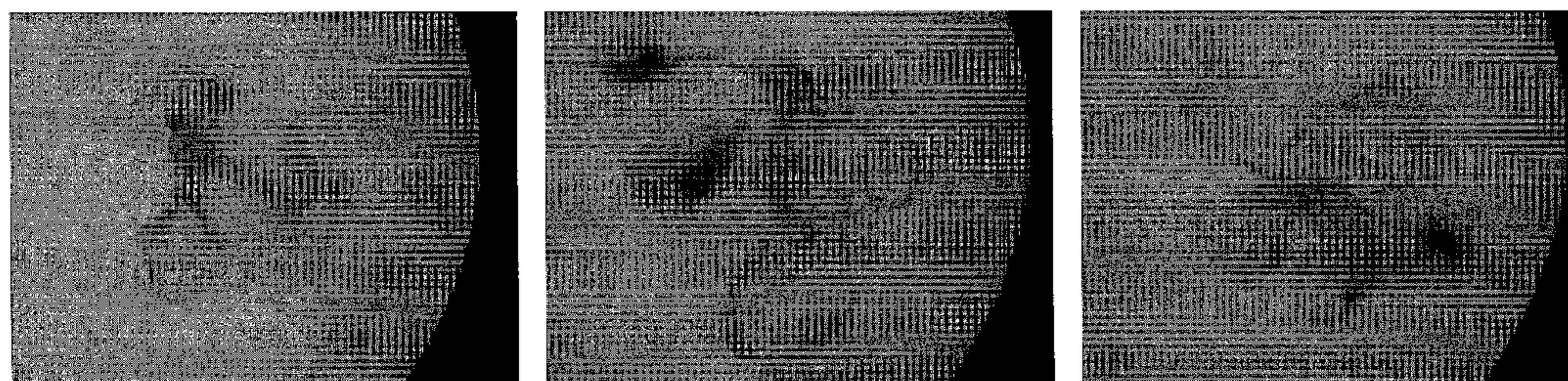
Wild Type
