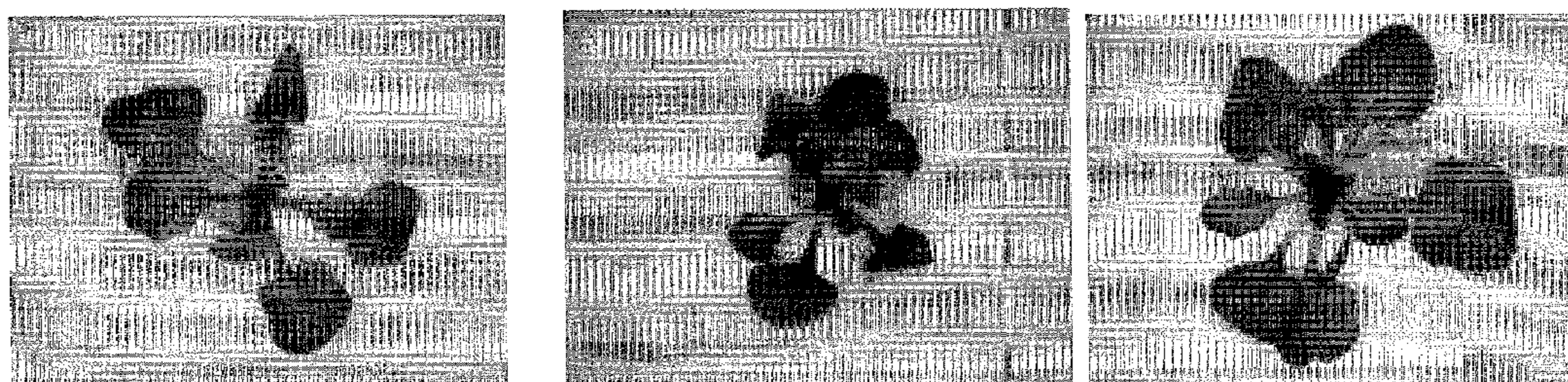
PpZF-2
