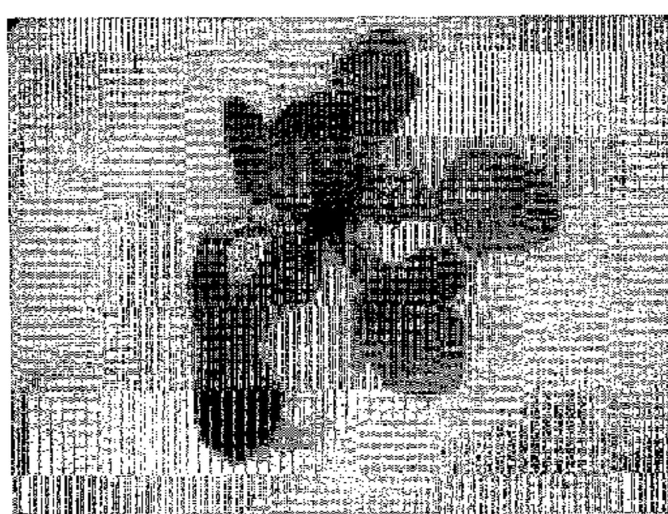
PpZF-4
