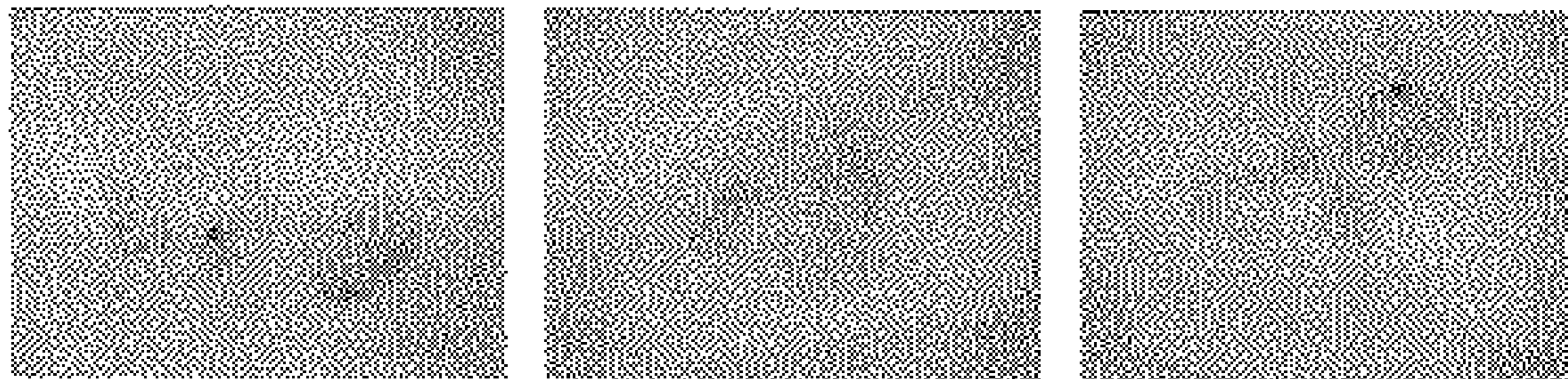
Wild Type
