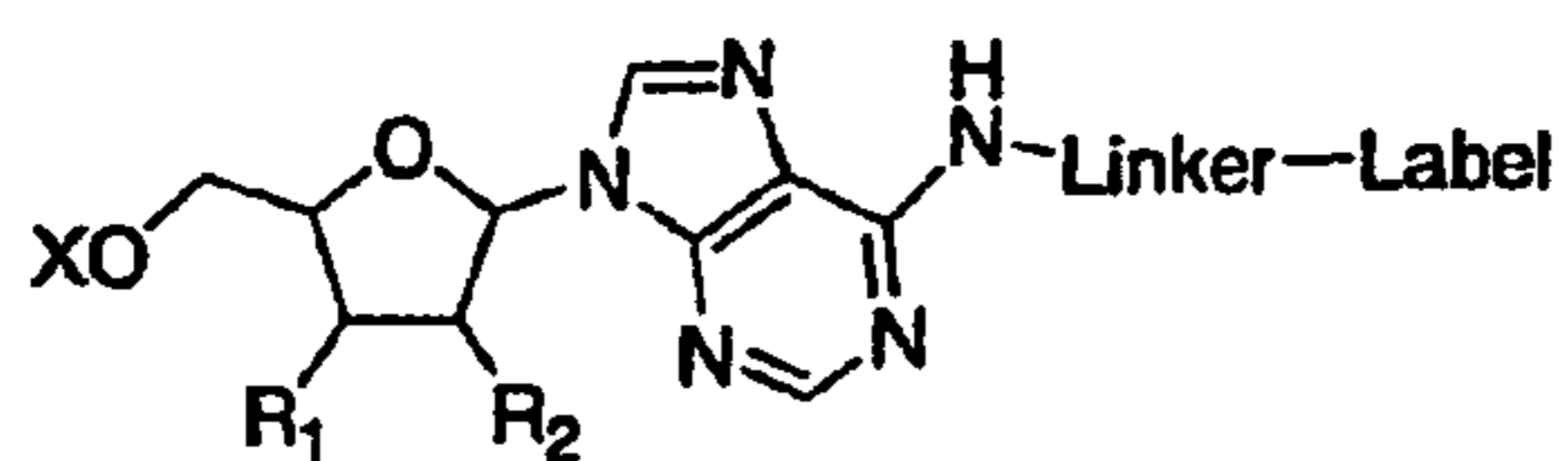
Adenosine N6-linker
