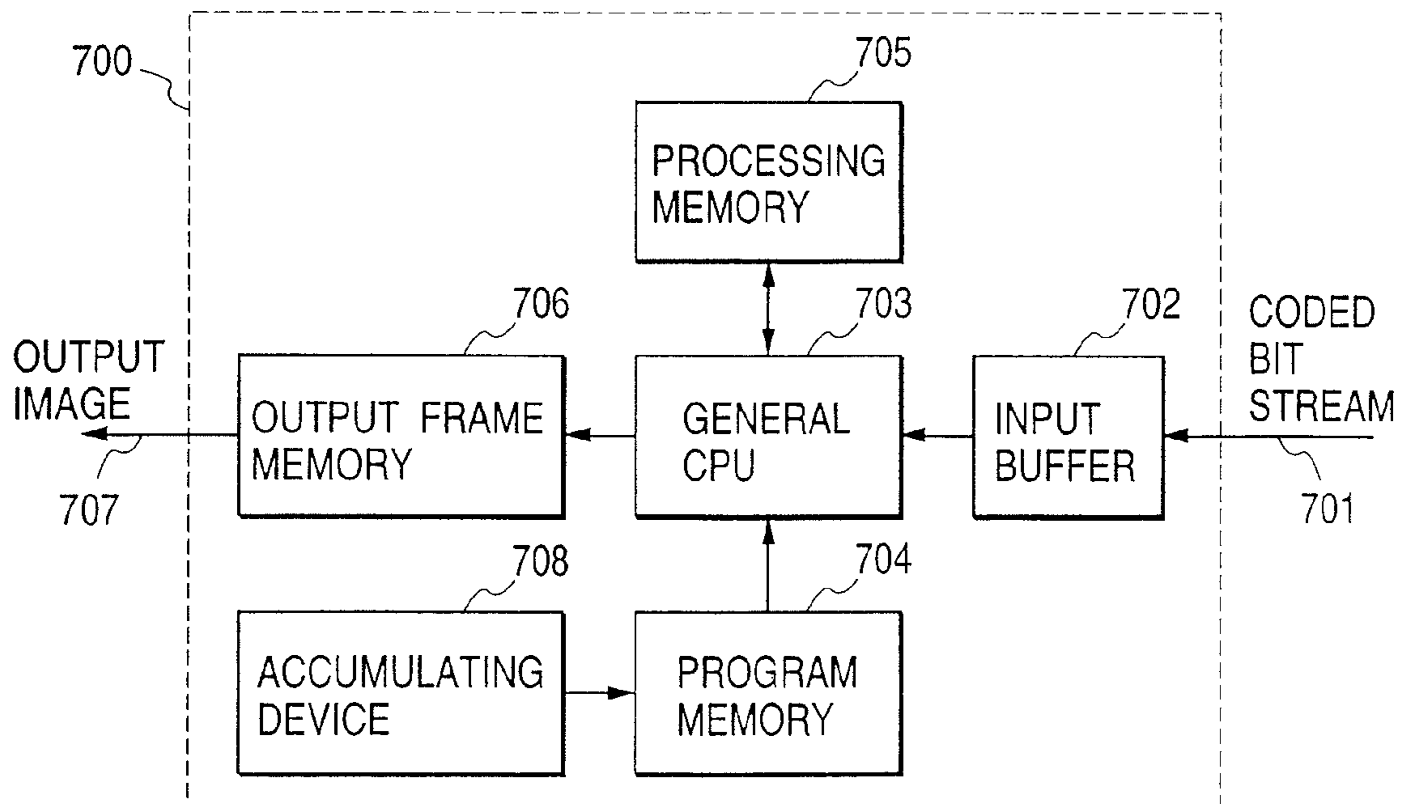
FIG. 7
