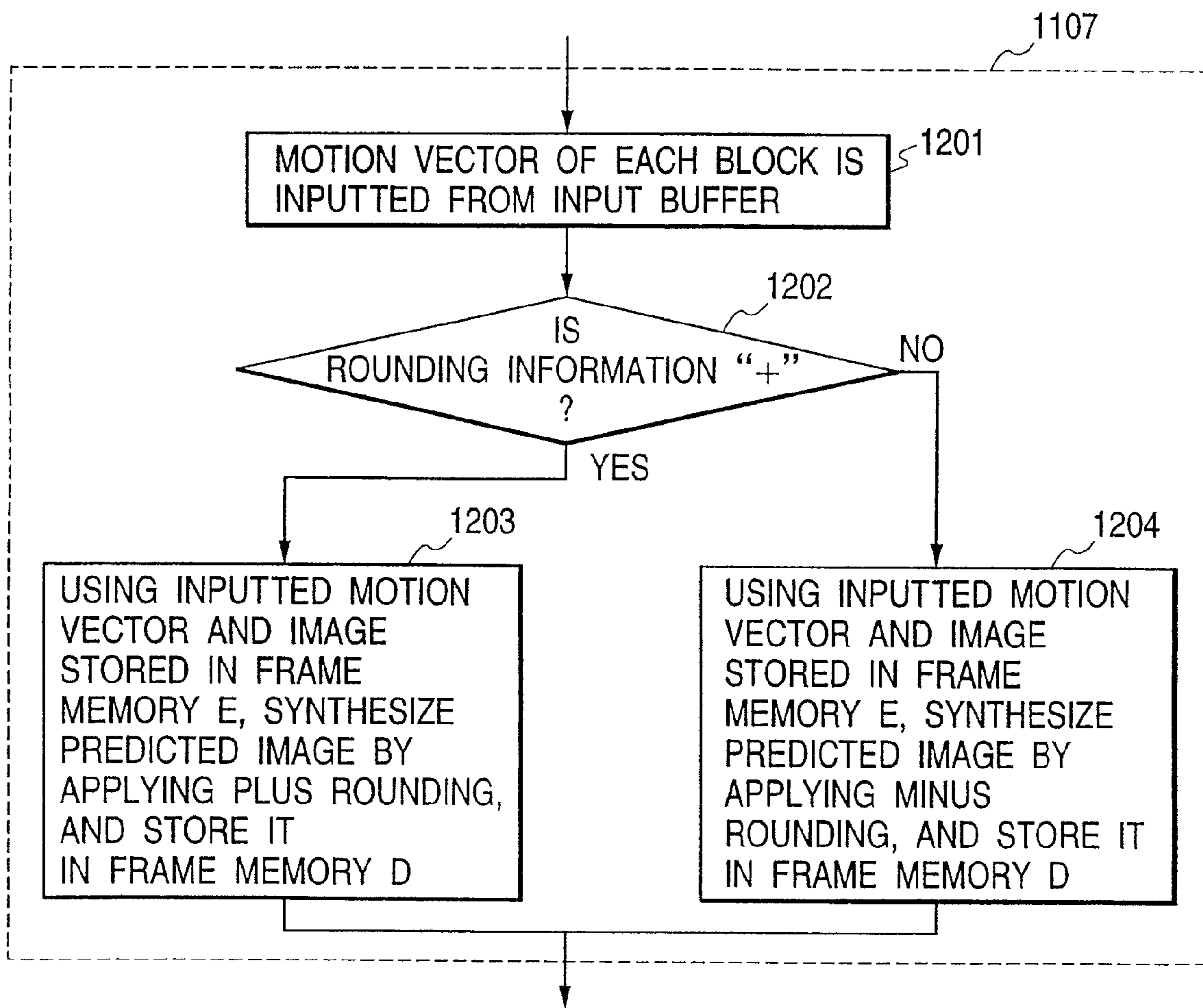
FIG. 12
