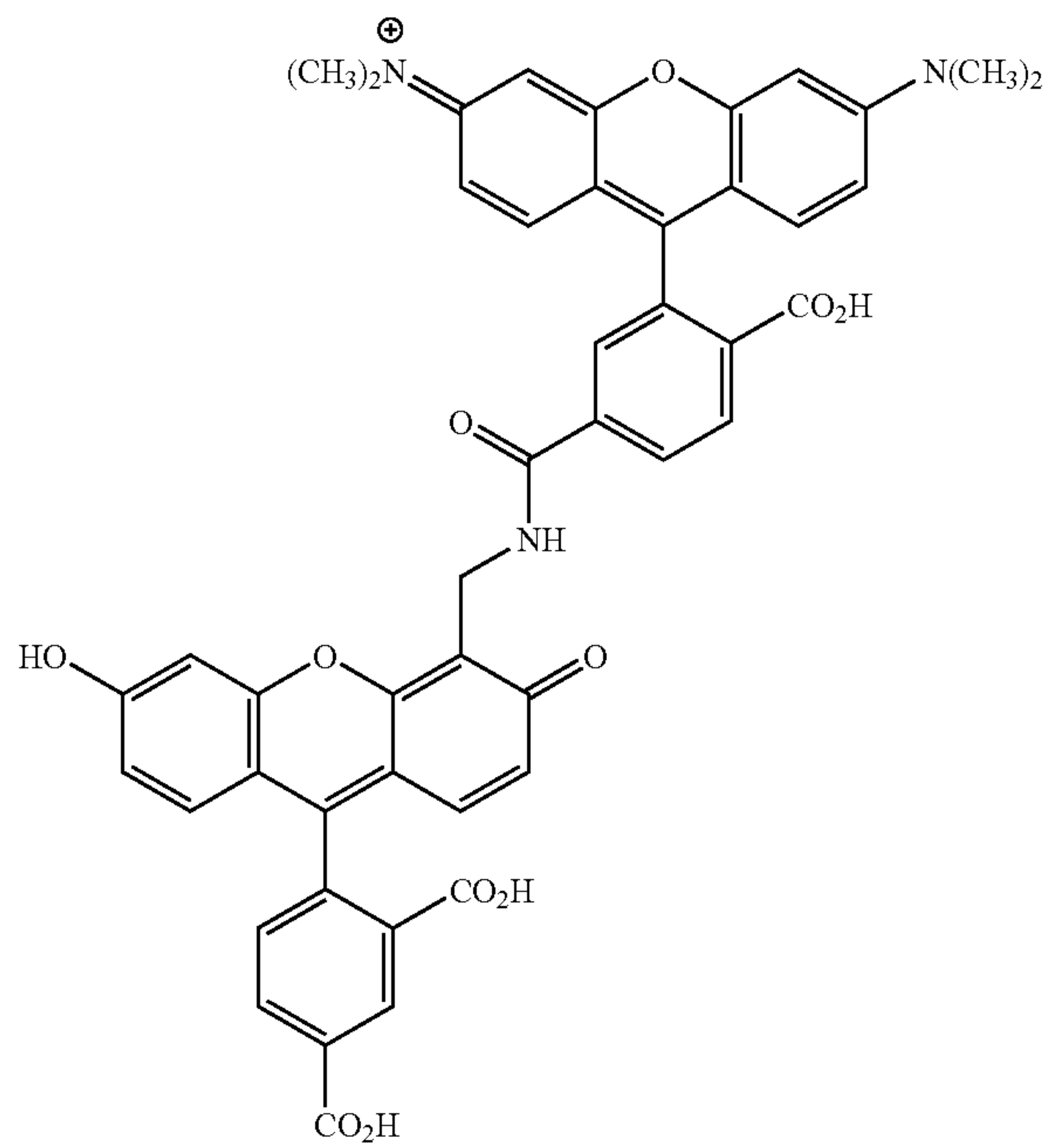
6TMR-CF
