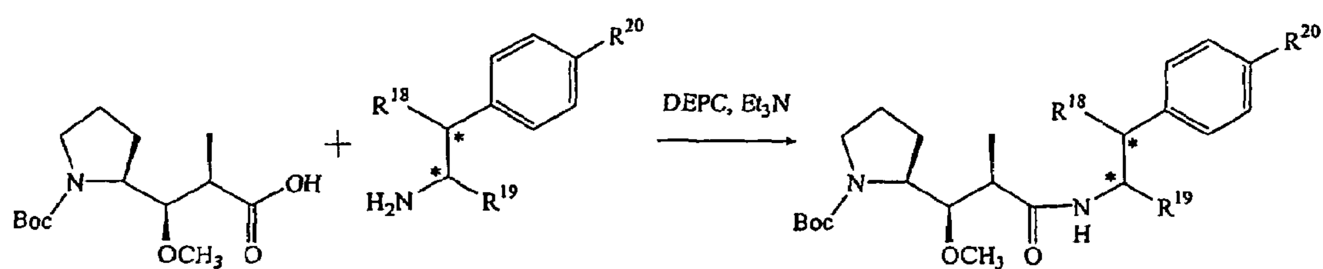
t -Boc Dolaprine (20)
