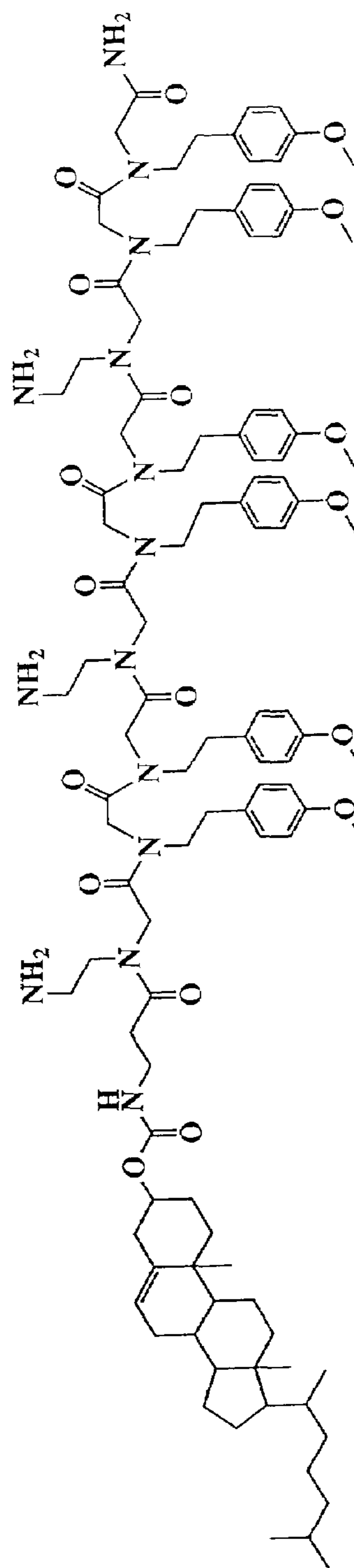
Chol-β-ala-(NaeNmpeNmpe) 3
