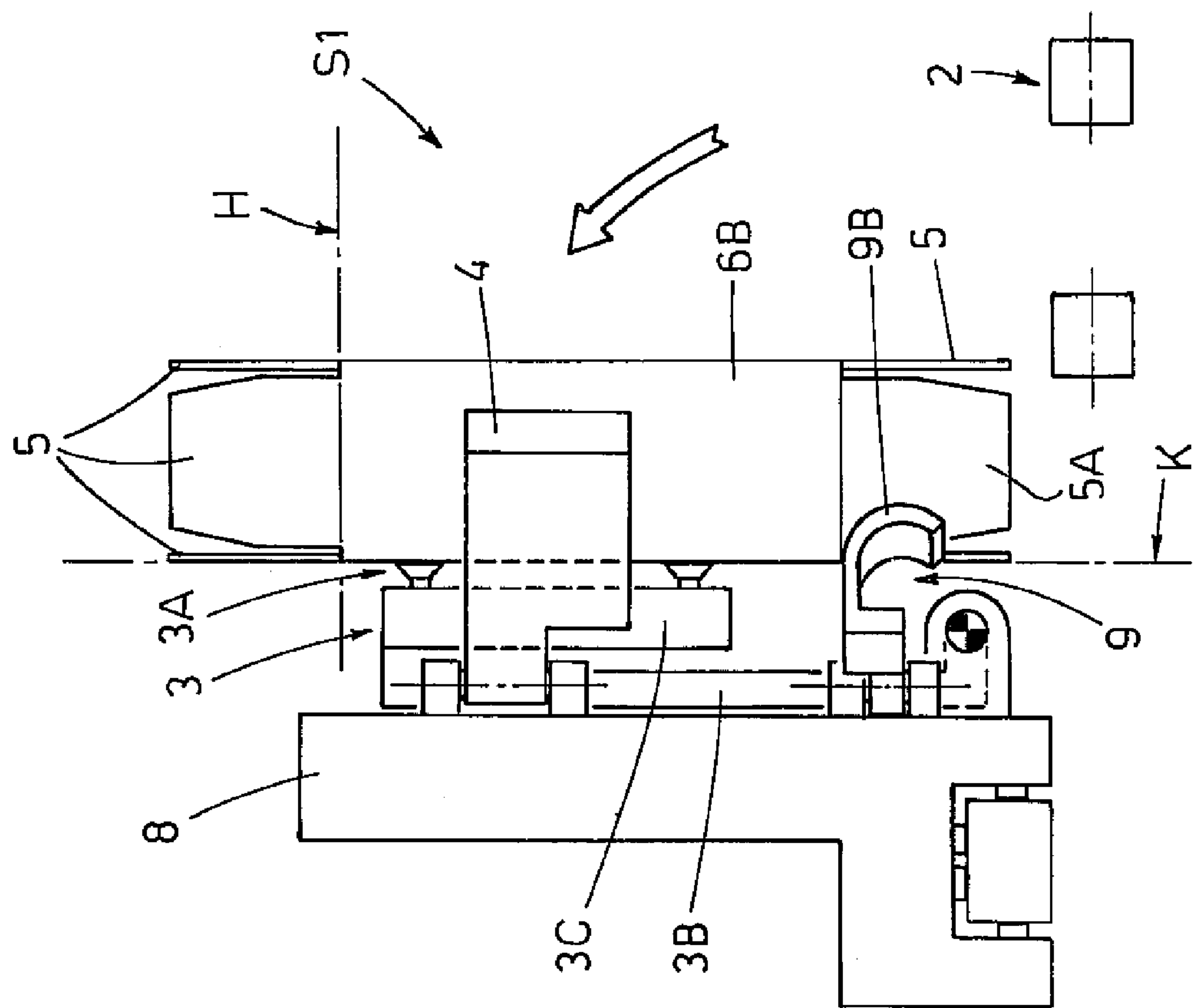
FIG. 4A
