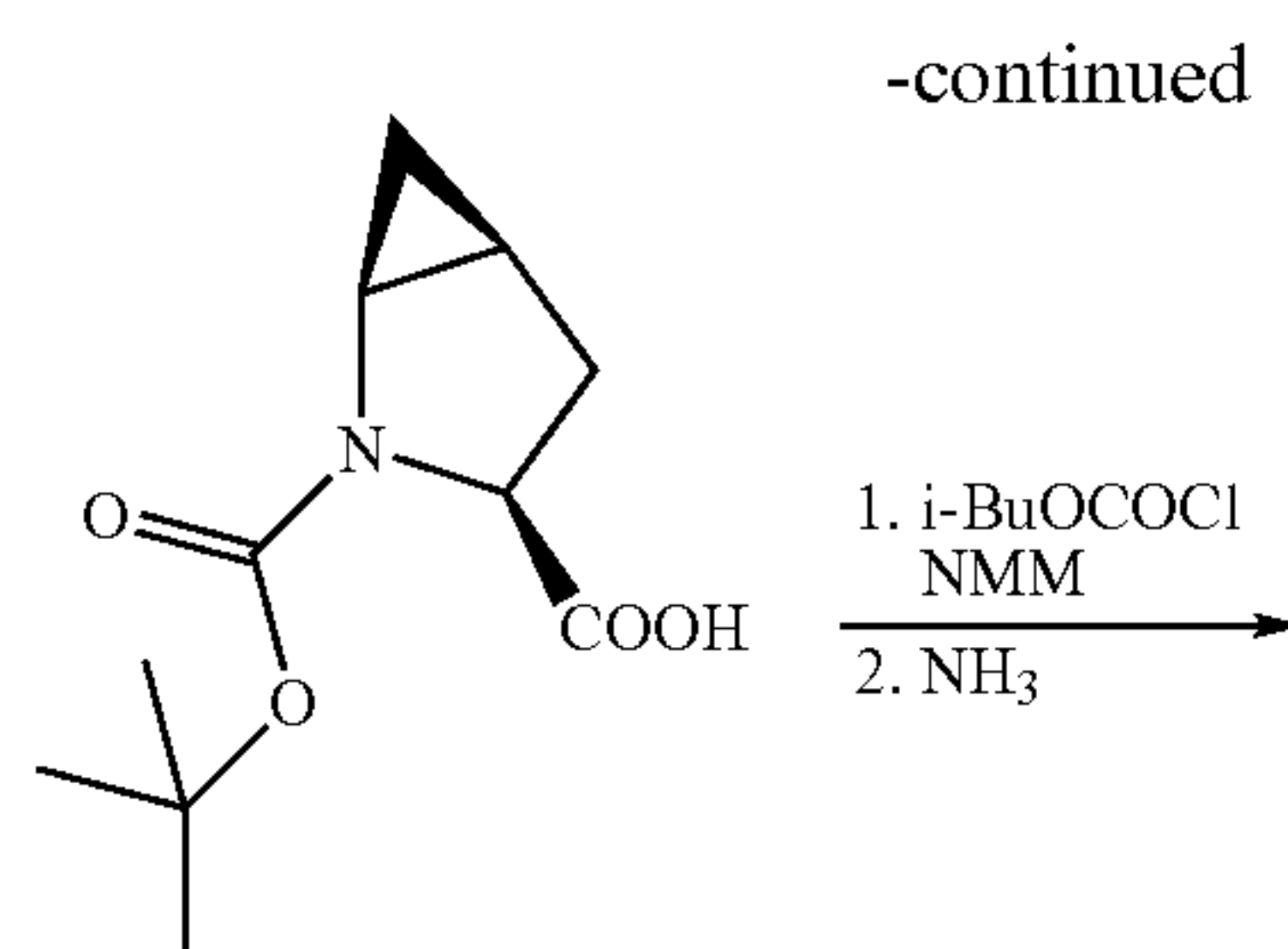
XVIII s-BOC-MP C 11 H 17 NO 4 Mol. Wt.: 227.26
